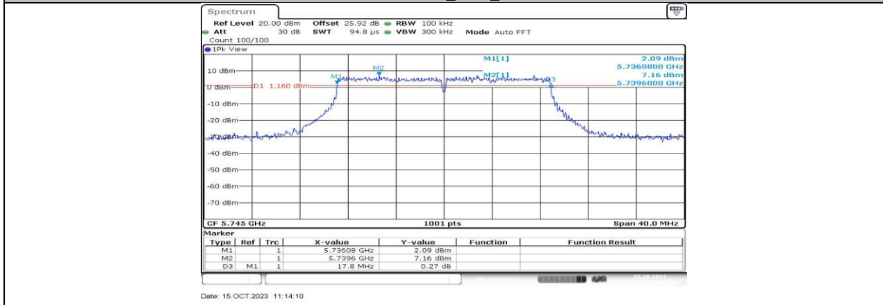
11N20MIMO_Ant4_5745
