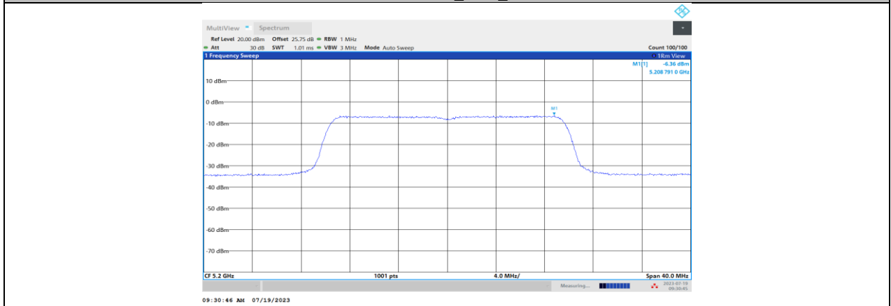
11BE20MIMO_Ant3_5200
