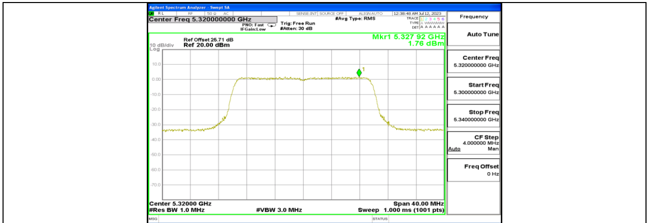
11BE20MIMO_Ant3_5320
