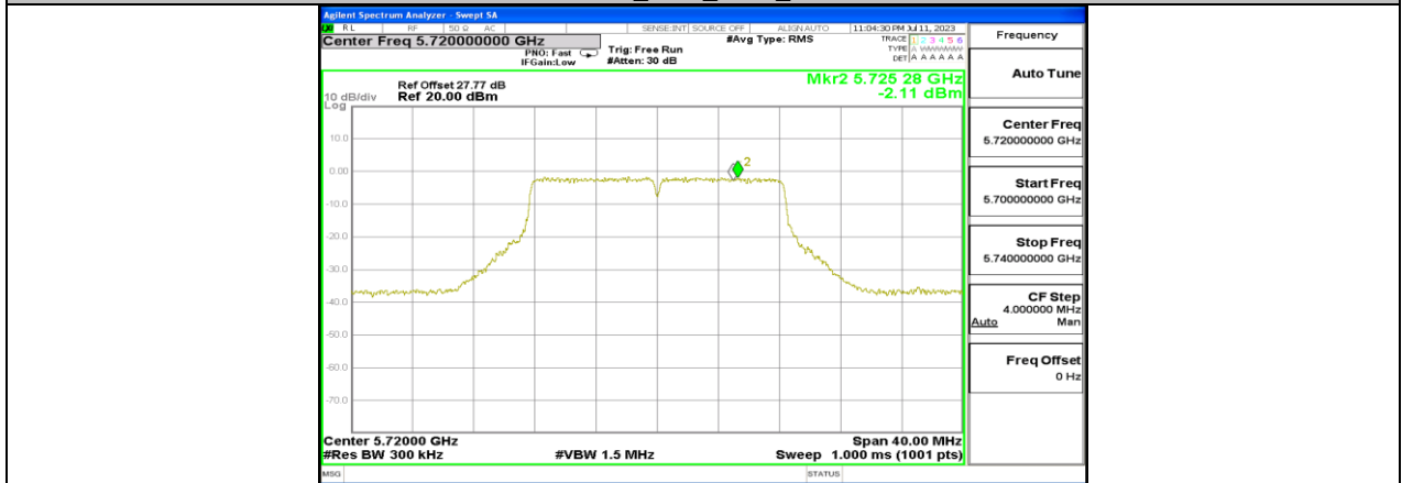
11A-CDD_Ant1_5720_UNII-3
