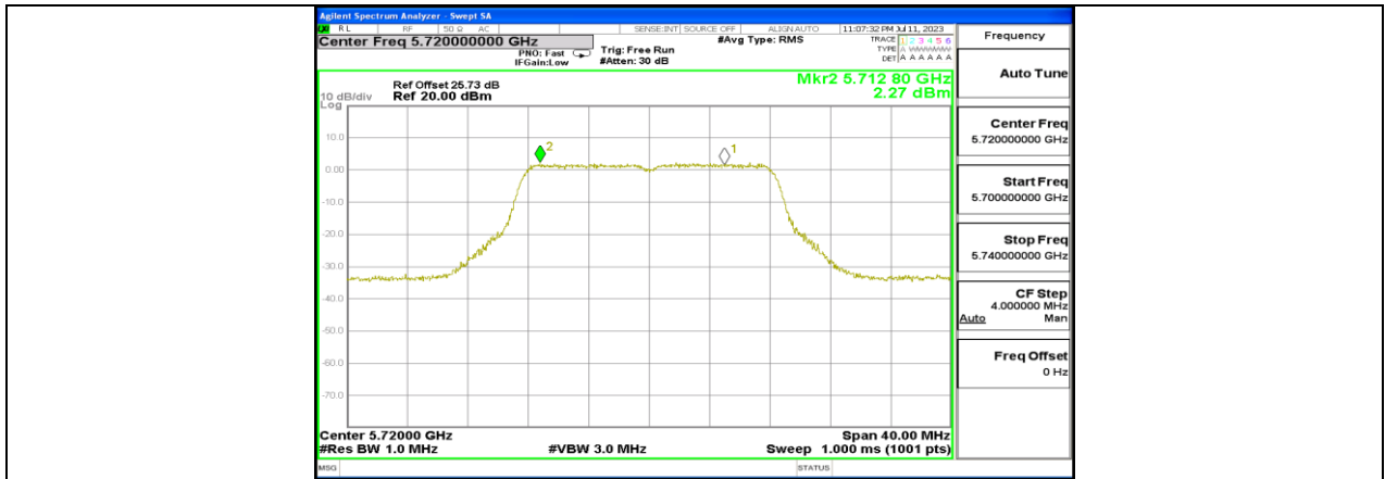
11A-CDD_Ant3_5720_UNII-2C
