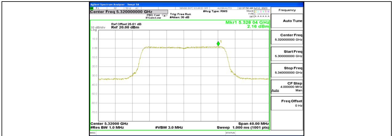
11BE20MIMO_Ant2_5320
