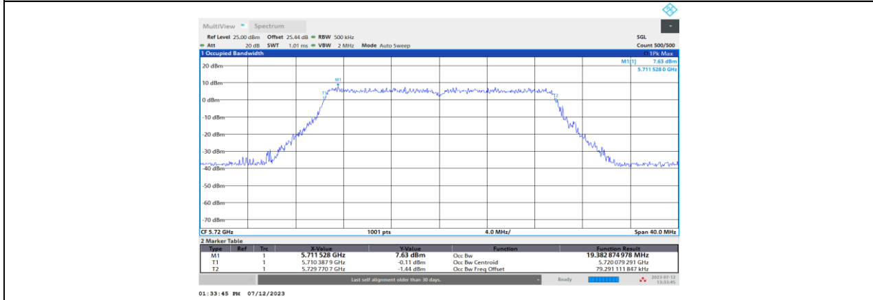
11BE20MIMO_Ant1_5720
