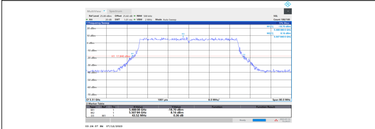
11BE40MIMO_Ant2_5510
