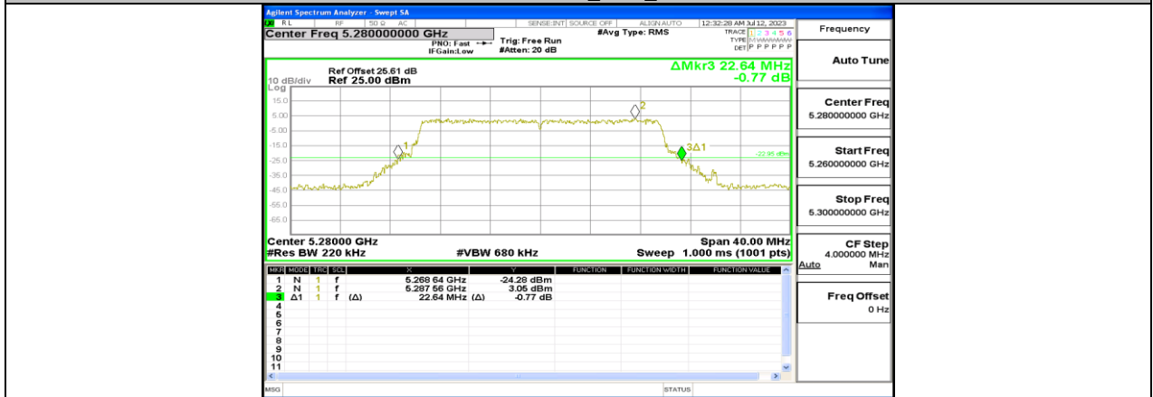
11BE20MIMO_Ant3_5280
