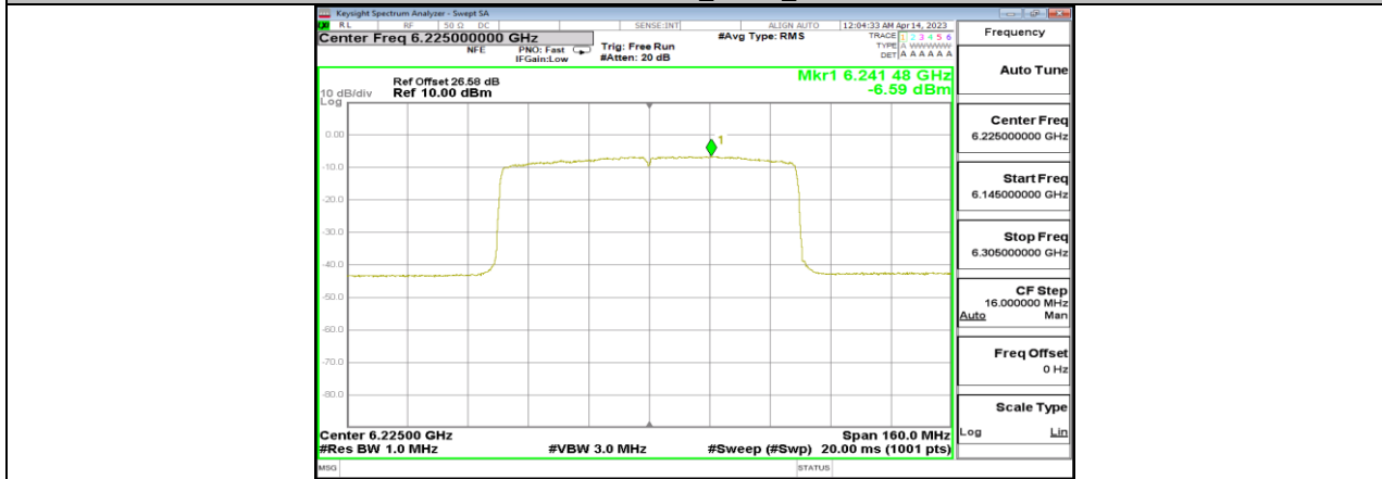
11AX80MIMO_Ant13_6225
