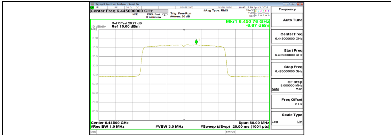
11AX40MIMO_Ant11_6445
