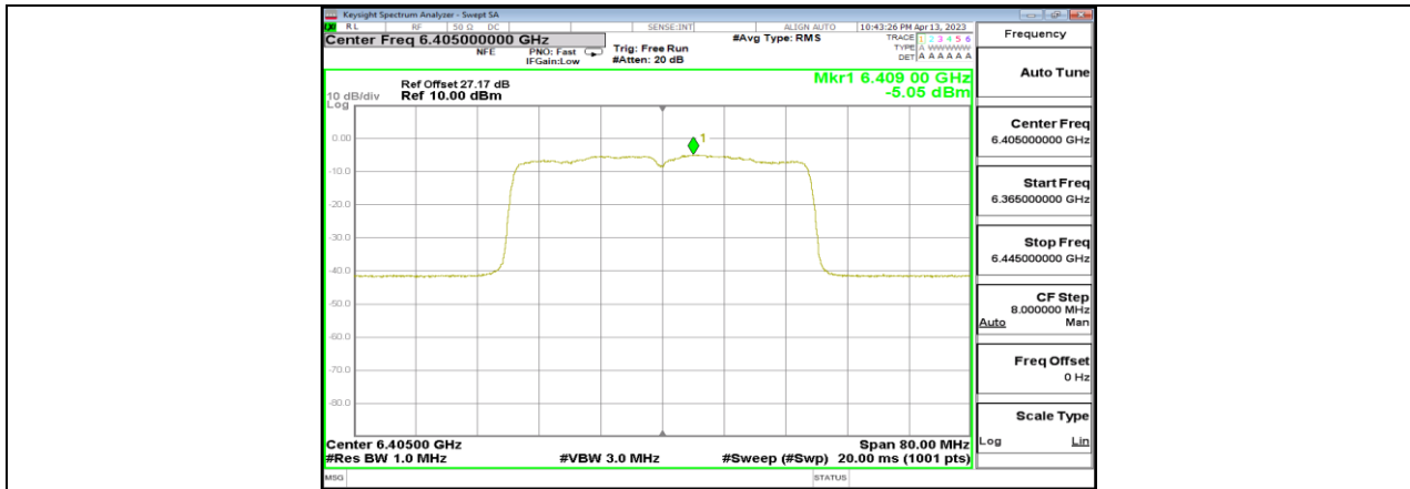
11AX40MIMO_Ant13_6405
