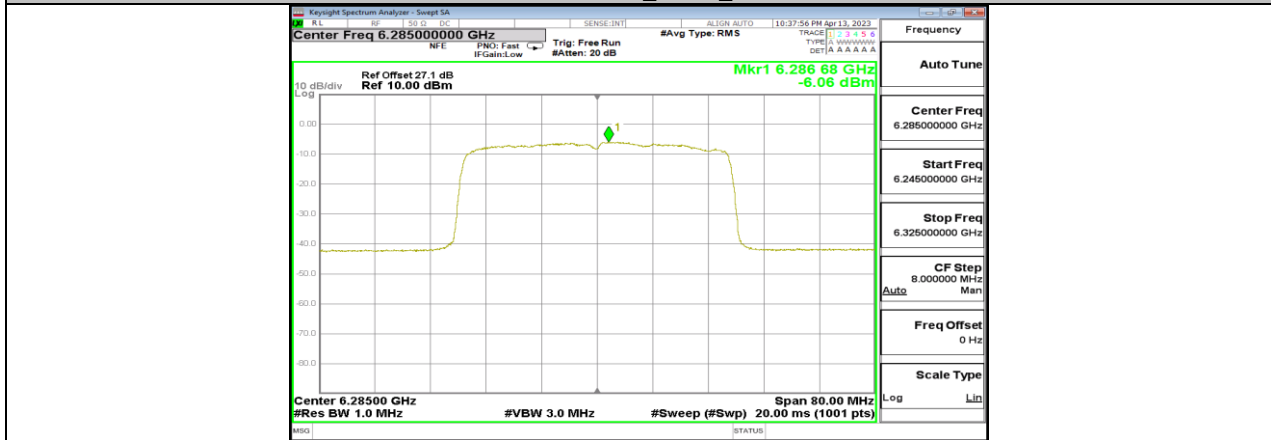
11AX40MIMO_Ant13_6285
