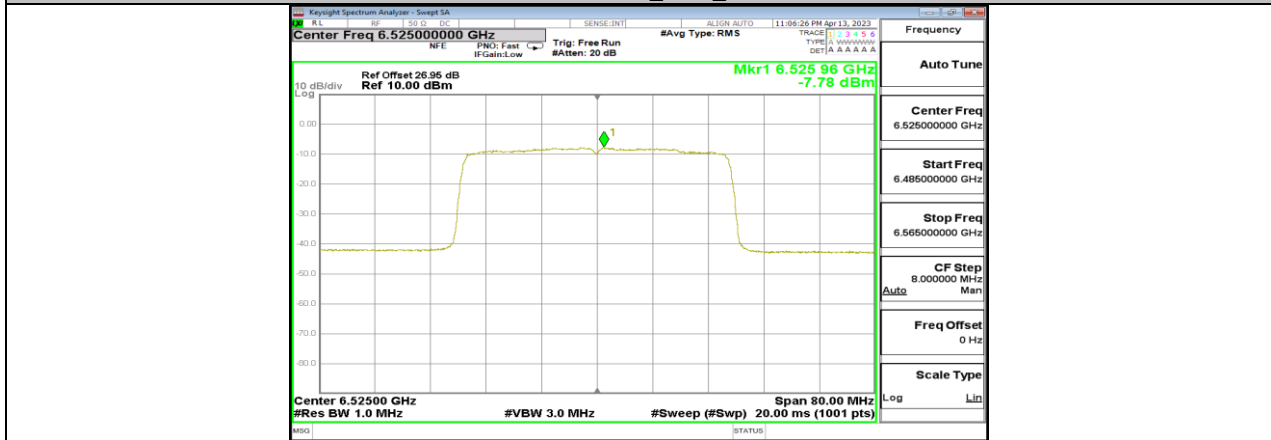
11AX40MIMO_Ant11_6525
