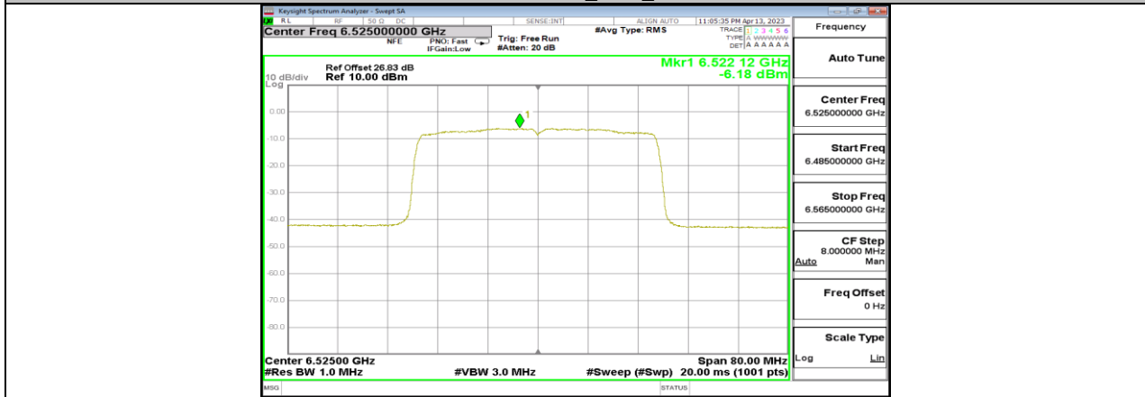
11AX40MIMO_Ant7_6525
