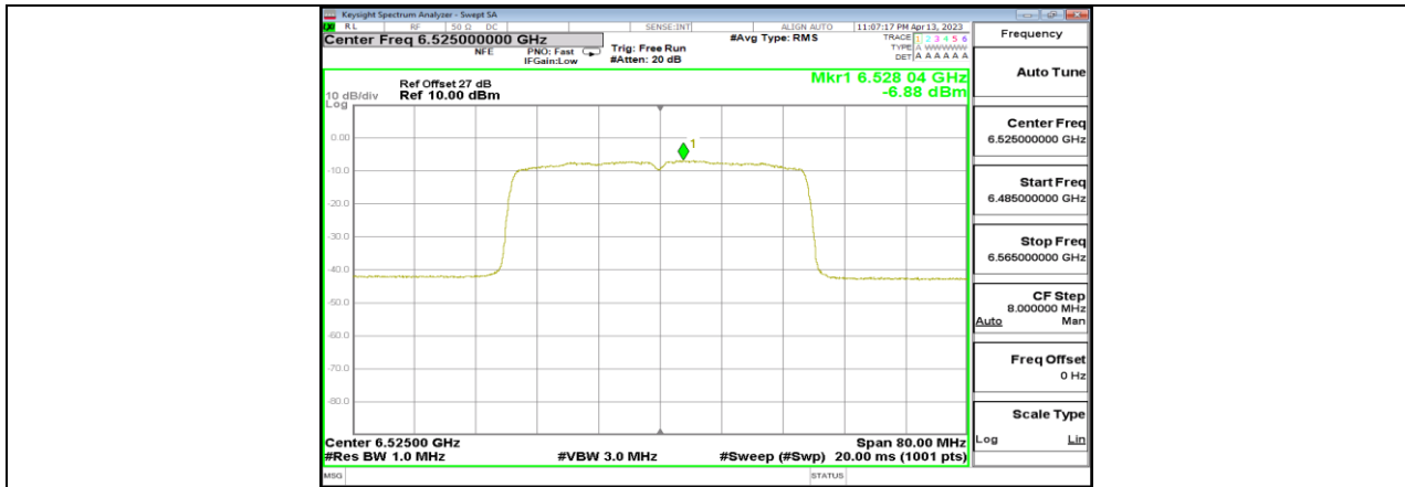
11AX40MIMO_Ant13_6525
