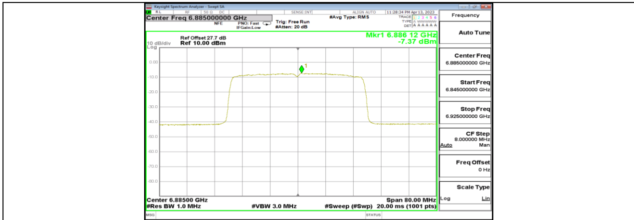
11AX40MIMO_Ant13_6885
