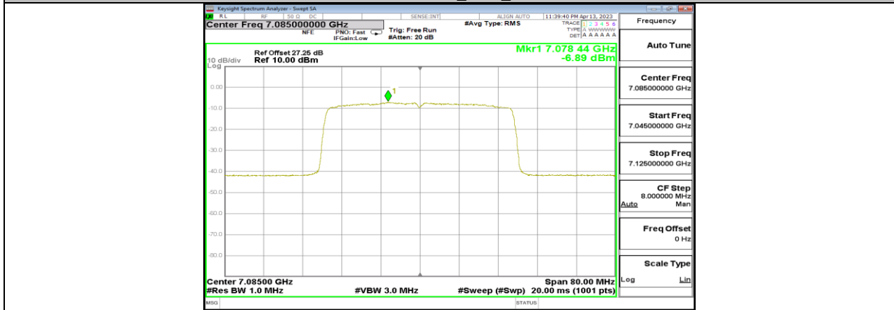
11AX40MIMO_Ant11_7085
