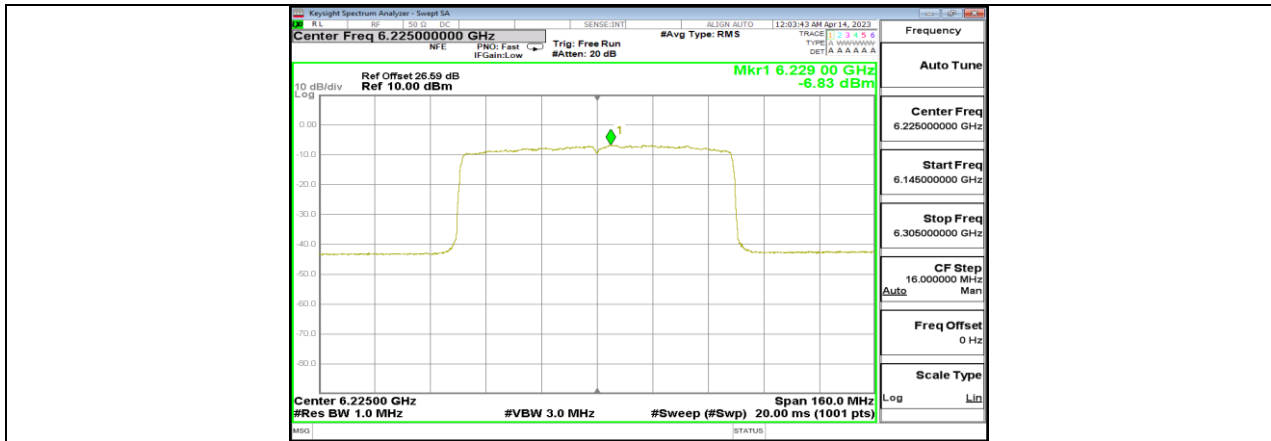
11AX80MIMO_Ant11_6225
