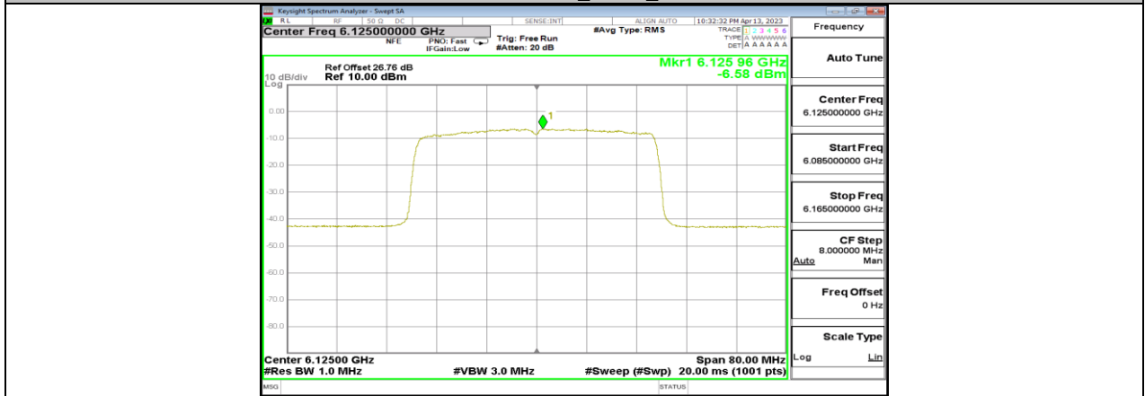
11AX40MIMO_Ant13_6125
