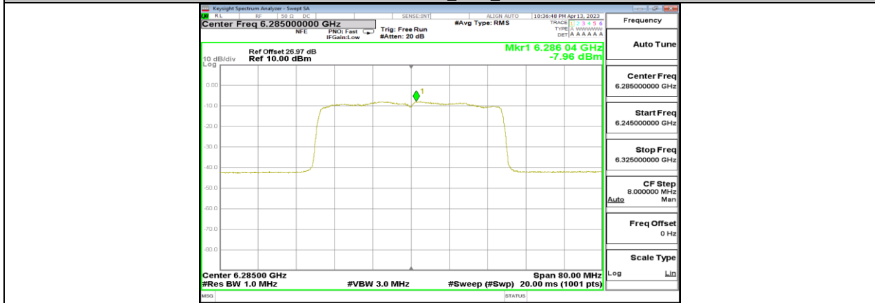
11AX40MIMO_Ant11_6285
