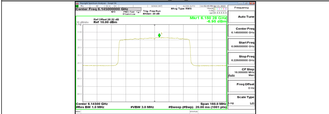
11AX80MIMO_Ant11_6145
