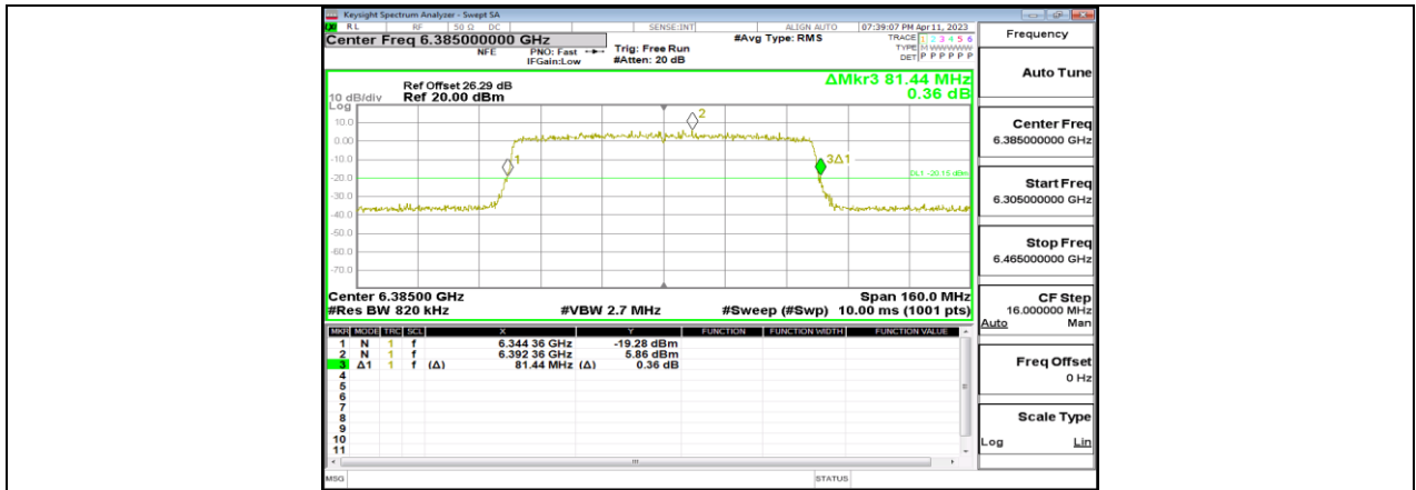
11AX80MIMO_Ant11_6385
