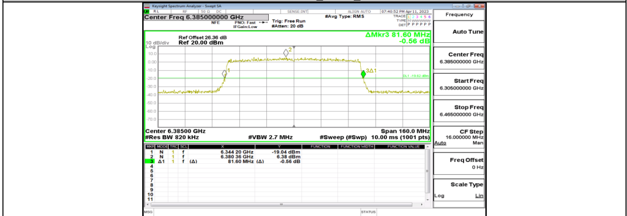
11AX80MIMO_Ant13_6385
