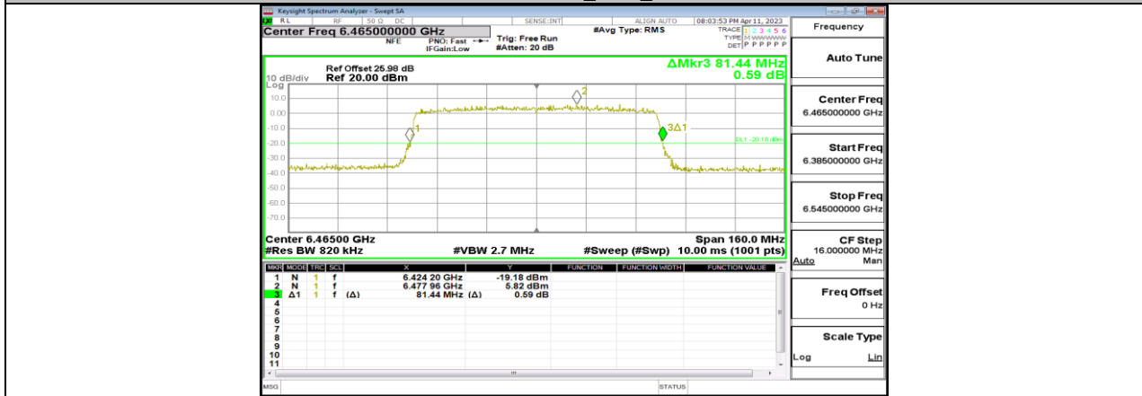
11AX80MIMO_Ant11_6465
