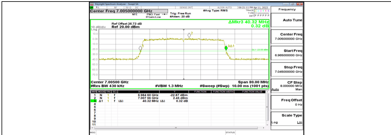
11AX40MIMO_Ant13_7005
