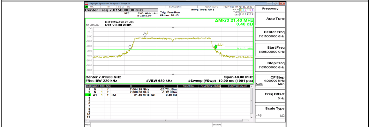
11AX20MIMO_Ant13_7015
