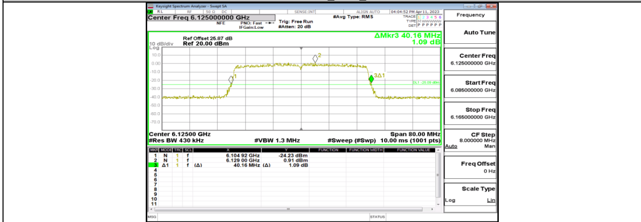
11AX40MIMO_Ant7_6125
