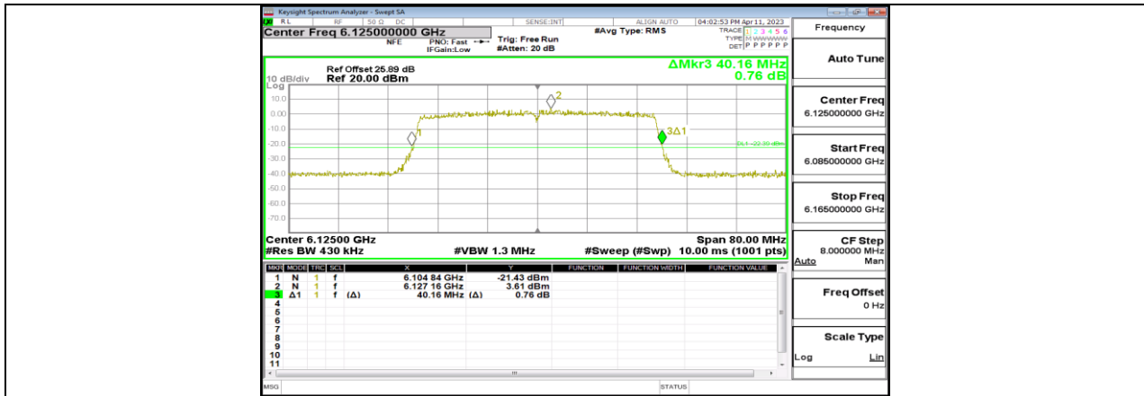
11AX40MIMO_Ant5_6125
