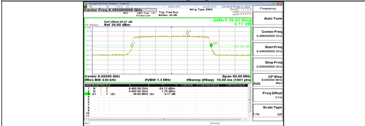
11AX40MIMO_Ant7_6485
