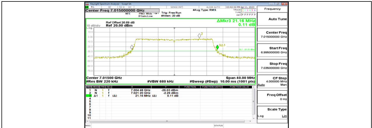
11AX20MIMO_Ant11_7015
