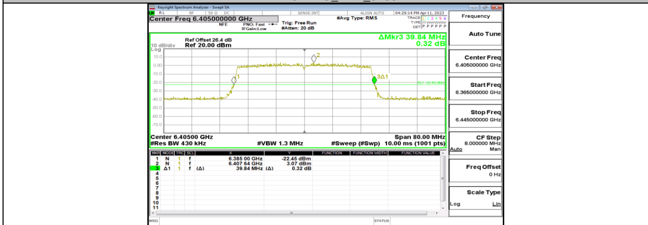
11AX40MIMO_Ant11_6405
