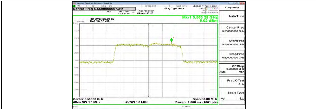
11AX40MIMO Ant15 5550
