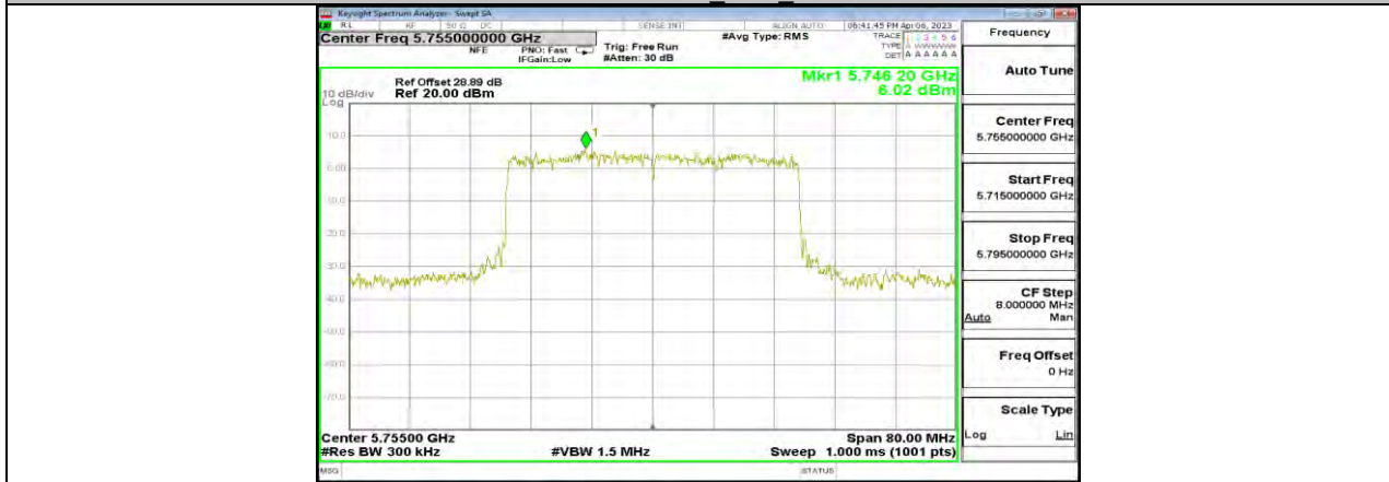
11AX40MIMO Ant10 5755
