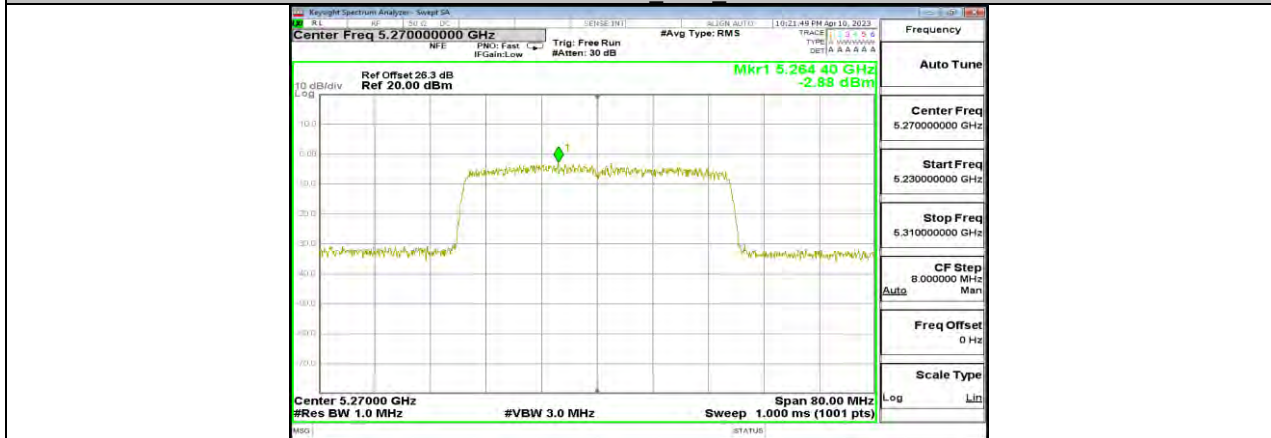
11AX40MIMO Ant10 5270
