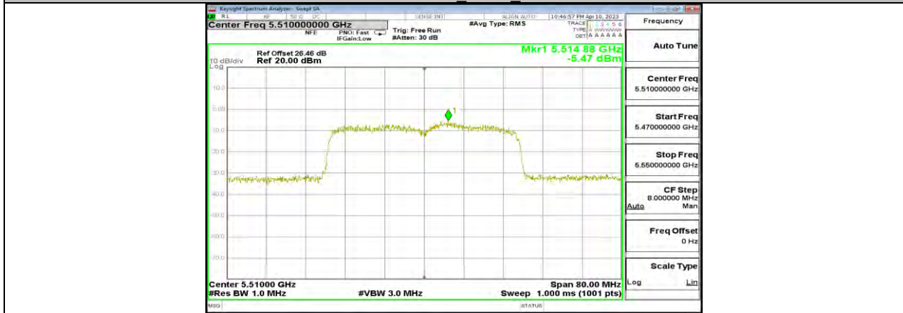
11AX40MIMO Ant15 5510
