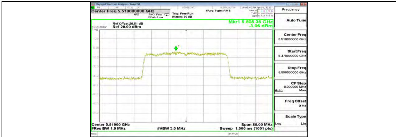
11AX40MIMO Ant10 5510
