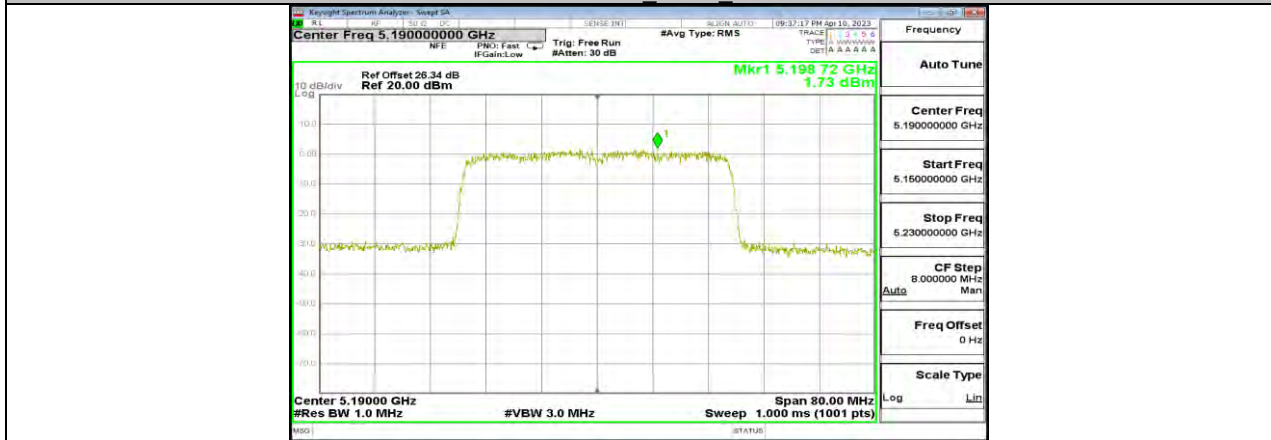
11AX40MIMO Ant15 5190
