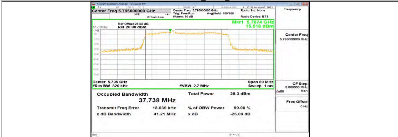
11AX40MIMO Ant16 5795
