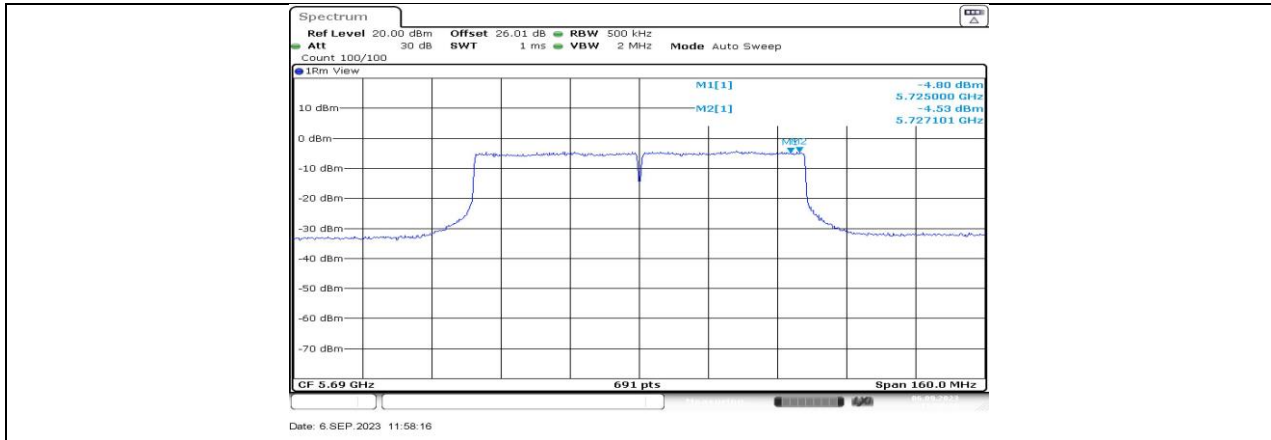
11AC80MIMO_Ant3_5690_UNII-3
