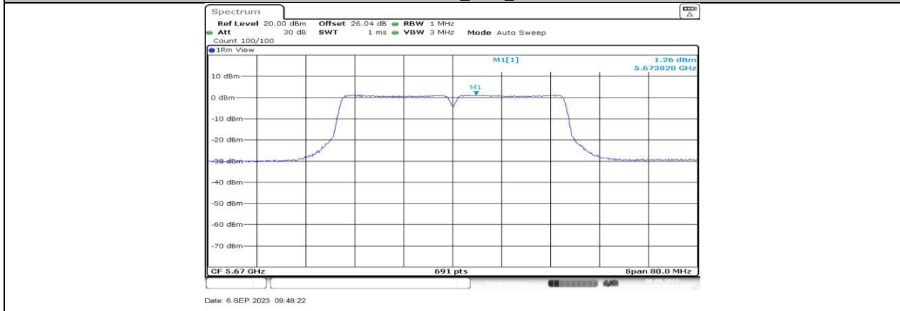
11AC40MIMO_Ant3_5670
