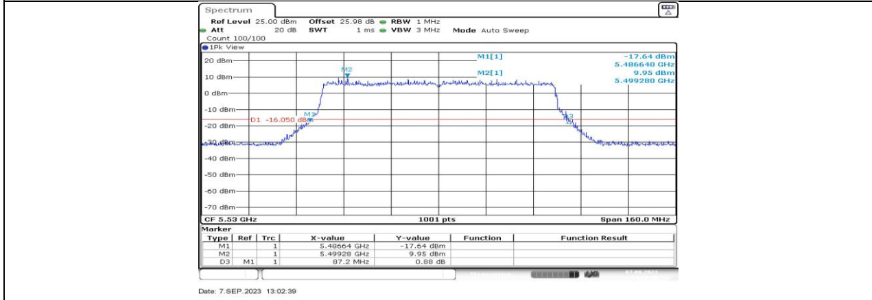
11BE80MIMO_Ant2_5530
