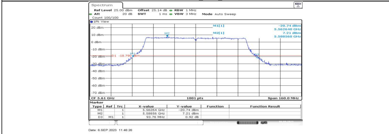
11AC80MIMO_Ant3_5610
