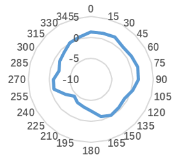
7125MHz
