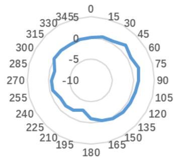
6525MHz
