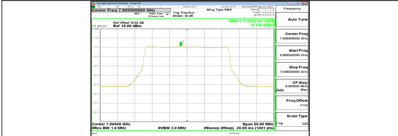
11BE40MIMO_Ant1_7005
