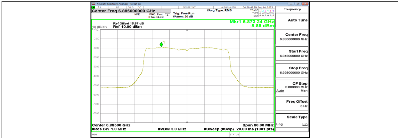
11BE40MIMO_Ant4_6885
