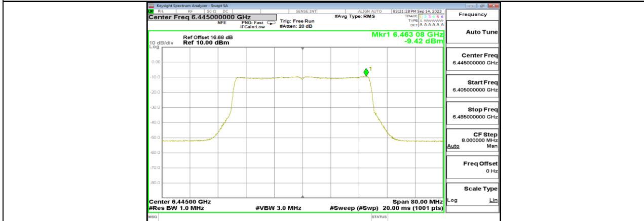
11BE40MIMO_Ant2_6445
