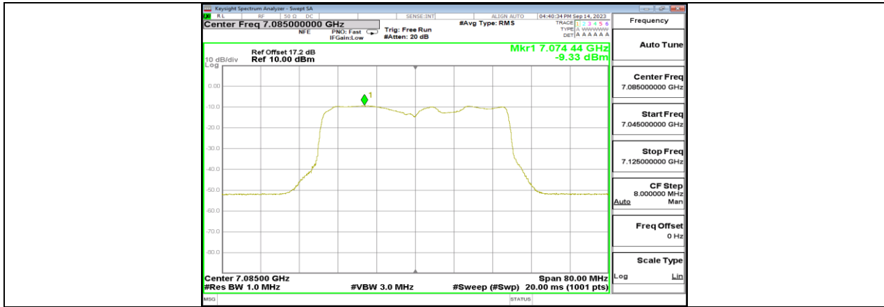
11BE40MIMO_Ant3_7085
