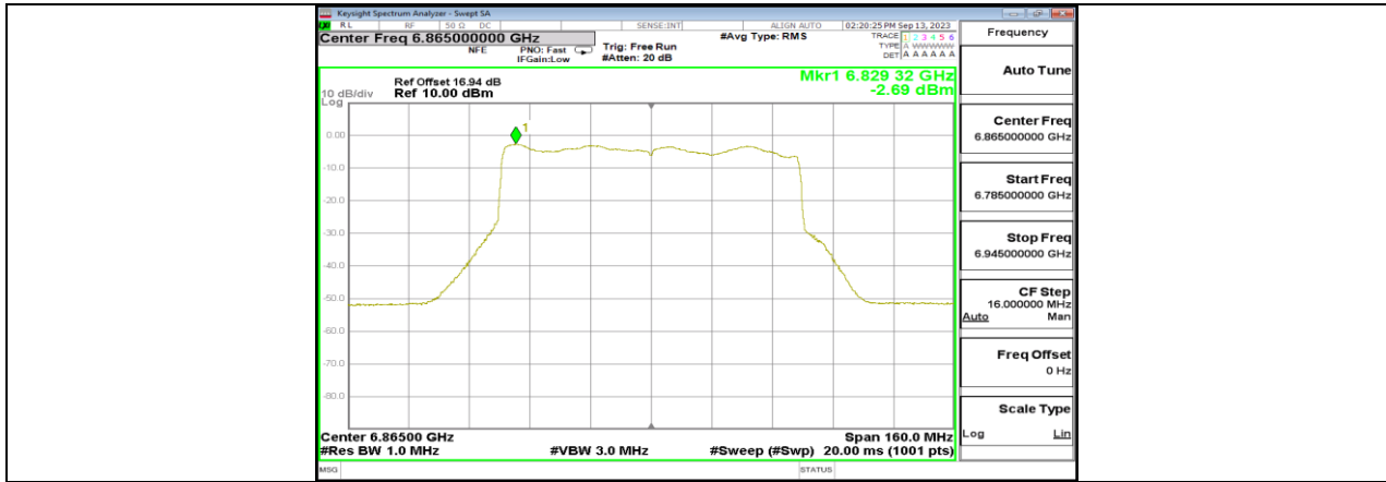
11BE80MIMO_Ant3_6865
