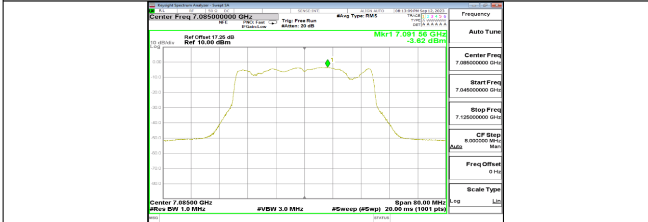
11BE40MIMO_Ant4_7085
