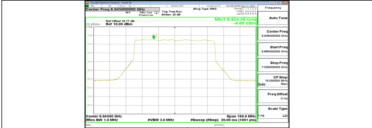
11BE80MIMO_Ant1_6945
