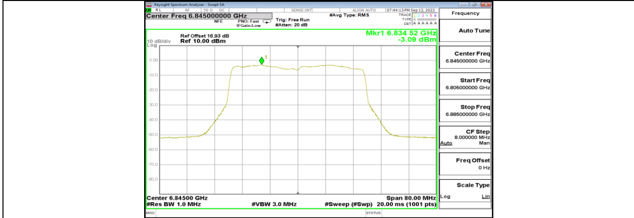
11BE40MIMO_Ant3_6845
