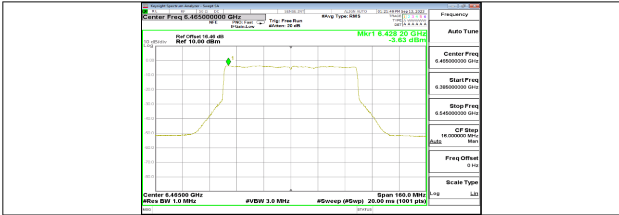
11BE80MIMO_Ant1_6465
