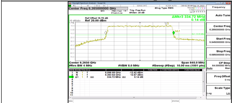
11BE320MIMO_Ant3_6265
