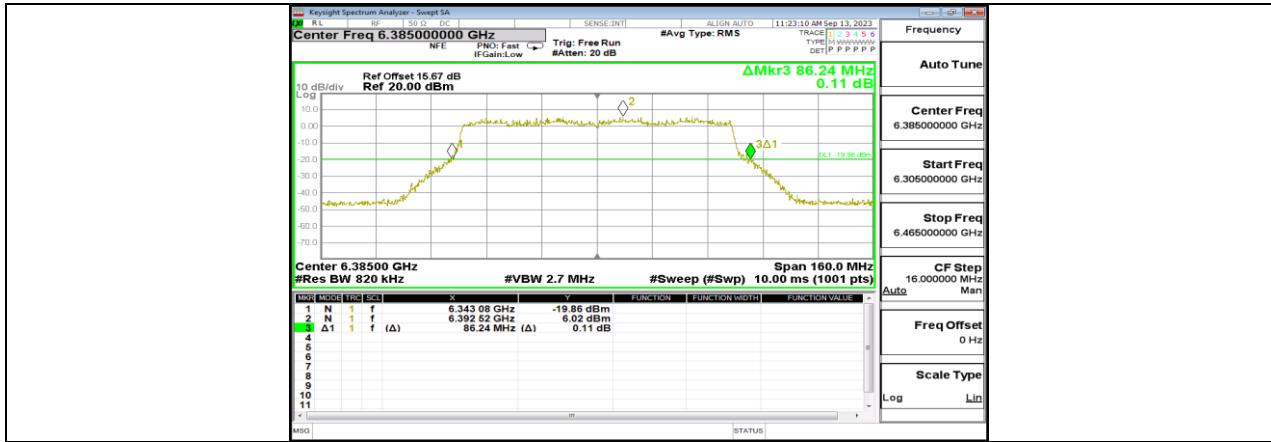
11BE80MIMO_Ant4_6385
