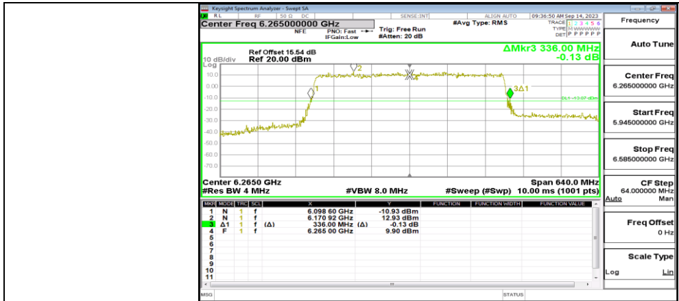
11BE320MIMO_Ant1_6265
