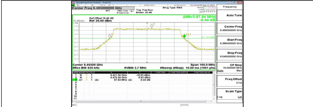
11BE80MIMO_Ant1_6465
