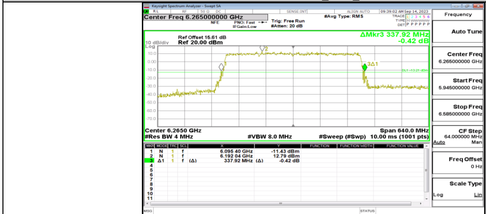
11BE320MIMO_Ant2_6265
