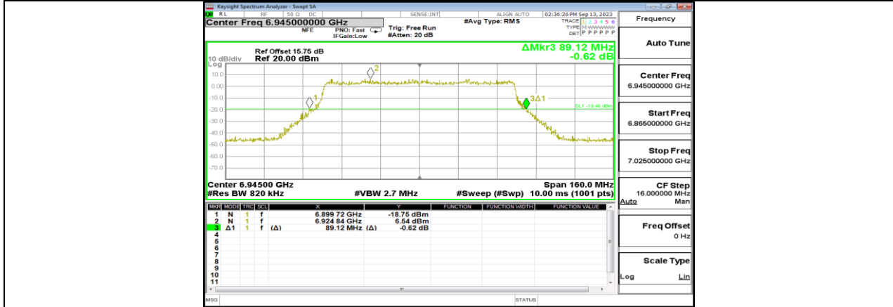
11BE80MIMO_Ant4_6865
