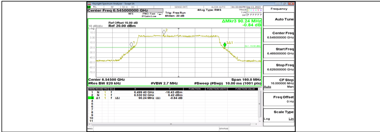
11BE80MIMO_Ant3_6545
