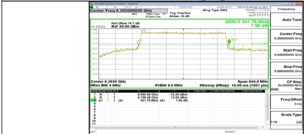
11BE320MIMO_Ant3_6265
