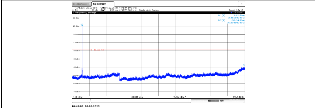
11B-CDD_Ant1_2457_1000~26500
