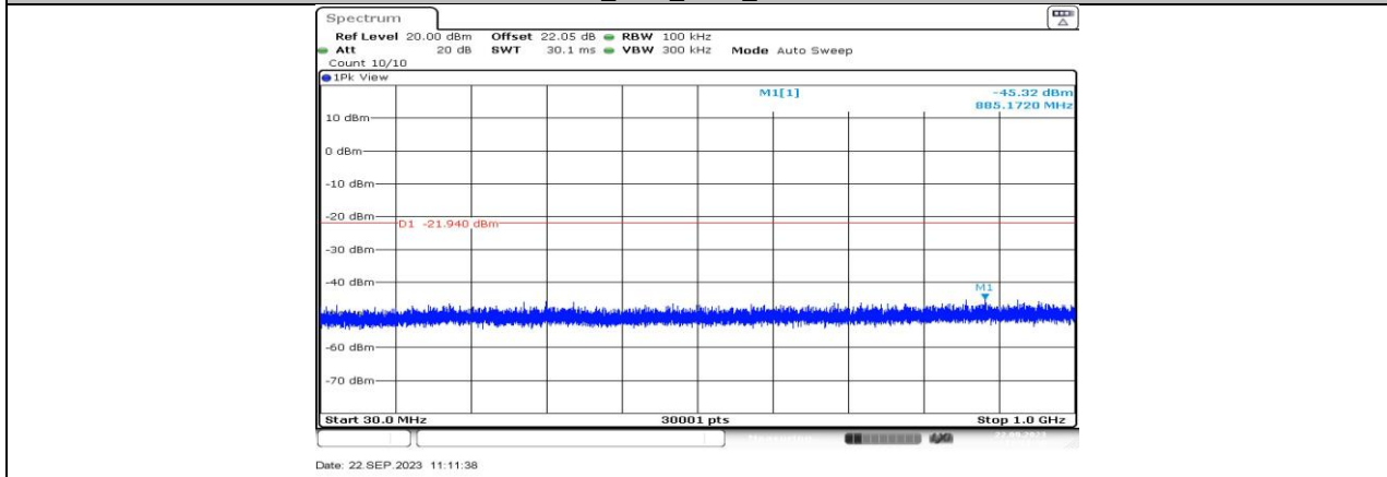
11G-CDD_Ant1_2457_30~1000
