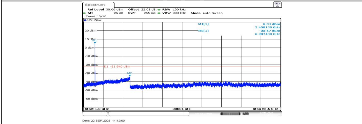
11G-CDD_Ant1_2457_1000~26500
