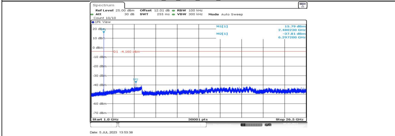
BLE_1M_Ant3_2480_1000~26500
