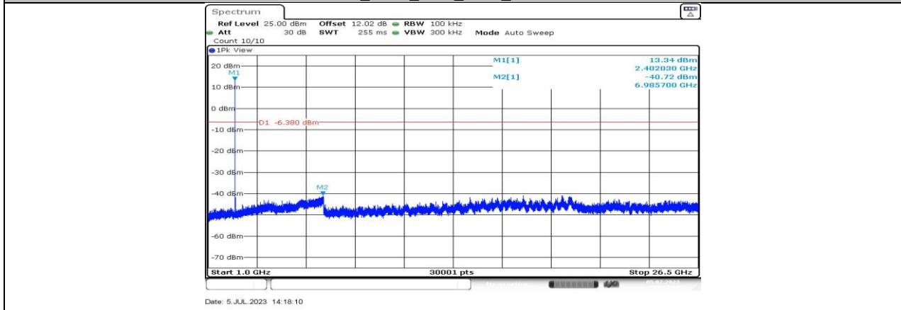
BLE_500K_Ant3_2402_1000~26500
