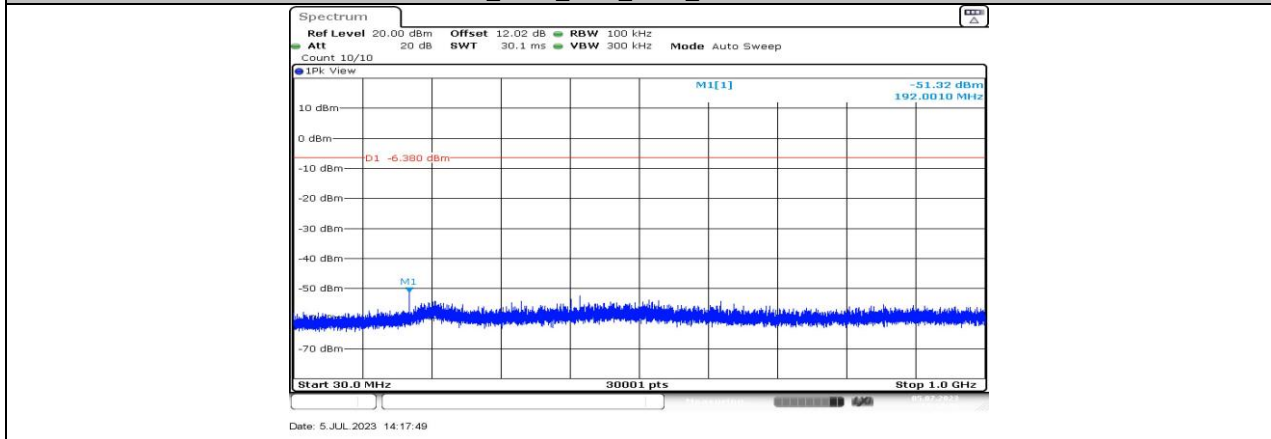
BLE_500K_Ant3_2402_30~1000
