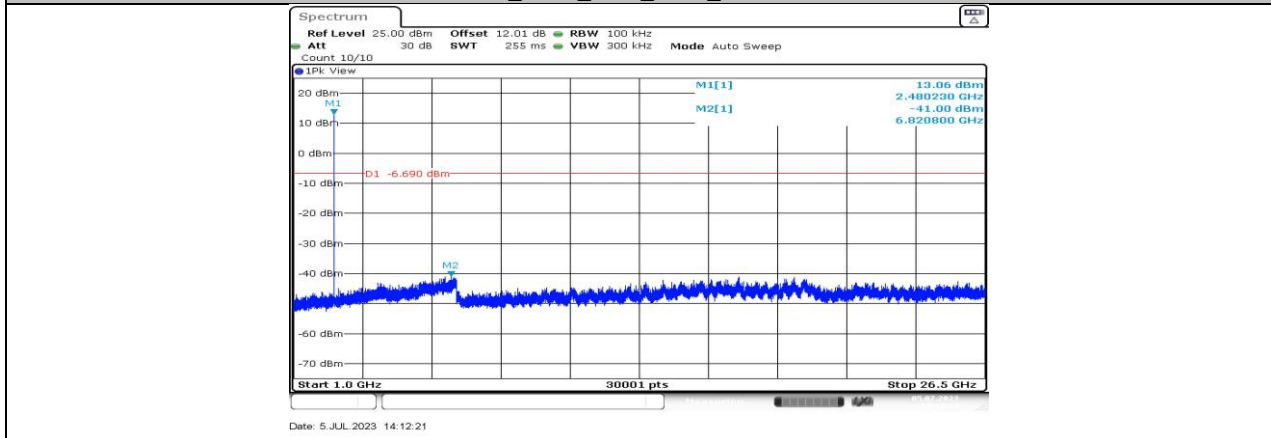
BLE_125K_Ant3_2480_1000~26500
