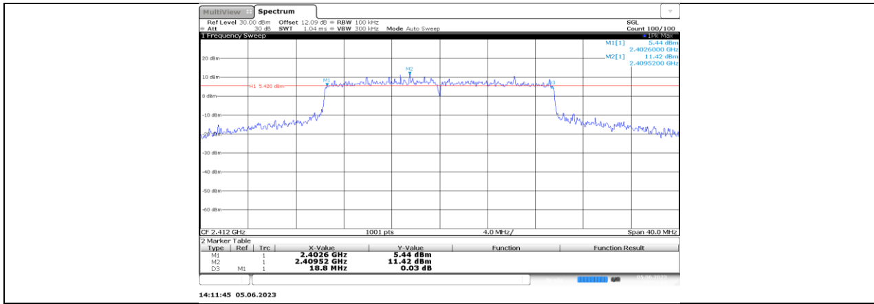
11AX20MIMO_Ant2_2412
