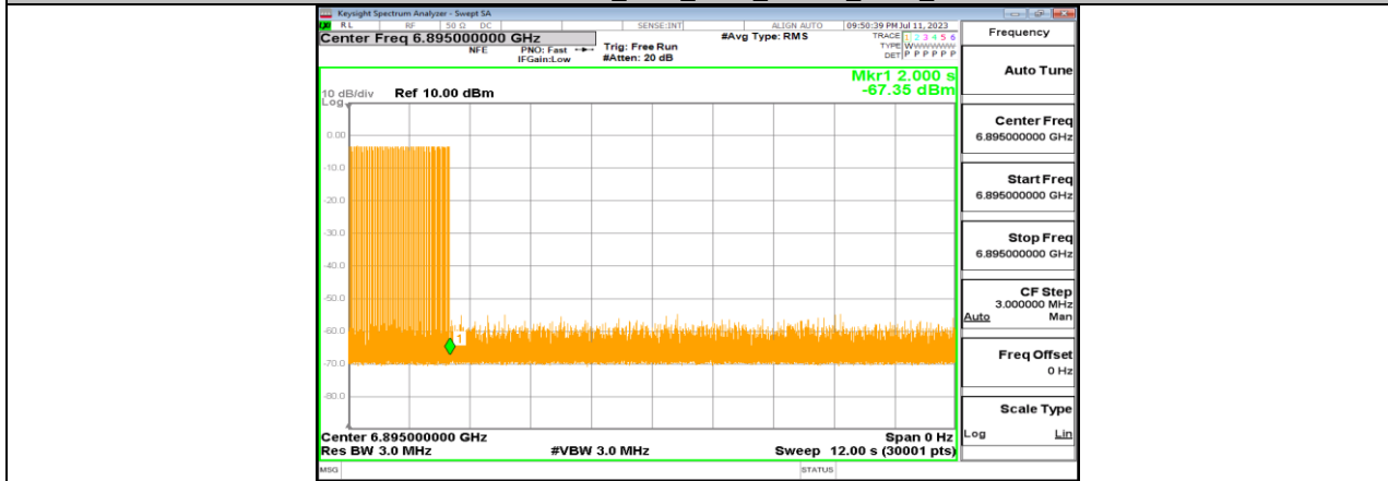
11BE20MIMO_Ant4_6895_Center_6895_7
