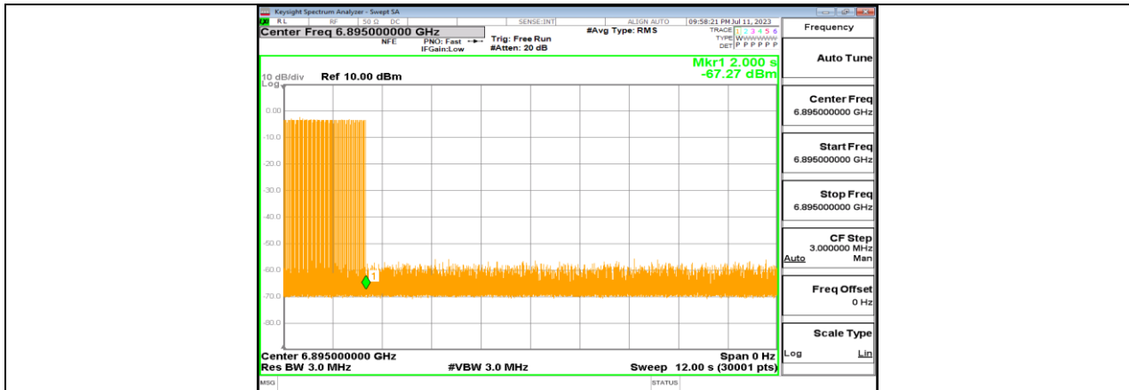
11BE20MIMO_Ant4_6895_Center_6895_9
