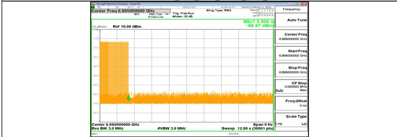
11BE20MIMO_Ant4_6895_Center_6895_4
