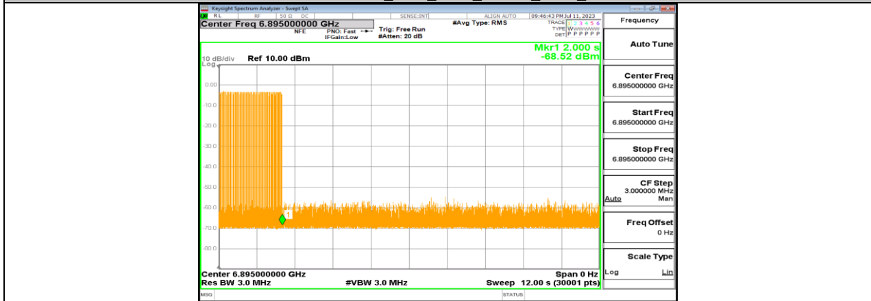
11BE20MIMO_Ant4_6895_Center_6895_5
