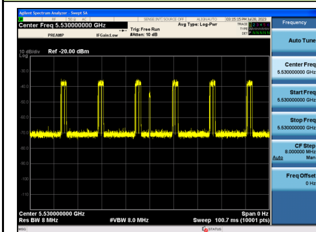
802.11ax-HE80 (5530MHz)
