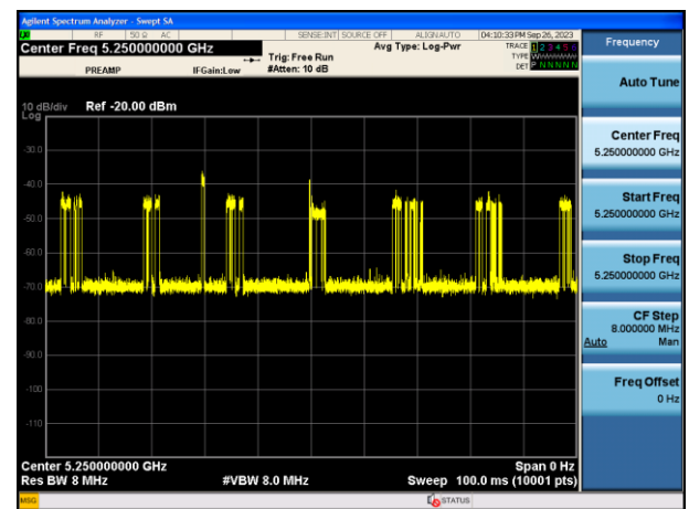
802.11ax-HE160 (5250MHz)
