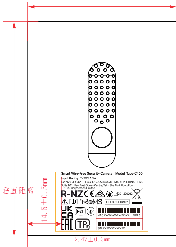
尺寸图
