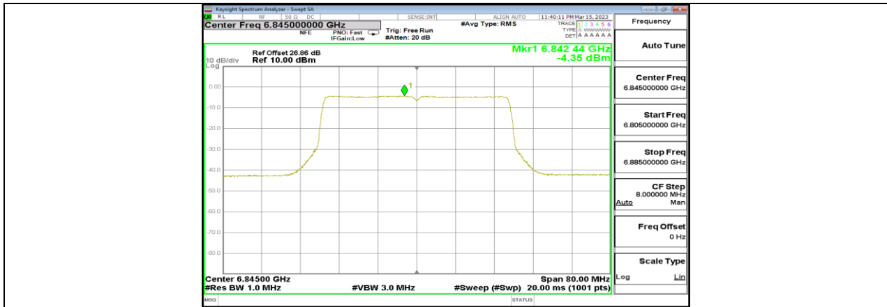
11AX40MIMO_Ant6_6845
