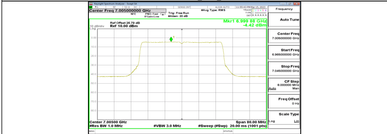
11AX40MIMO_Ant6_7005
