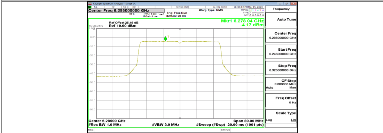
11AX40MIMO_Ant8_6285
