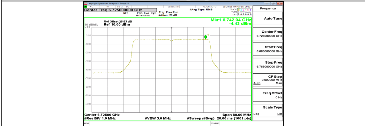
11AX40MIMO_Ant6_6725
