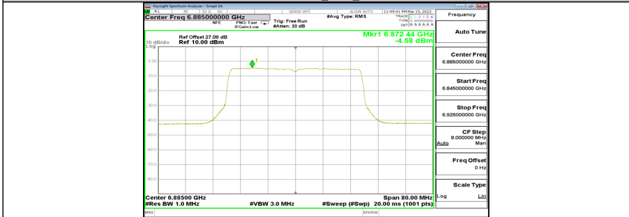
11AX40MIMO_Ant8_6885
