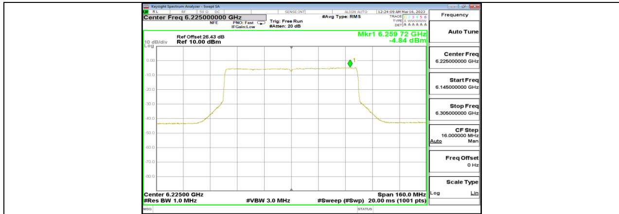
11AX80MIMO_Ant8_6225
