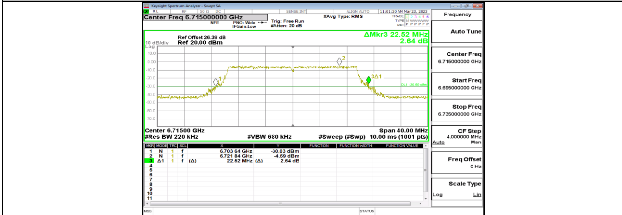
11BE20MIMO_Ant4_6715
