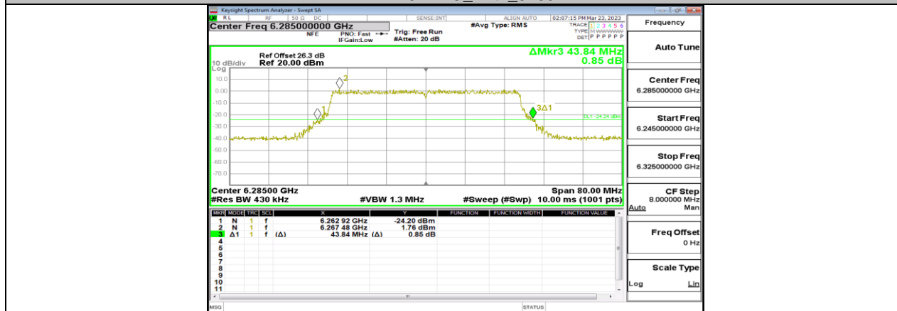
11BE40MIMO_Ant6_6285
