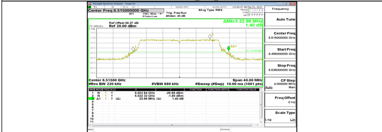
11BE20MIMO_Ant8_6515
