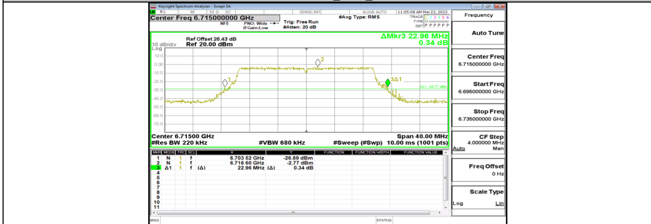
11BE20MIMO_Ant6_6715
