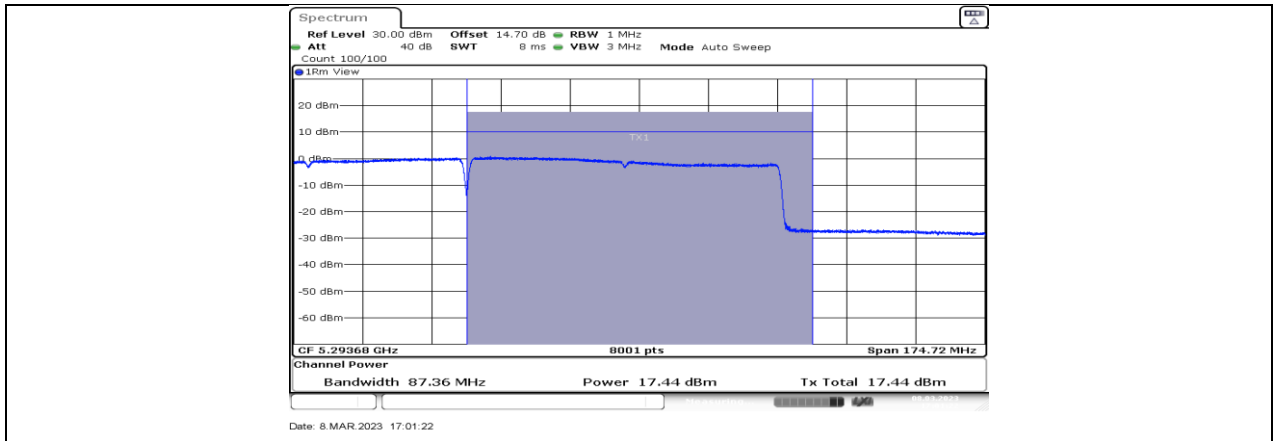
11BE160MIMO_Ant3_5250_UNII-2A
