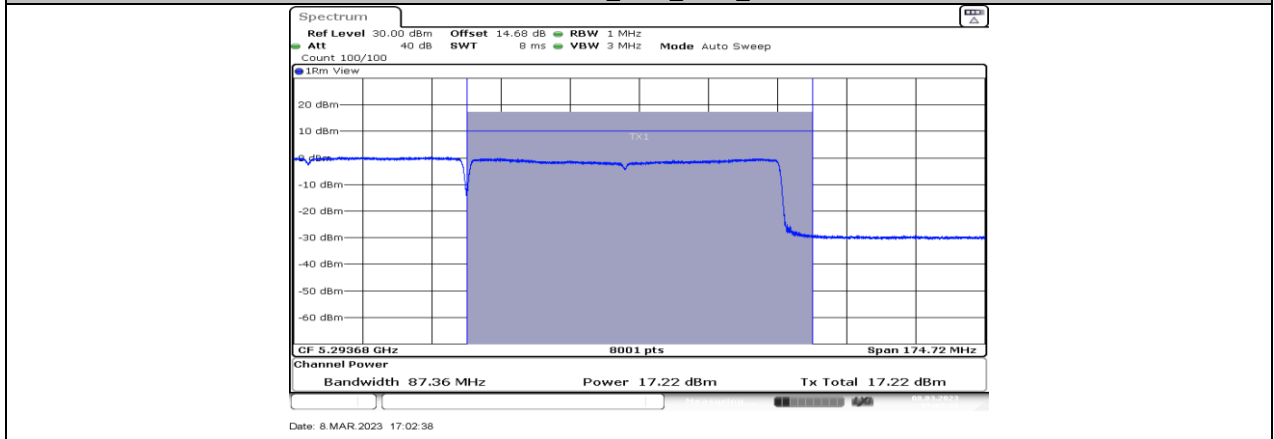
11BE160MIMO_Ant4_5250_UNII-2A
