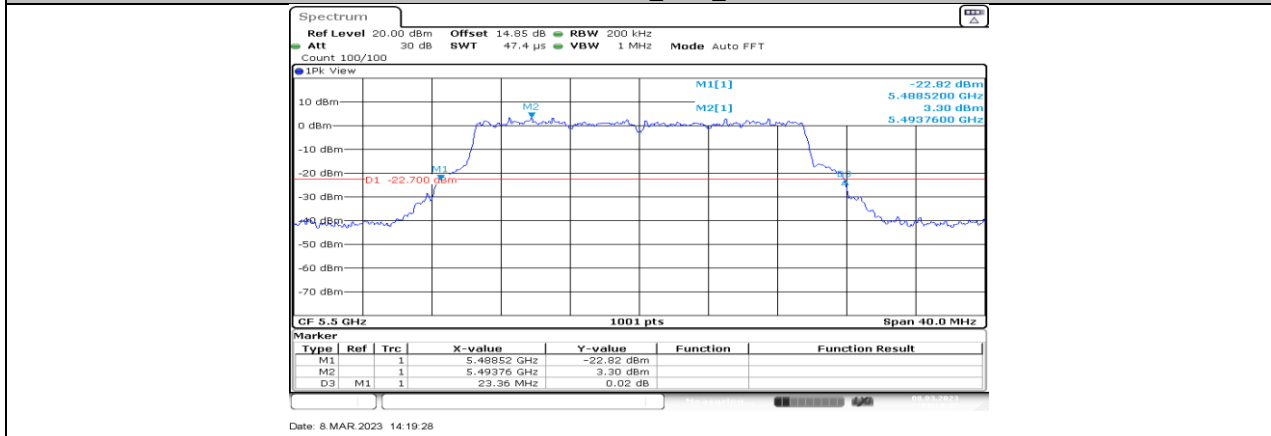
11BE20MIMO_Ant4_5500
