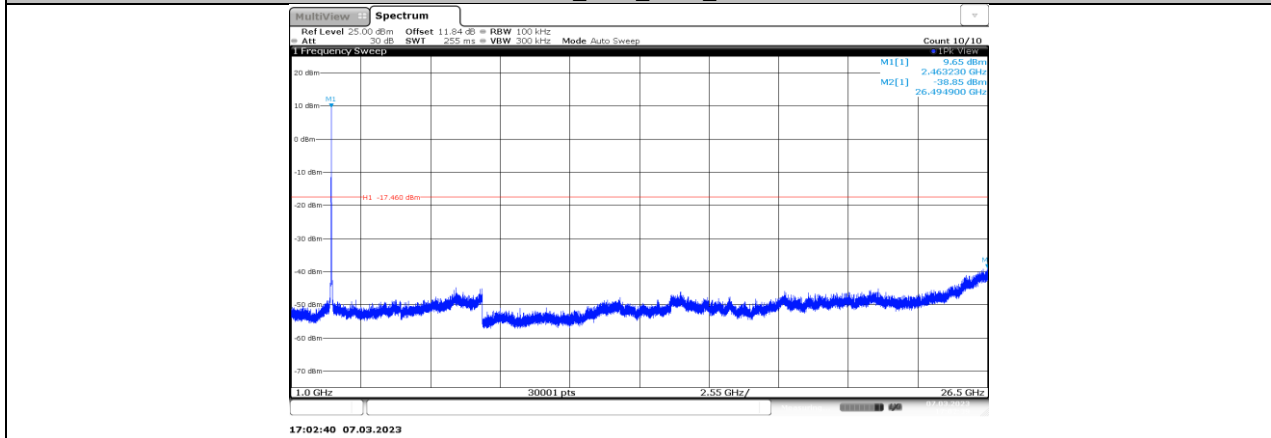
11G-CDD_Ant5_2462_1000~26500
