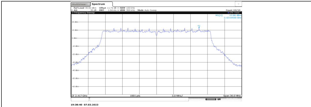
11AX20MIMO_Ant5_2417_0-Reference
