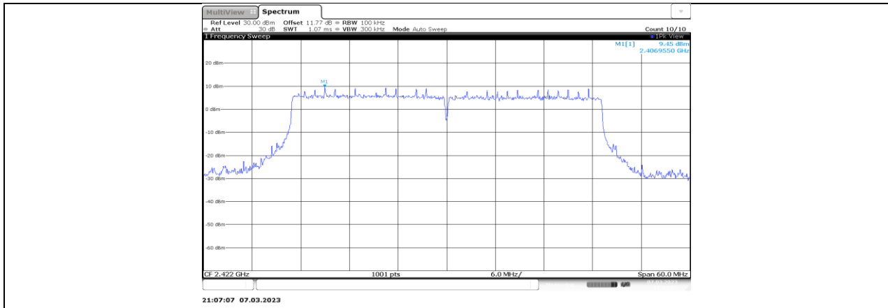
11AX40MIMO_Ant7_2422_0-Reference
