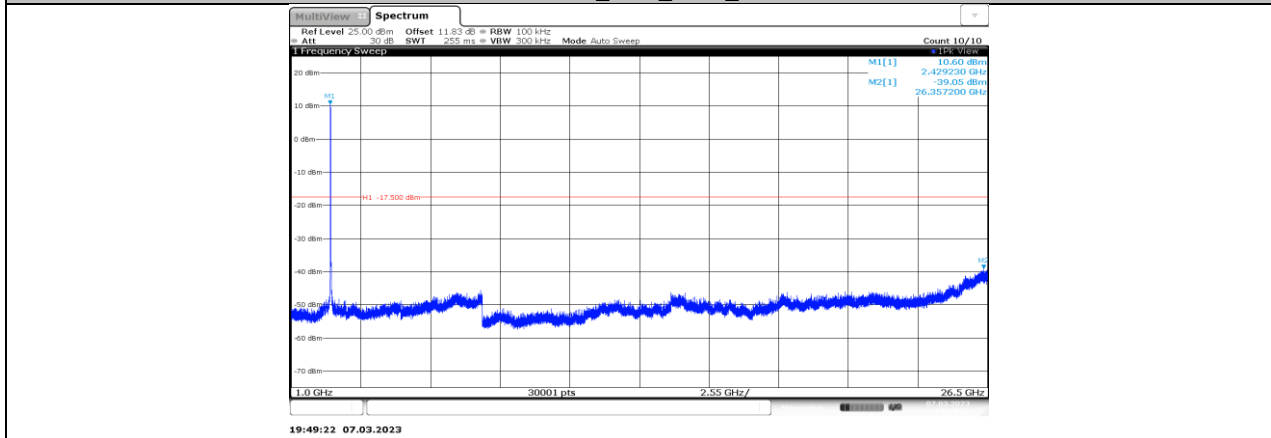
11AX20MIMO_Ant5_2437_1000~26500
