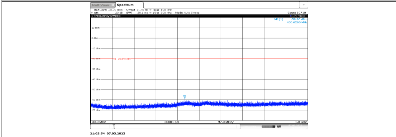
11AX40MIMO_Ant5_2422_30~1000
