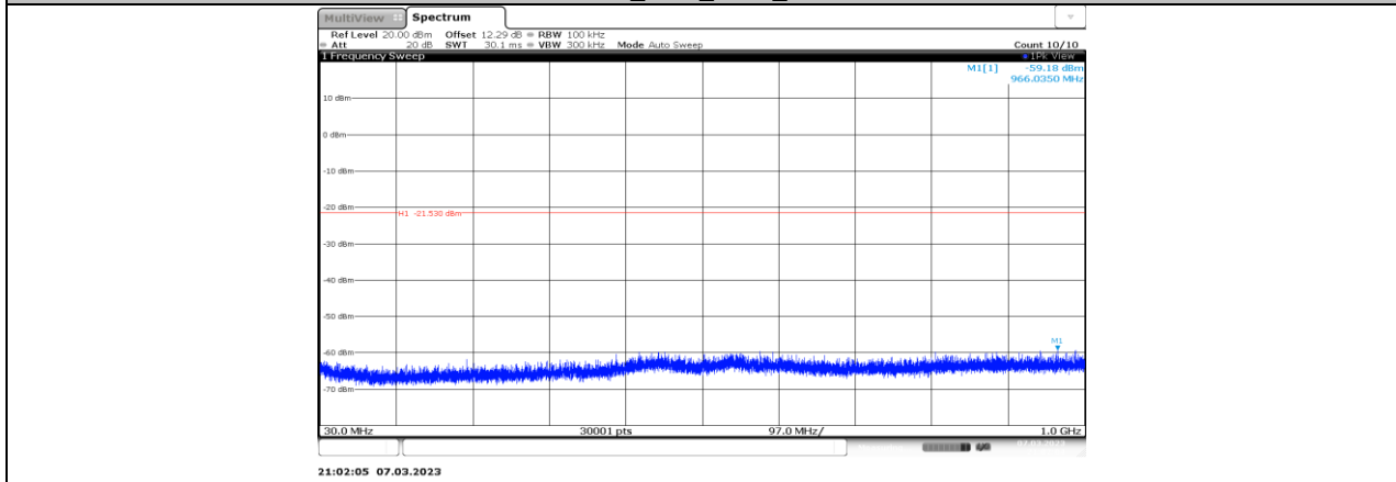
11AX40MIMO_Ant3_2422_30~1000
