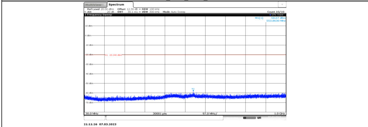
11AX40MIMO_Ant3_2427_30~1000
