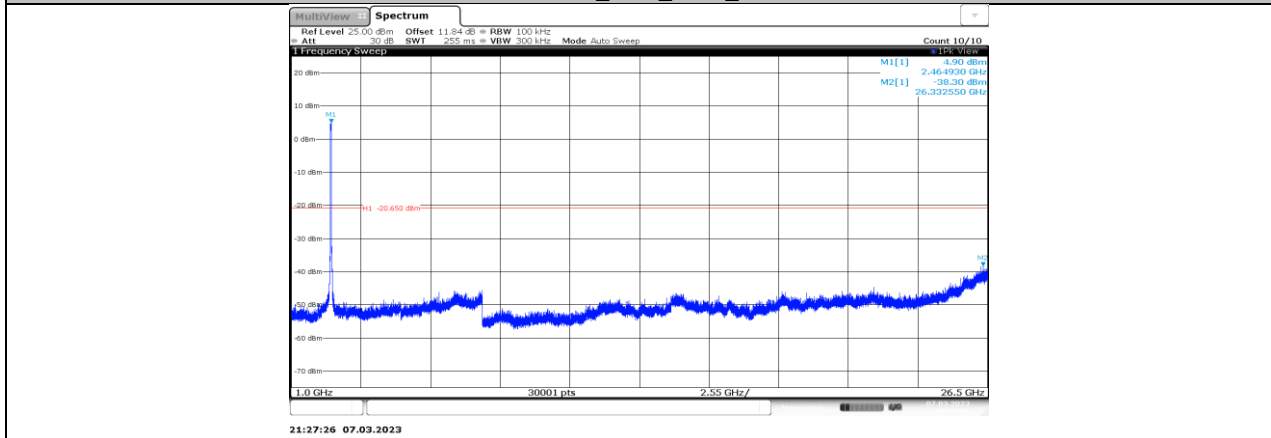
11AX40MIMO_Ant7_2447_1000~26500
