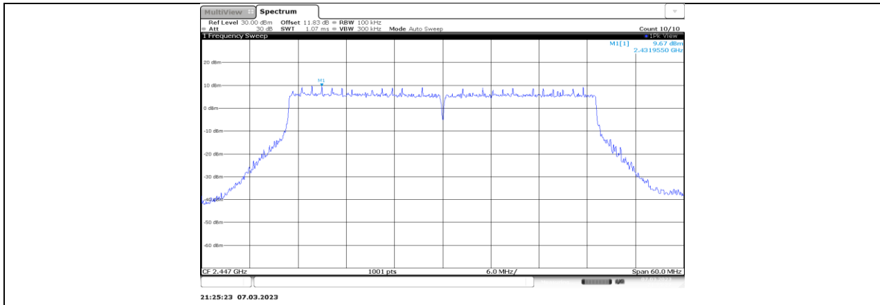
11AX40MIMO_Ant5_2447_0-Reference
