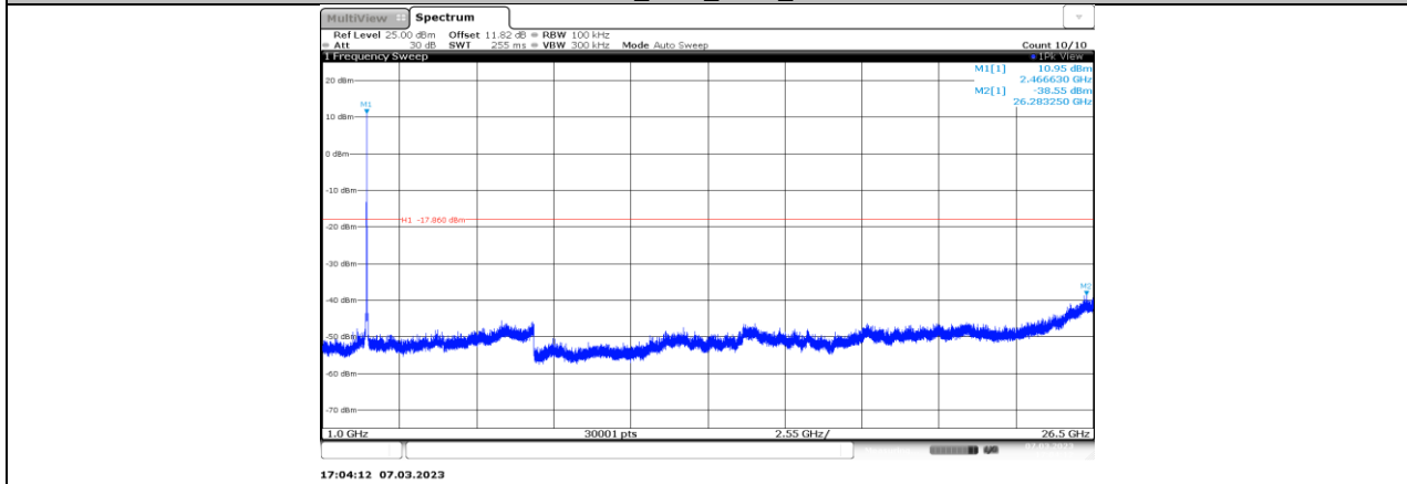
11G-CDD_Ant7_2462_1000~26500
