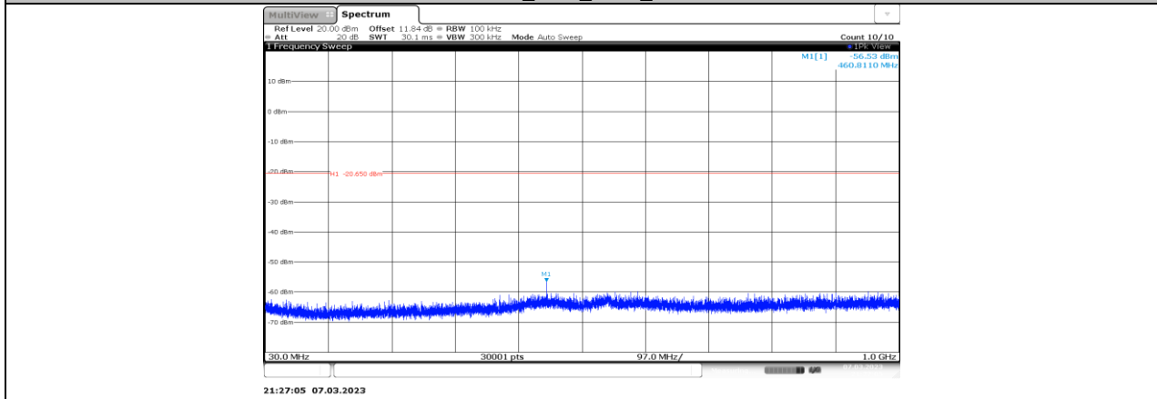
11AX40MIMO_Ant7_2447_30~1000
