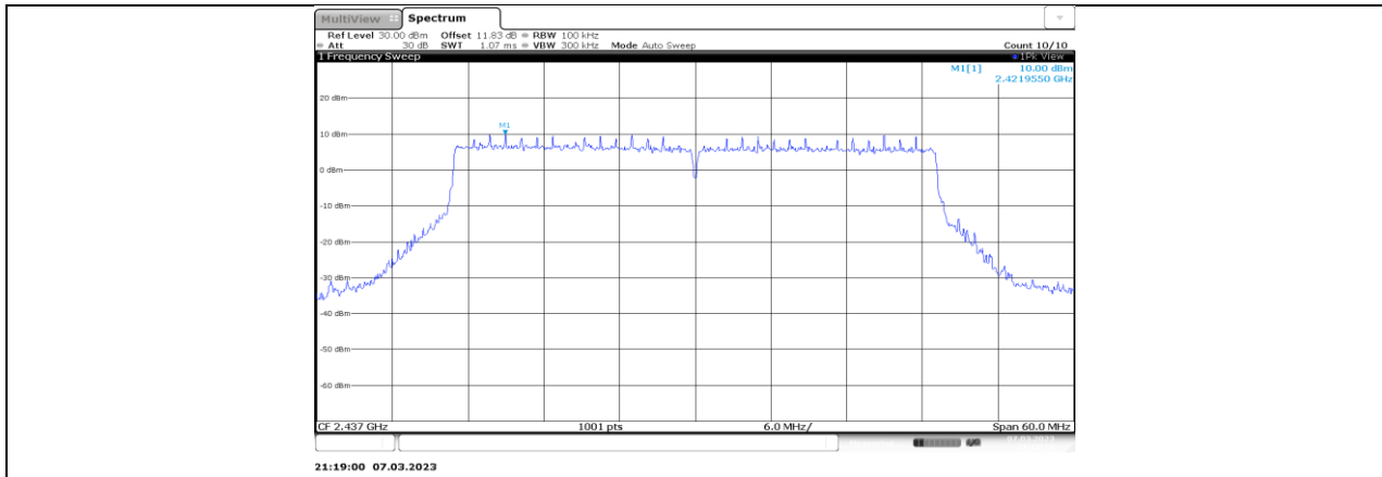
11AX40MIMO_Ant5_2437_0-Reference
