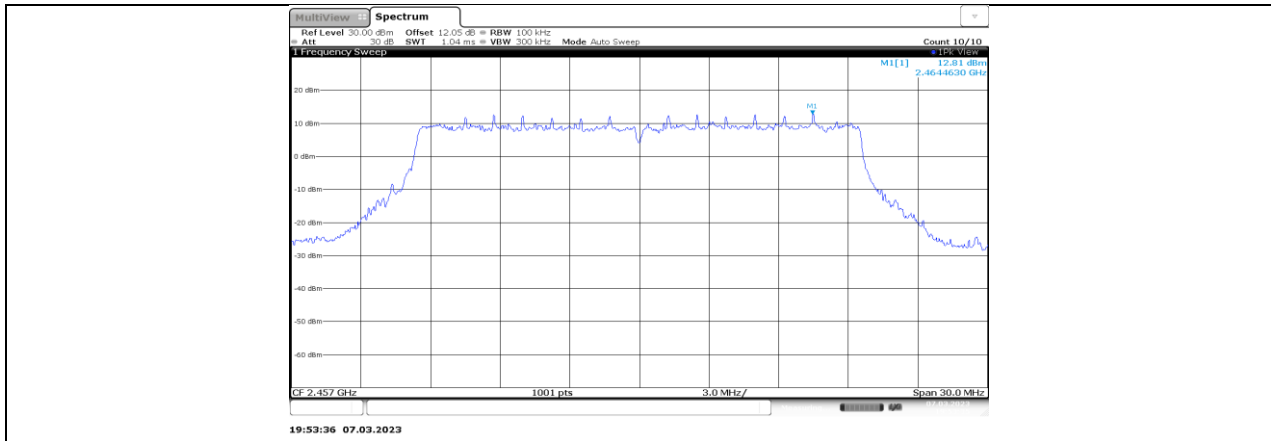
11AX20MIMO_Ant1_2457_0-Reference
