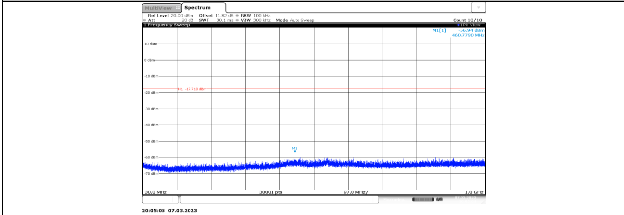
11AX20MIMO_Ant7_2462_30~1000
