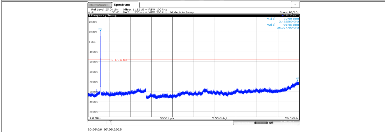
11AX20MIMO_Ant7_2462_1000~26500
