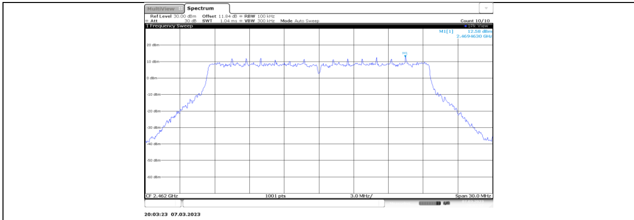
11AX20MIMO_Ant5_2462_0-Reference
