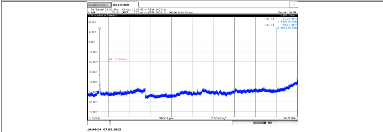
11AX20MIMO_Ant1_2457_1000~26500
