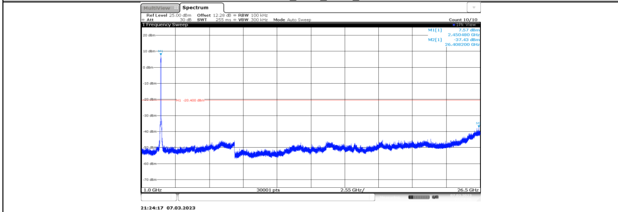
11AX40MIMO_Ant3_2447_1000~26500
