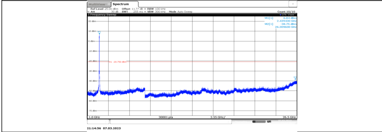
11AX40MIMO_Ant7_2427_1000~26500
