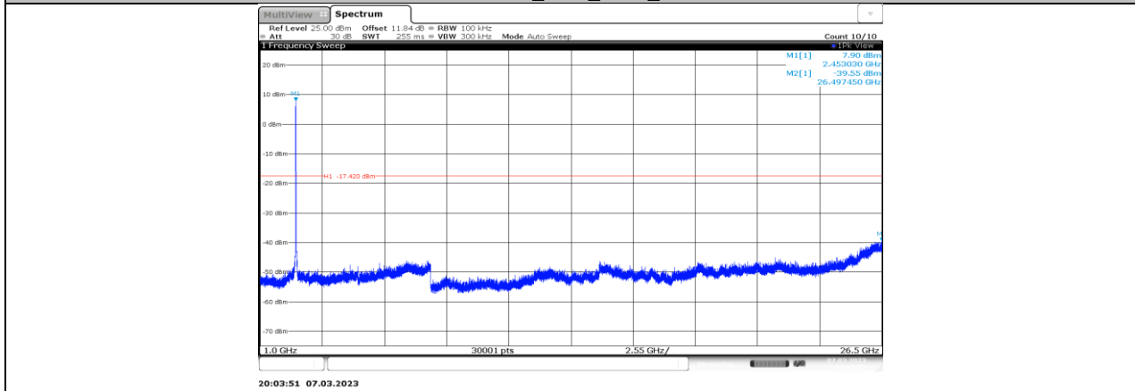
11AX20MIMO_Ant5_2462_1000~26500
