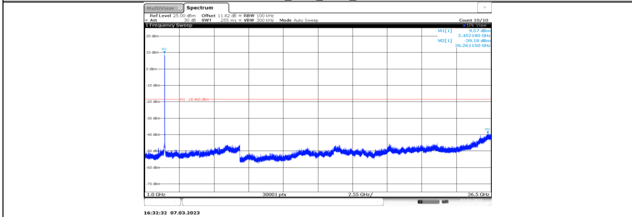
11G-CDD_Ant7_2457_1000~26500
