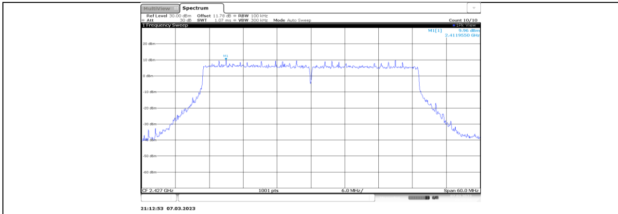
11AX40MIMO_Ant5_2427_0-Reference
