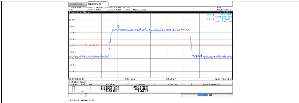
11BE20-CDD_Ant3_5955
