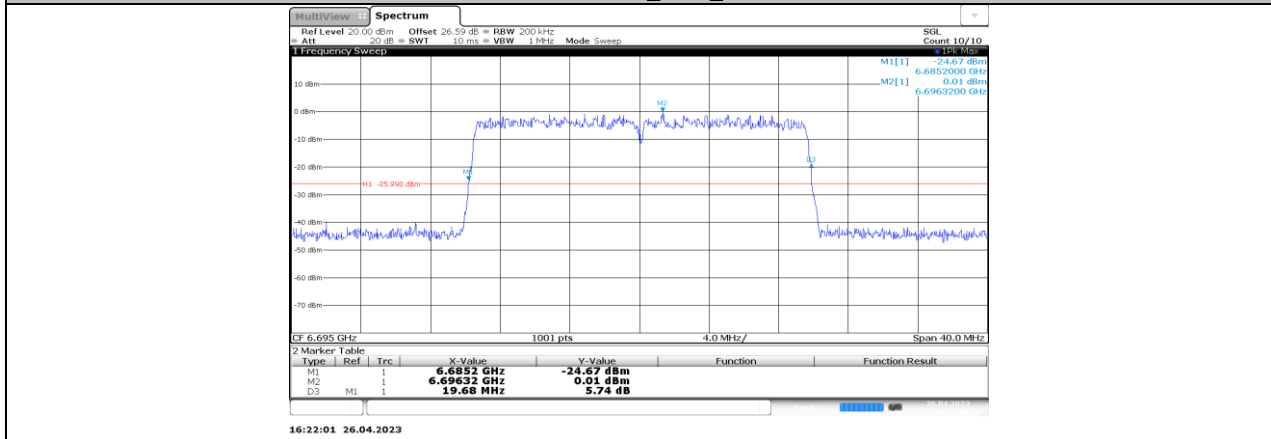
11BE20-CDD_Ant3_6695
