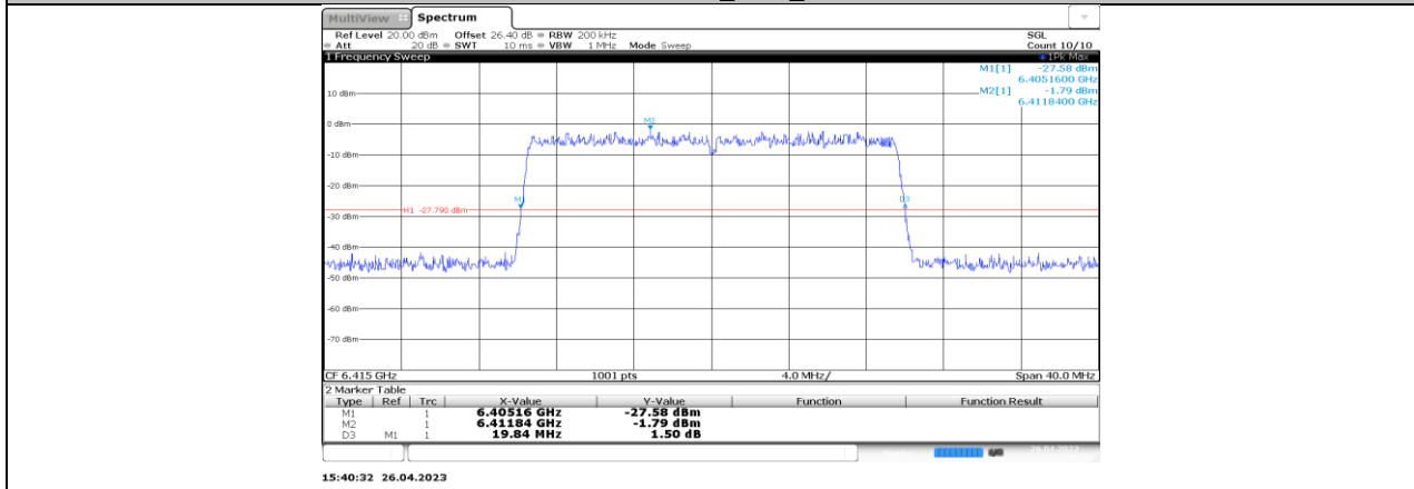
11BE20-CDD_Ant3_6415
