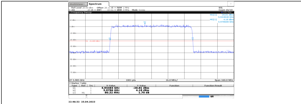
11AX80-CDD_Ant1_5985
