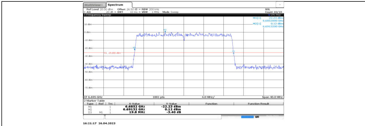
11BE20-CDD_Ant2_6695
