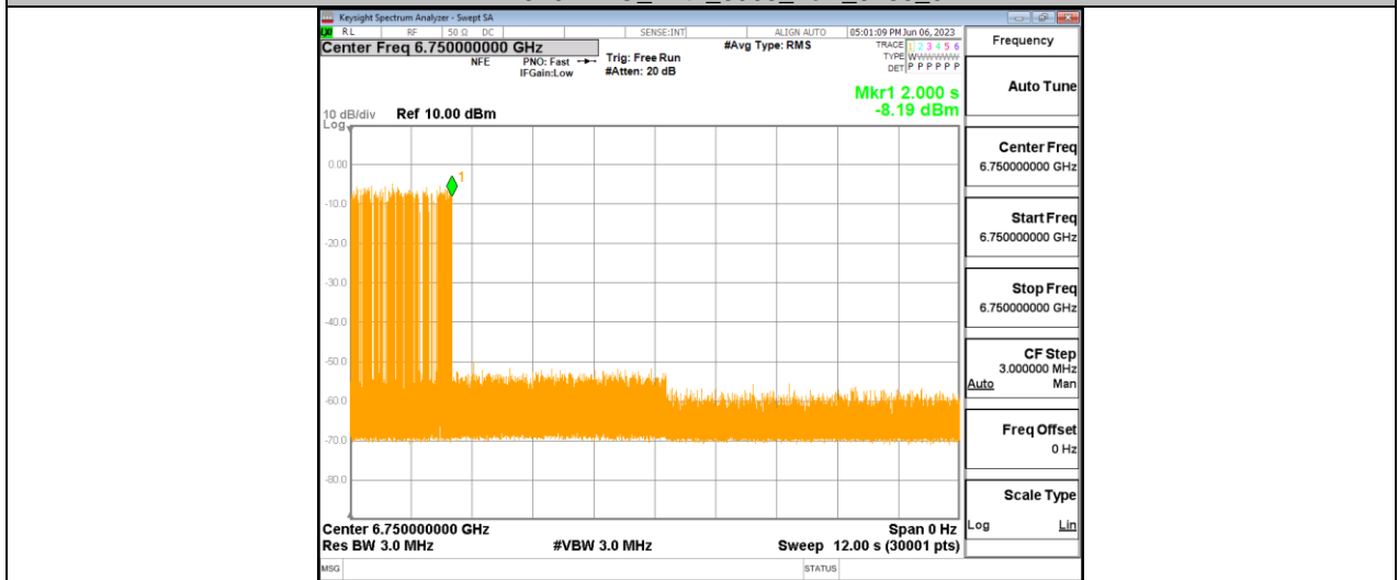
11BE320MIMO_Ant1_6905_Low_6750_6
