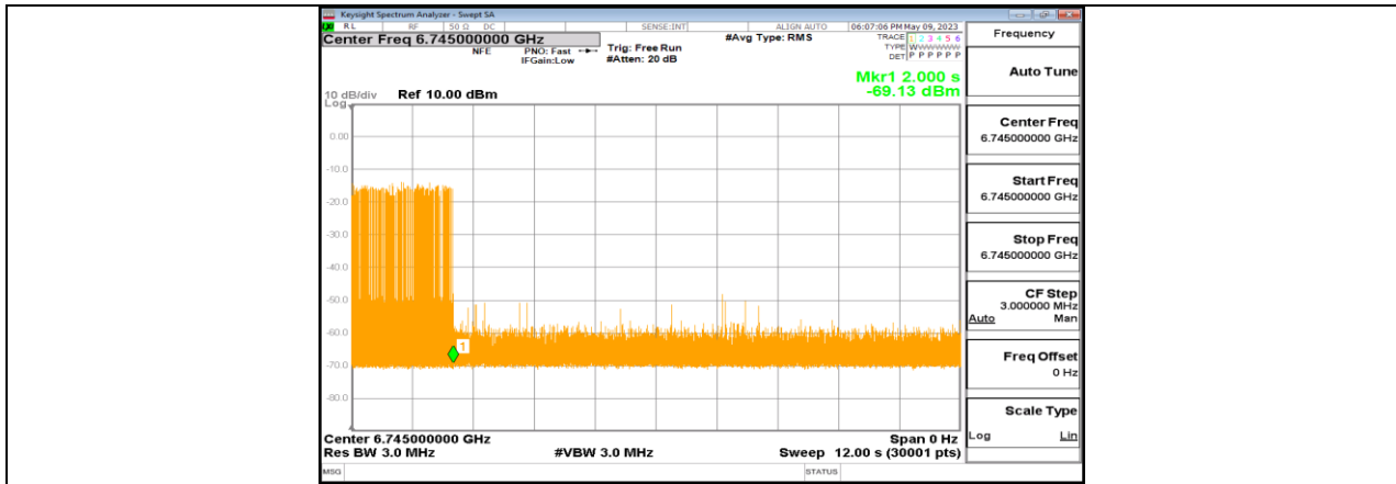
11BE320-CDD_Ant1_6745_Center_6745_1
