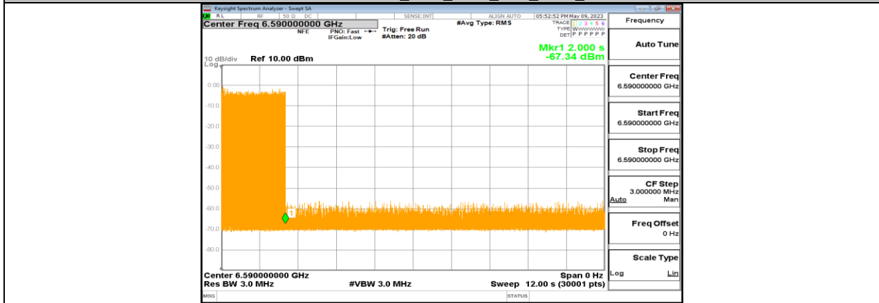
11BE320-CDD_Ant1_6745_Low_6590_3
