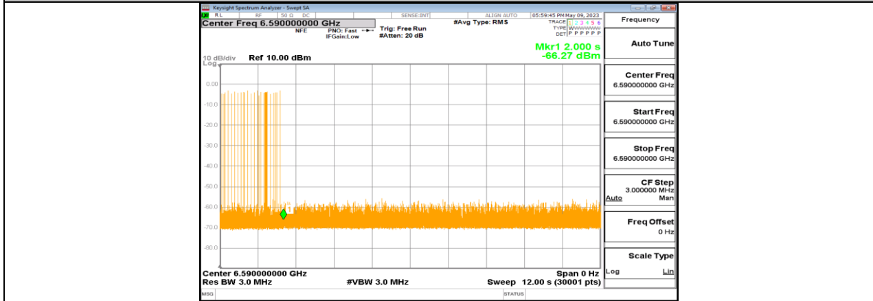
11BE320-CDD_Ant1_6745_Low_6590_7
