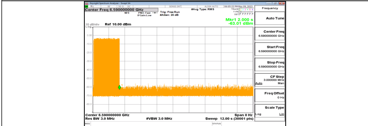
11BE320-CDD_Ant1_6745_Low_6590_10
