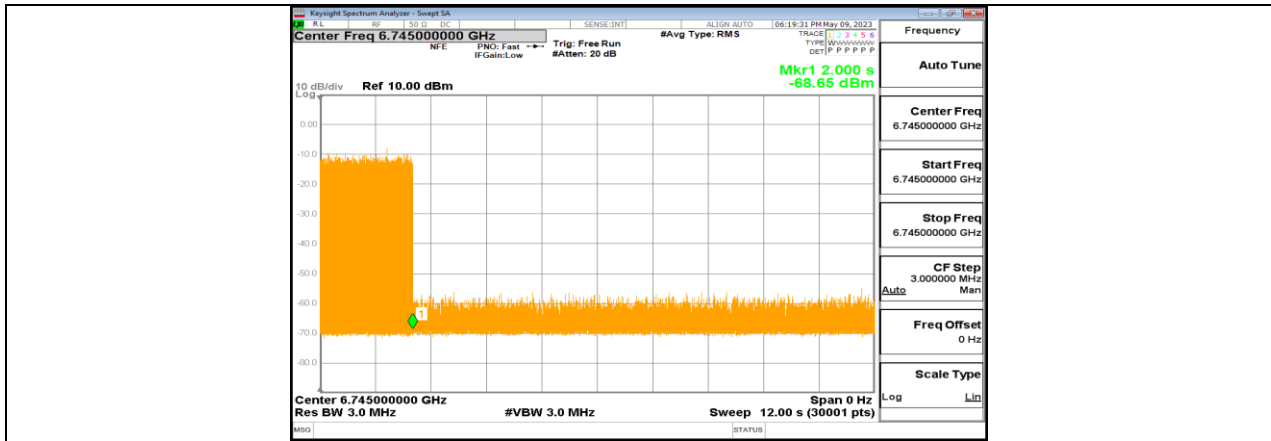
11BE320-CDD_Ant1_6745_Center_6745_7
