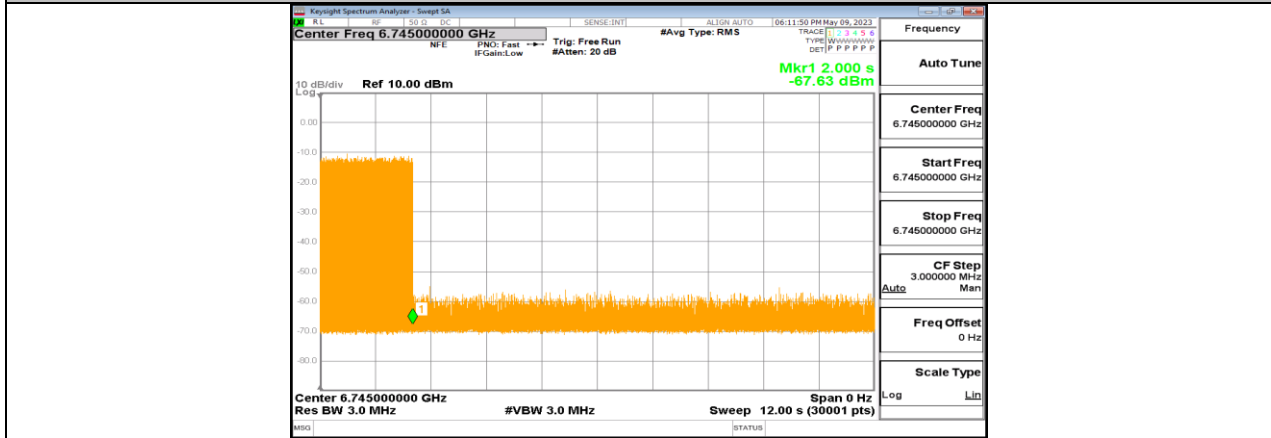
11BE320-CDD_Ant1_6745_Center_6745_3
