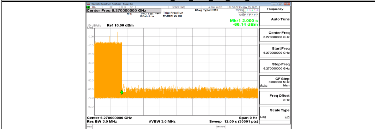
11BE320-CDD_Ant1_6425_Low_6270_10
