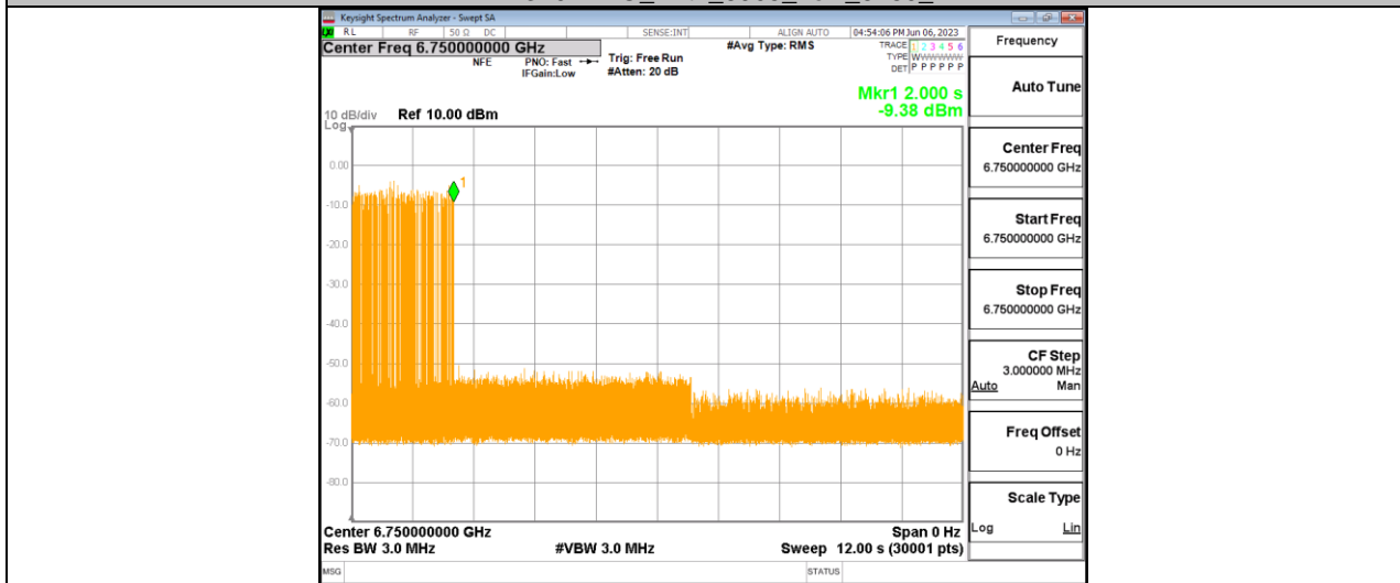
11BE320MIMO_Ant1_6905_Low_6750_3
