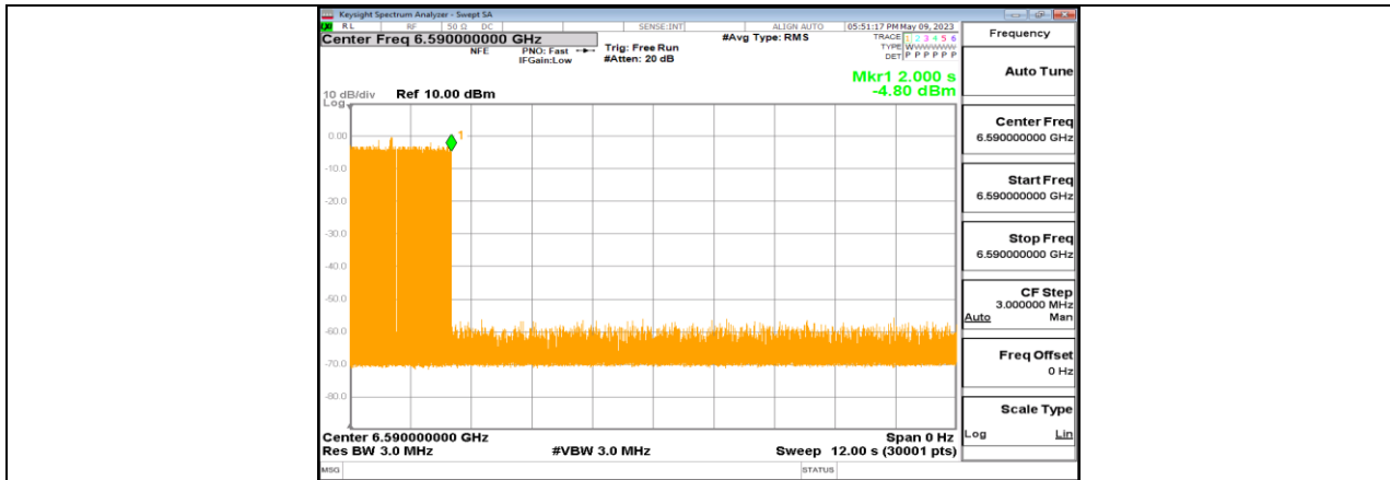
11BE320-CDD_Ant1_6745_Low_6590_2
