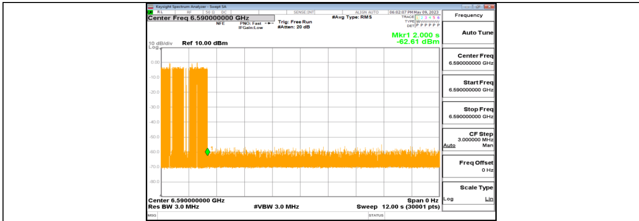
11BE320-CDD_Ant1_6745_Low_6590_8
