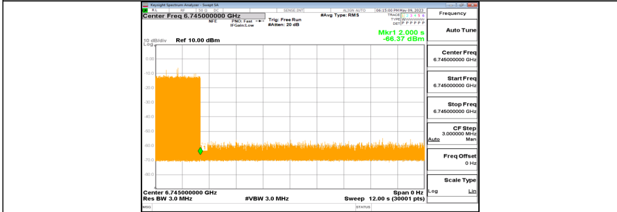
11BE320-CDD_Ant1_6745_Center_6745_5
