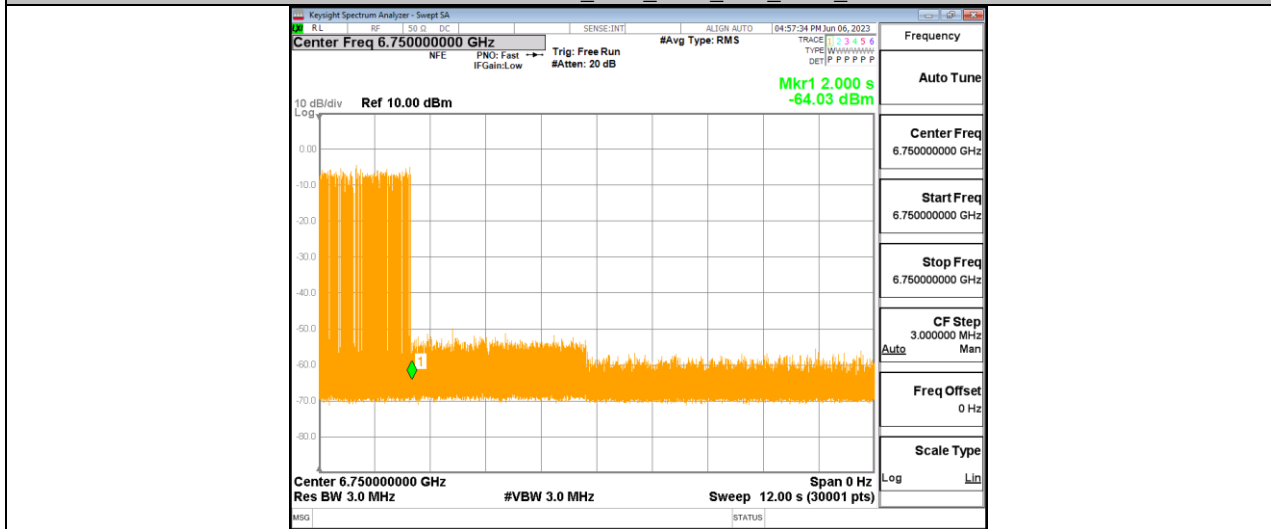
11BE320MIMO_Ant1_6905_Low_6750_4
