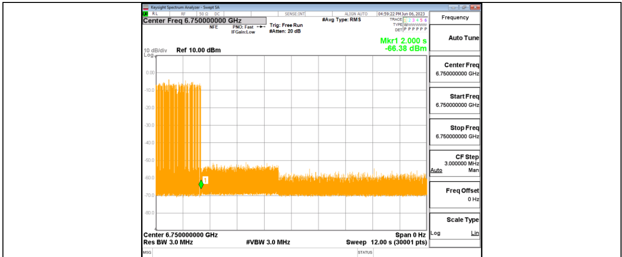
11BE320MIMO_Ant1_6905_Low_6750_5
