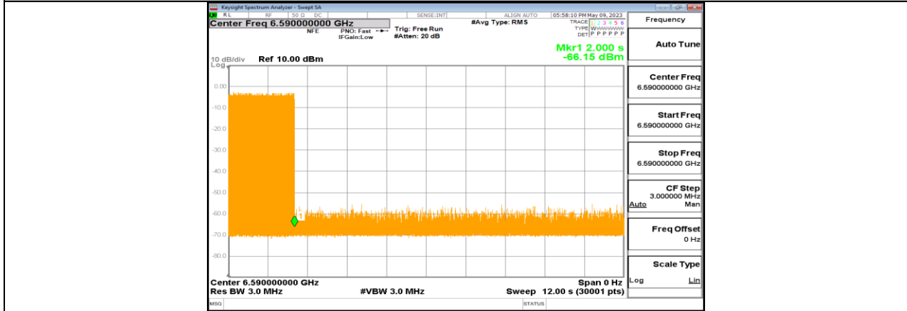
11BE320-CDD_Ant1_6745_Low_6590_6
