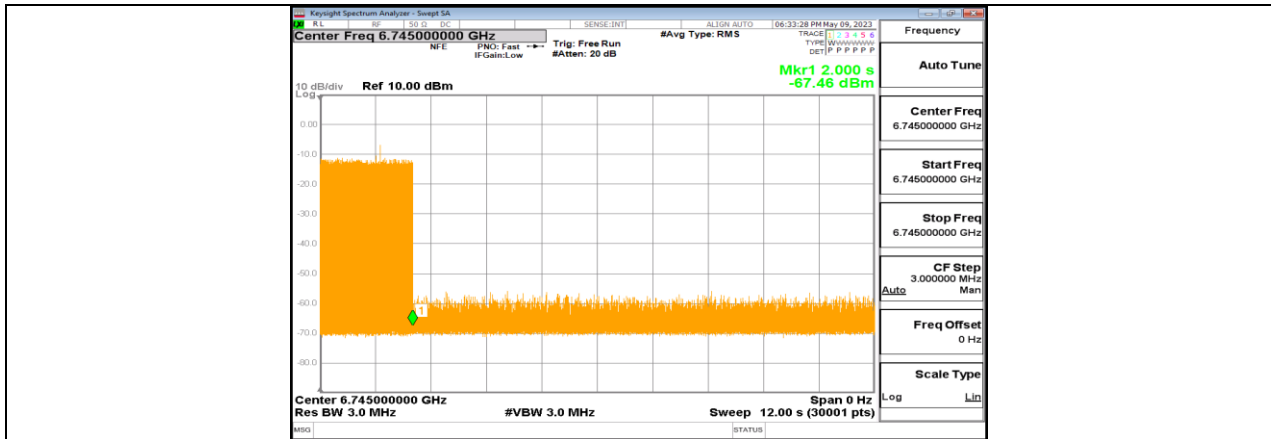
11BE320-CDD_Ant1_6745_Center_6745_10
