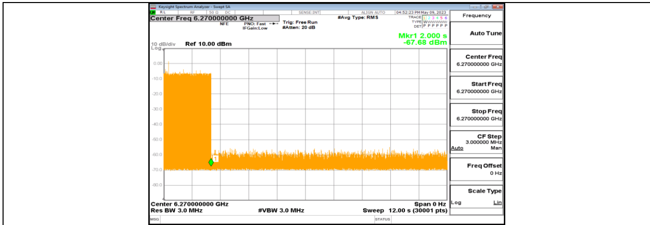
11BE320-CDD_Ant1_6425_Low_6270_8
