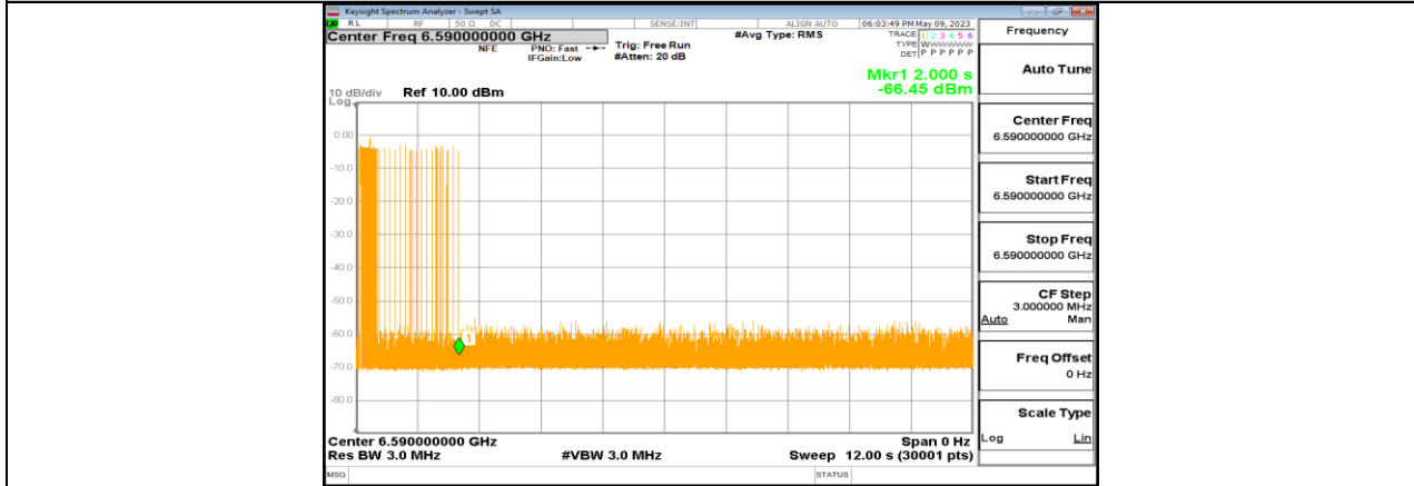
11BE320-CDD_Ant1_6745_Low_6590_9
