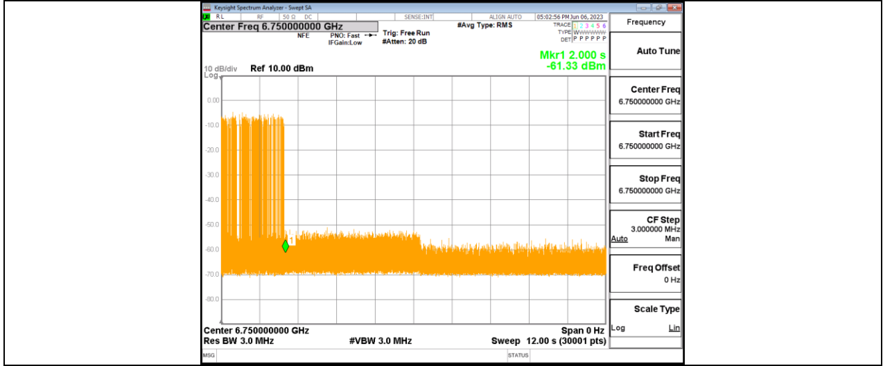
11BE320MIMO_Ant1_6905_Low_6750_7
