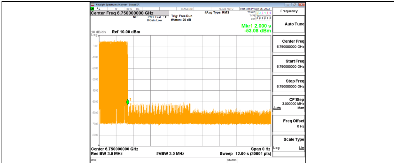
11BE320MIMO_Ant1_6905_Low_6750_2
