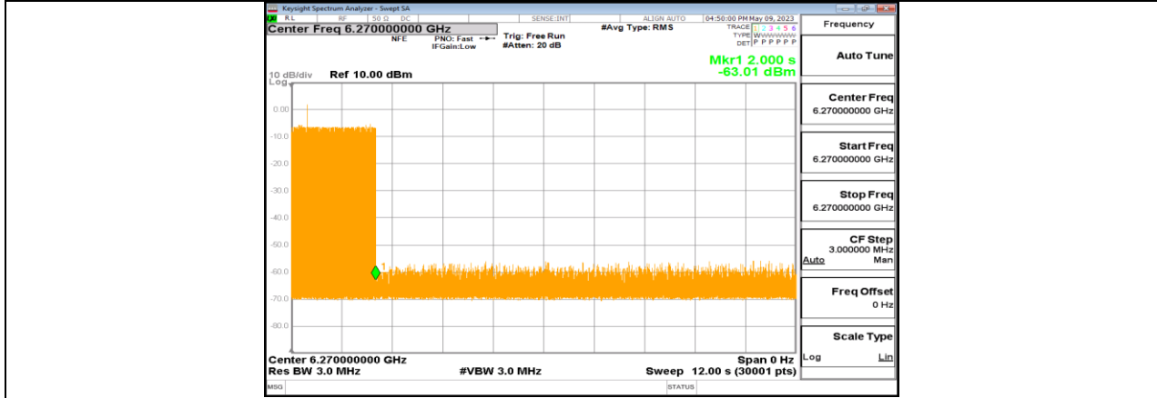
11BE320-CDD_Ant1_6425_Low_6270_7
