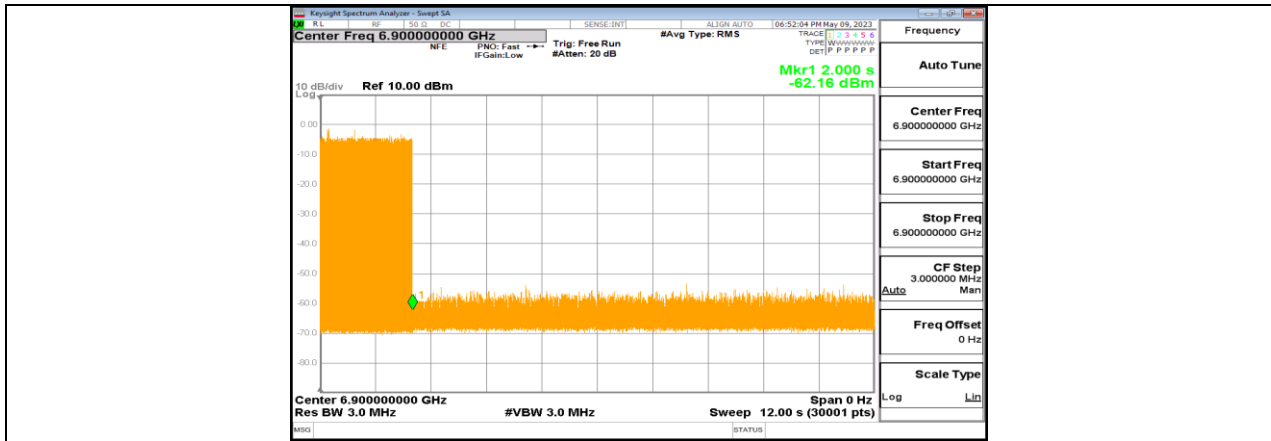
11BE320-CDD_Ant1_6745_High_6900_9
