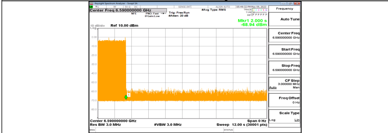
11BE320-CDD_Ant1_6745_Low_6590_1
