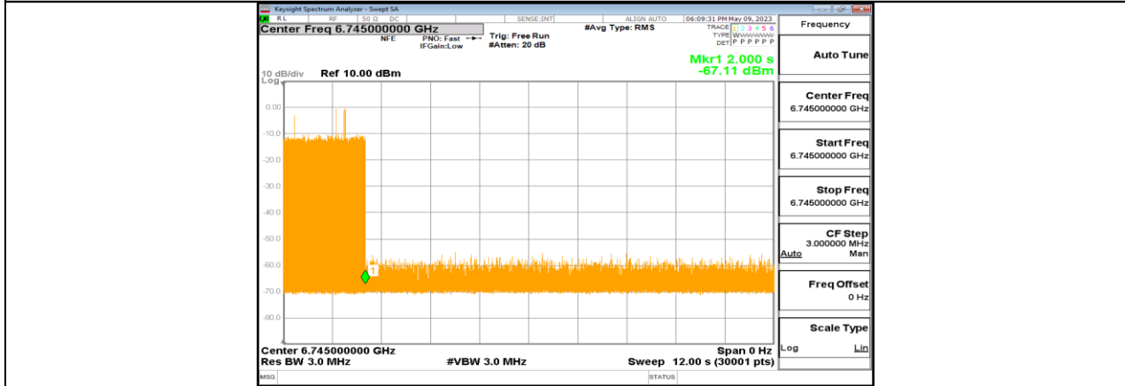
11BE320-CDD_Ant1_6745_Center_6745_2
