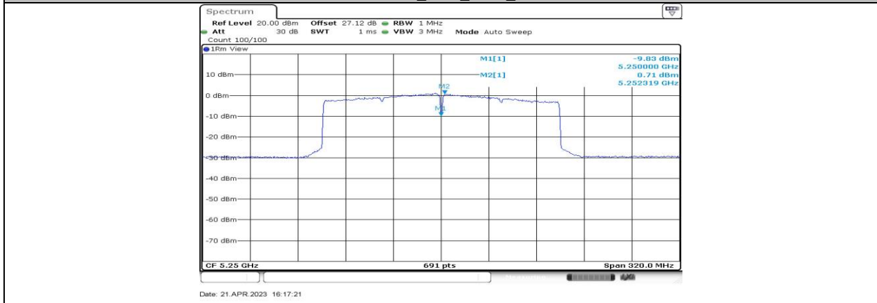
11AX160-CDD_Ant2_5250_UNII-2A
