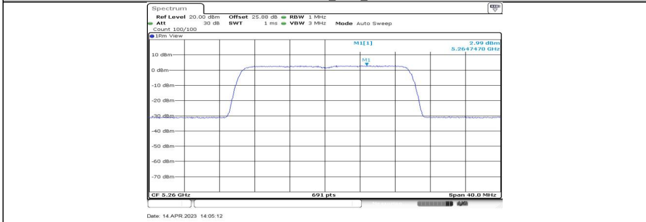
11BE20-CDD_Ant1_5260
