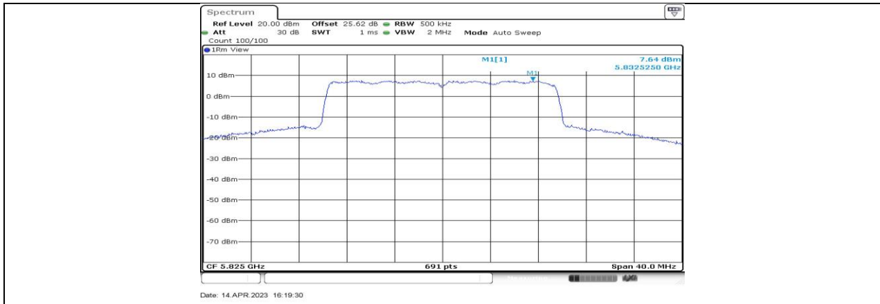
11BE20-CDD_Ant3_5825
