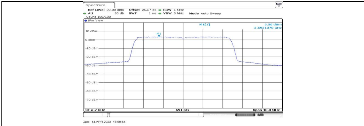
11BE20-CDD_Ant3_5700
