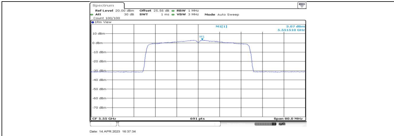
11BE40-CDD_Ant3_5550
