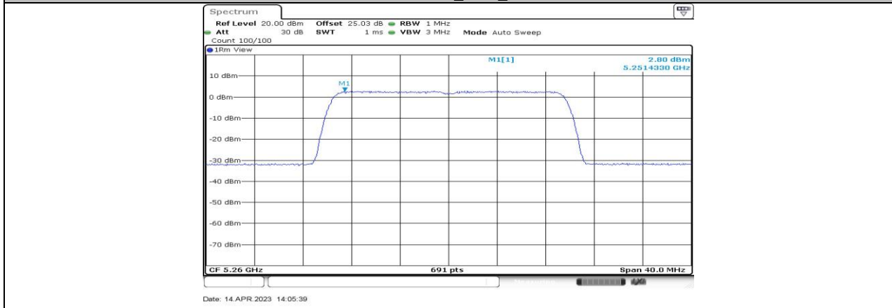
11BE20-CDD_Ant3_5260
