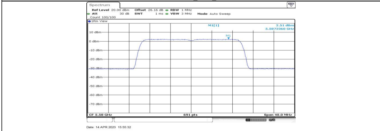
11BE20-CDD_Ant2_5580
