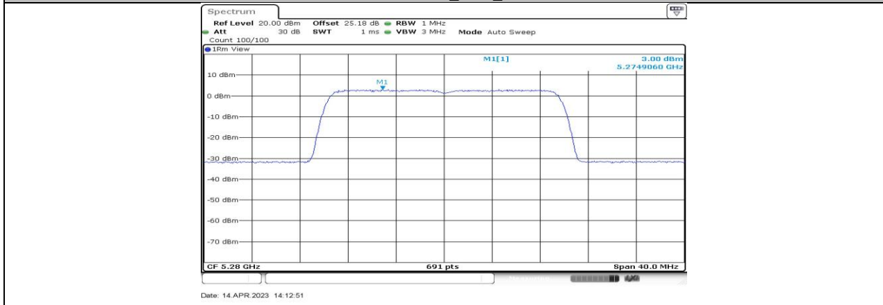
11BE20-CDD_Ant3_5280
