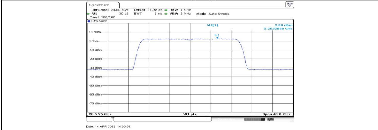
11BE20-CDD_Ant4_5260
