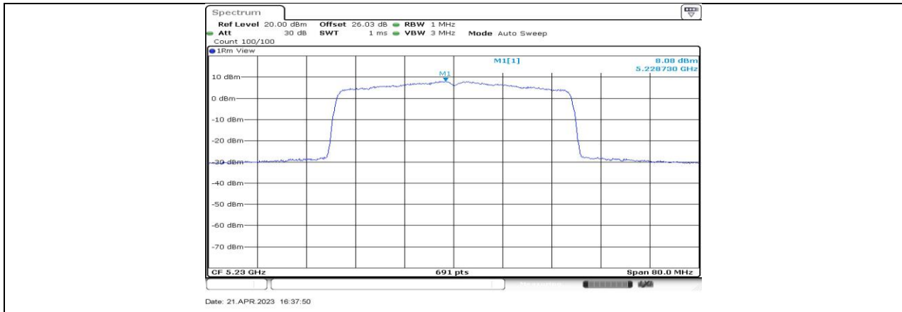
11BE40-CDD_Ant1_5230
