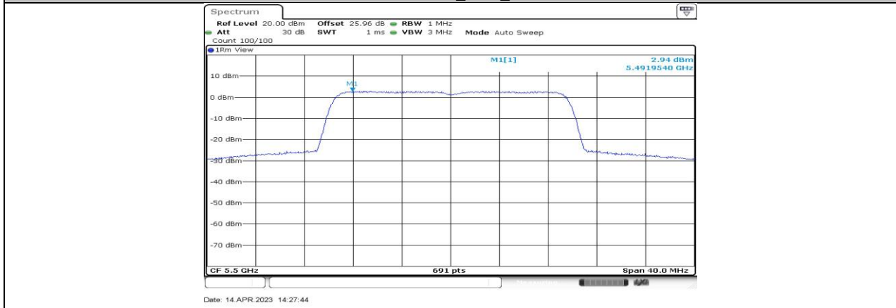
11BE20-CDD_Ant1_5500
