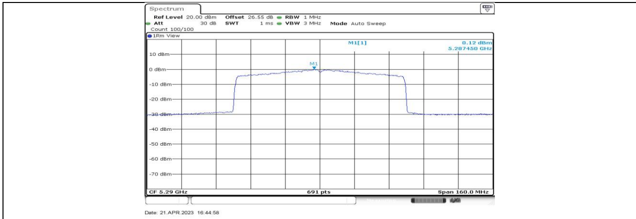
11BE80-CDD_Ant1_5290
