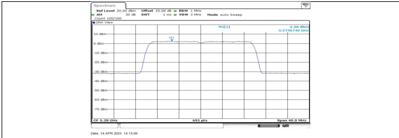
11BE20-CDD_Ant4_5280
