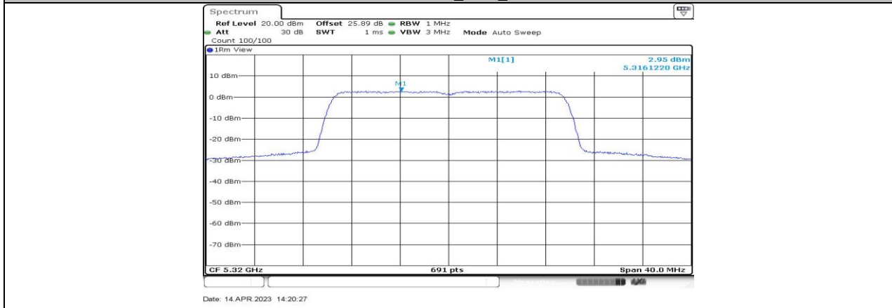
11BE20-CDD_Ant1_5320
