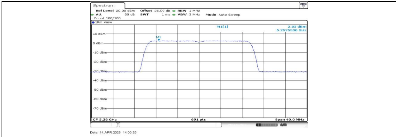
11BE20-CDD_Ant2_5260
