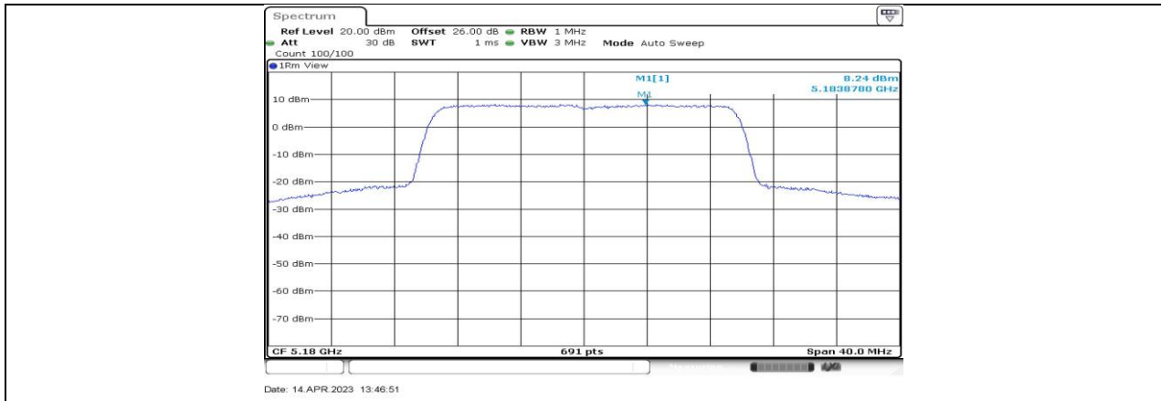
11BE20-CDD_Ant2_5180
