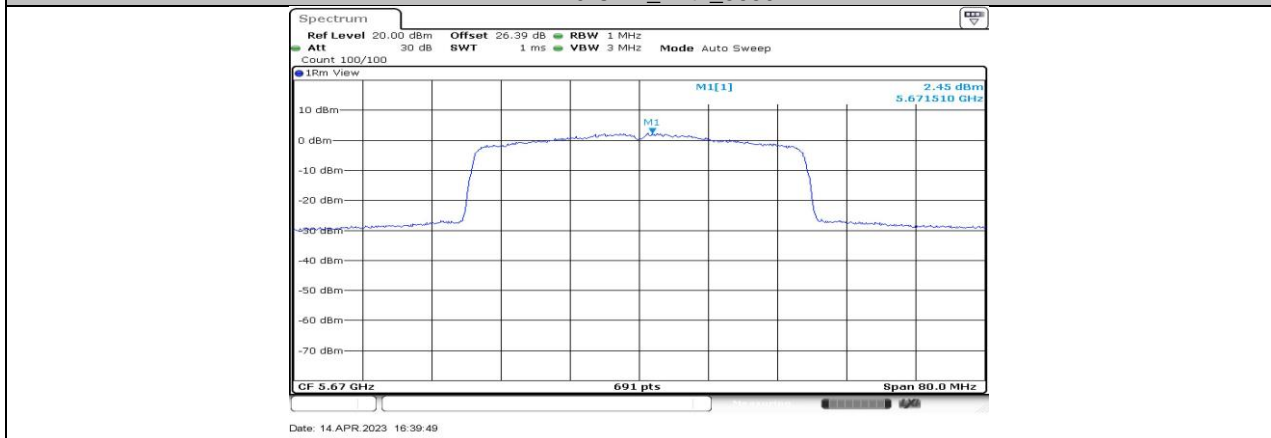
11BE40-CDD_Ant1_5670
