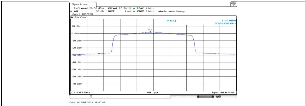
11BE40-CDD_Ant2_5670
