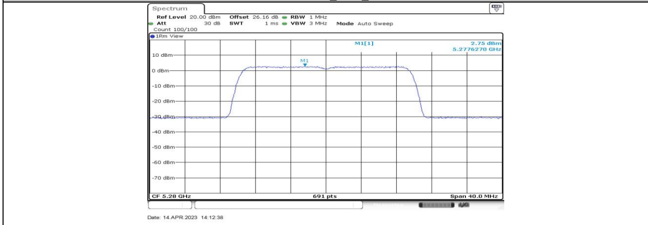
11BE20-CDD_Ant2_5280
