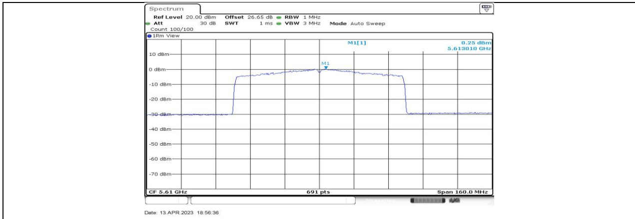
11AX80-CDD_Ant1_5610
