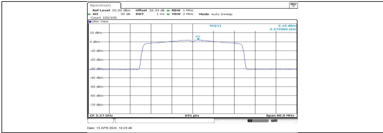
11AX40-CDD_Ant2_5270
