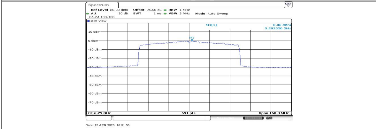
11AX80-CDD_Ant1_5290
