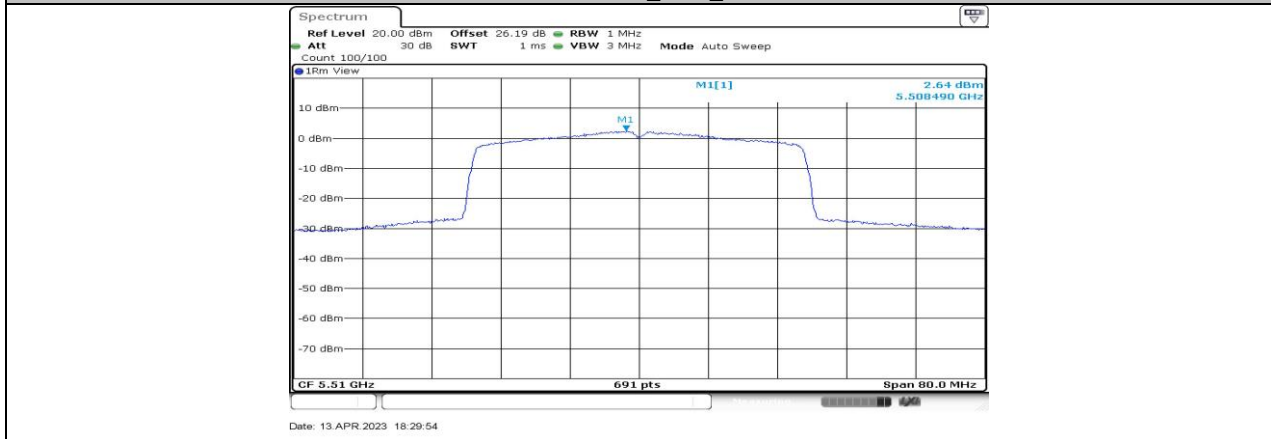
11AX40-CDD_Ant1_5510
