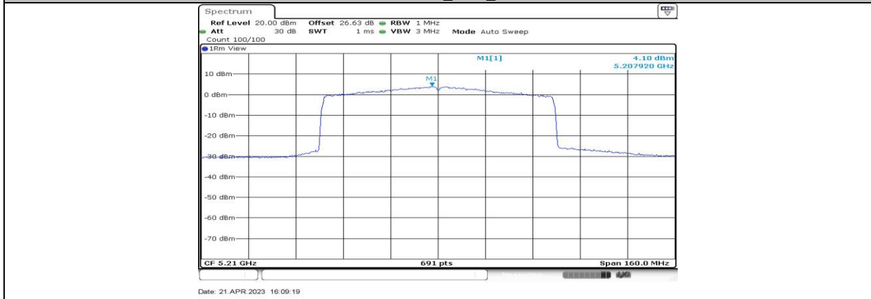
11AX80-CDD_Ant2_5210
