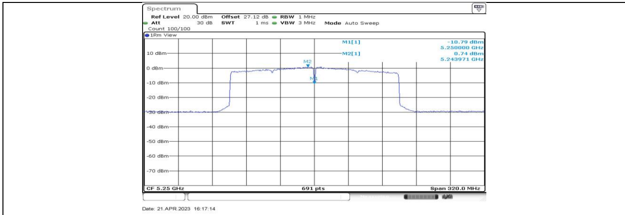
11AX160-CDD_Ant2_5250_UNII-1
