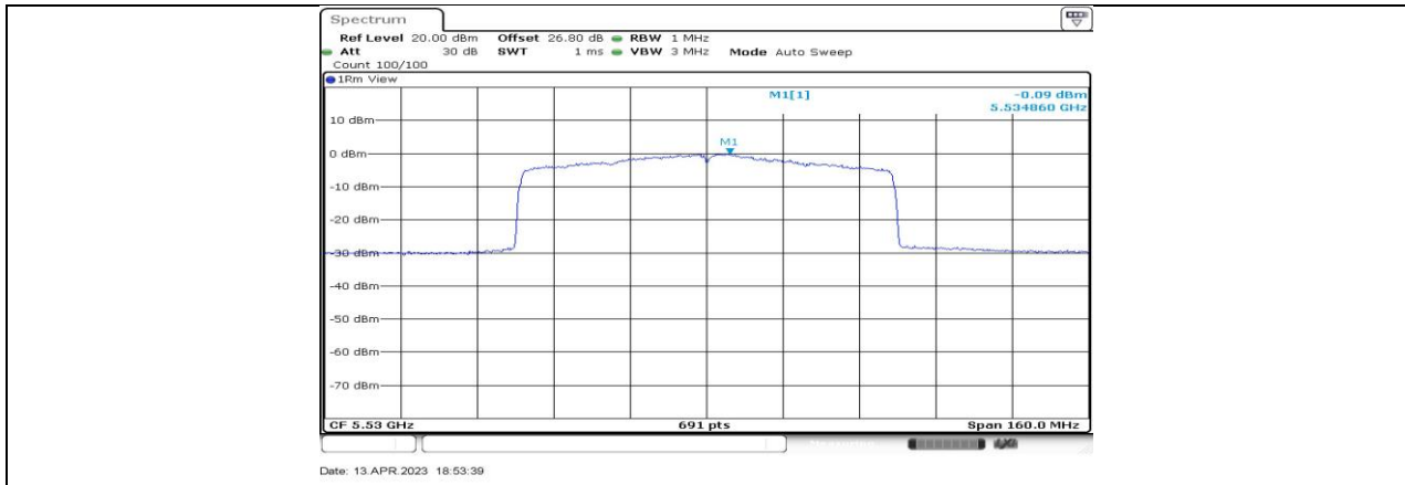
11AX80-CDD_Ant2_5530
