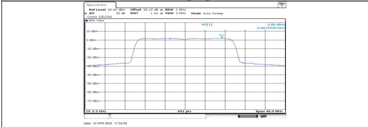
11AX20-CDD_Ant2_5500
