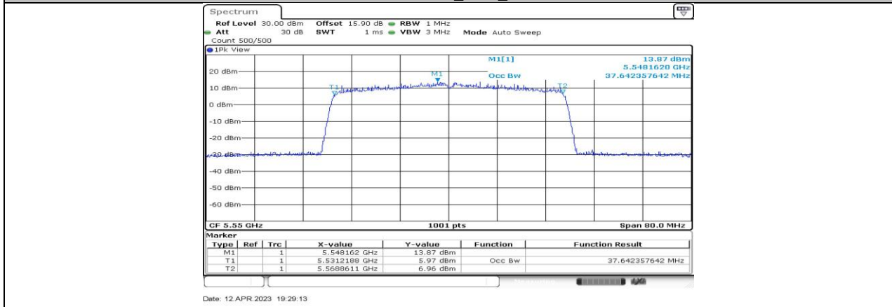
11AX40-CDD_Ant1_5550
