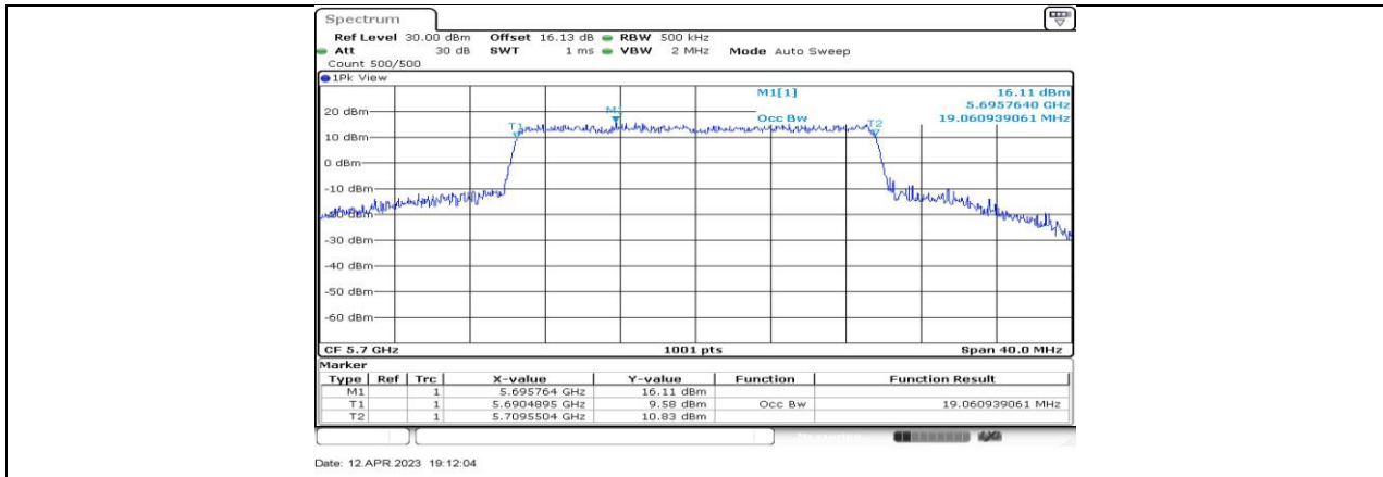
11AX20-CDD_Ant2_5700
