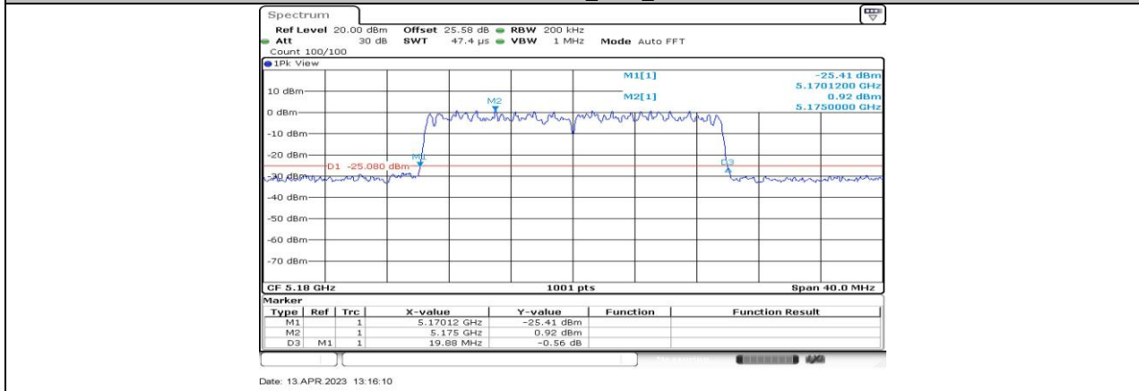
11BE20-CDD_Ant1_5180
