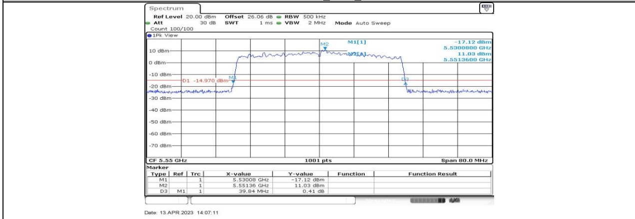
11BE40-CDD_Ant2_5550
