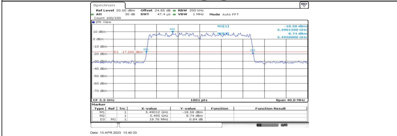
11BE20-CDD_Ant4_5500
