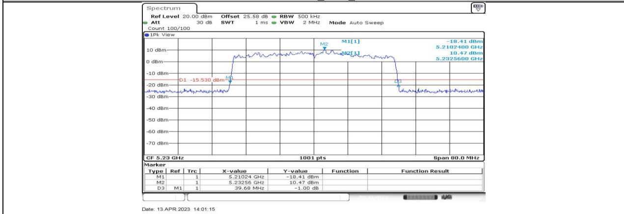
11BE40-CDD_Ant1_5230
