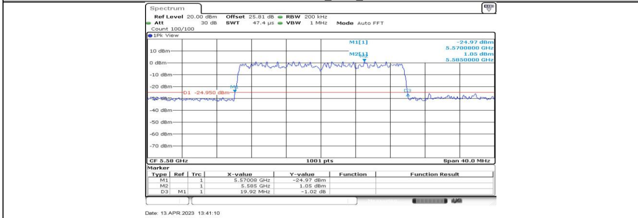
11BE20-CDD_Ant1_5580
