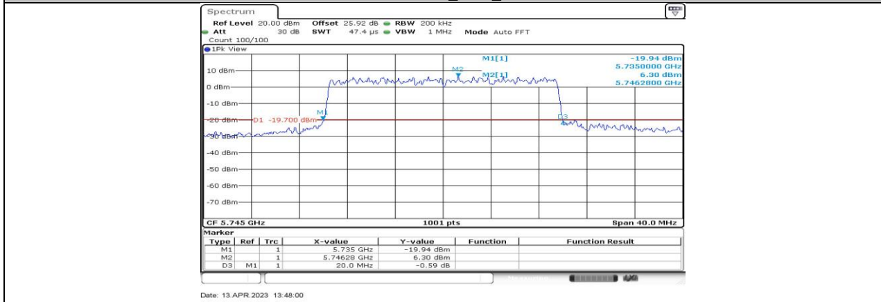
11BE20-CDD_Ant2_5745
