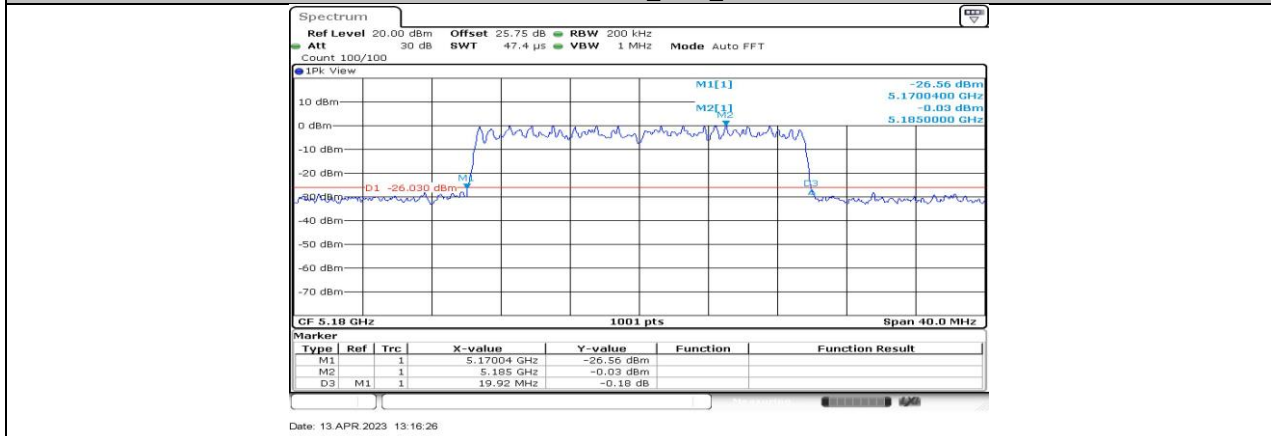
11BE20-CDD_Ant2_5180
