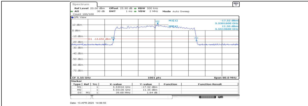
11BE40-CDD_Ant1_5550
