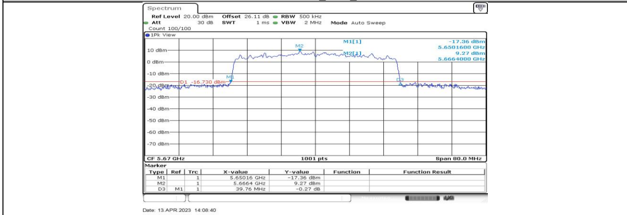
11BE40-CDD_Ant2_5670
