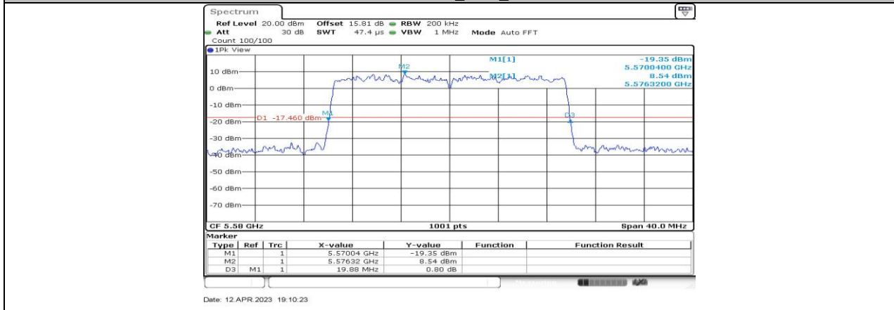
11AX20-CDD_Ant1_5580
