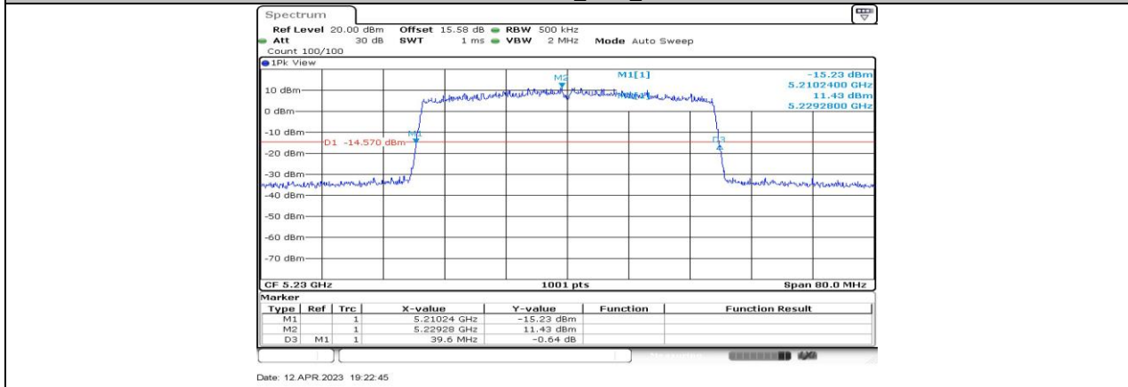
11AX40-CDD_Ant1_5230
