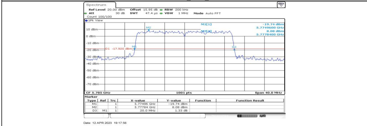
11AX20-CDD_Ant1_5785
