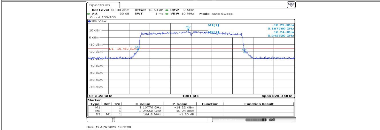
11AX160-CDD_Ant1_5250
