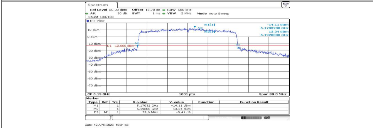
11AX40-CDD_Ant2_5190
