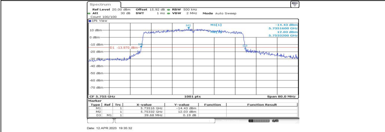
11AX40-CDD_Ant1_5755
