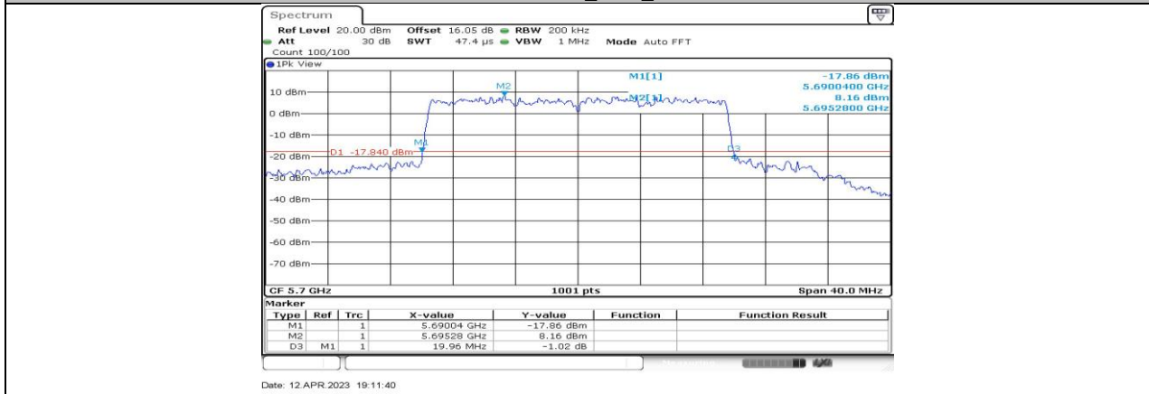
11AX20-CDD_Ant1_5700
