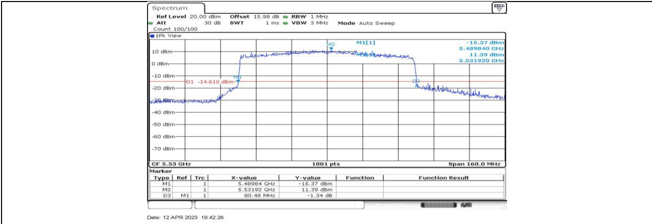
11AX80-CDD_Ant2_5530
