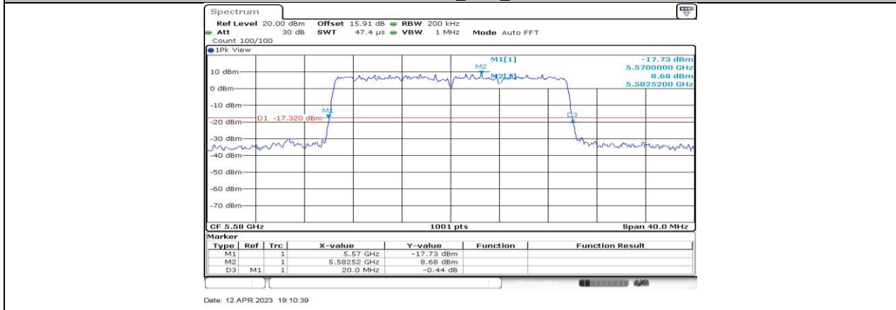
11AX20-CDD_Ant2_5580
