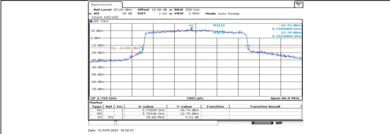
11AX40-CDD_Ant2_5755
