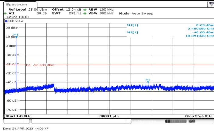
11BE20-CDD_Ant1_2412_1000~26500
