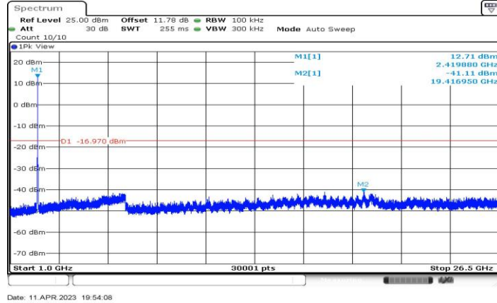
11BE20-CDD_Ant3_2417_1000~26500
