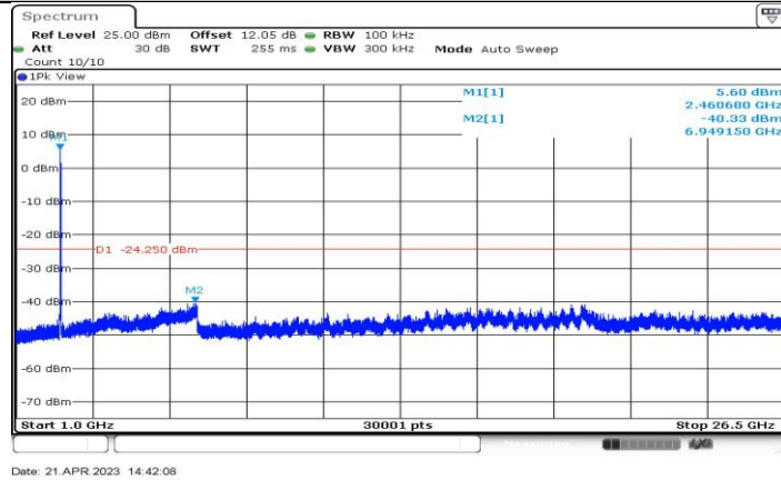
11BE20-CDD_Ant1_2462_1000~26500
