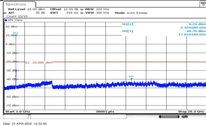
11BE20-CDD_Ant1_2457_1000~26500
