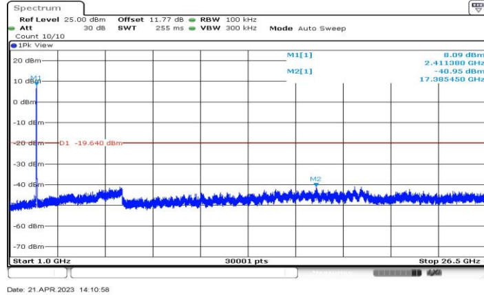
11BE20-CDD_Ant4_2412_1000~26500
