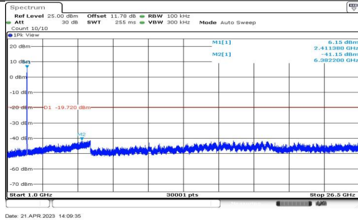
11BE20-CDD_Ant3_2412_1000~26500
