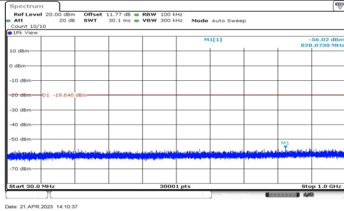
11BE20-CDD_Ant4_2412_30~1000
