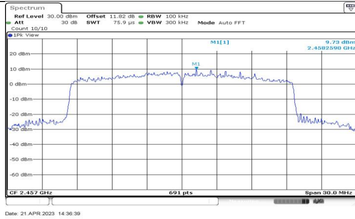
11BE20-CDD_Ant4_2457_0~Reference
