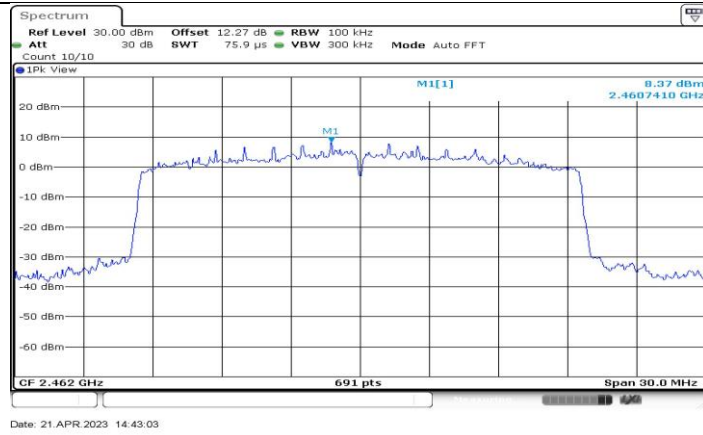
11BE20-CDD_Ant2_2462_0~Reference
