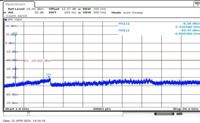
11BE20-CDD_Ant2_2457_1000~26500
