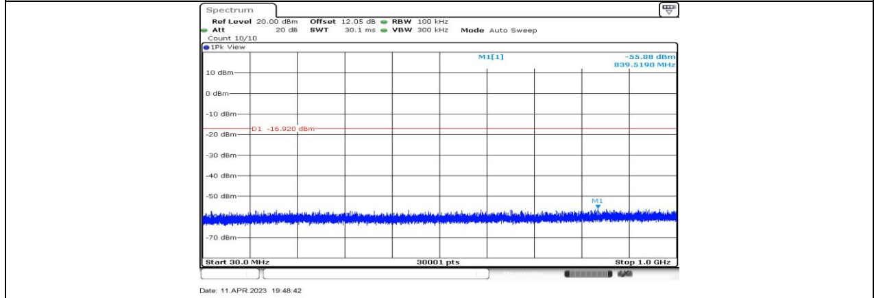
11BE20-CDD_Ant1_2417_30~1000
