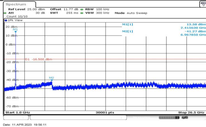
11BE20-CDD_Ant4_2417_1000~26500
