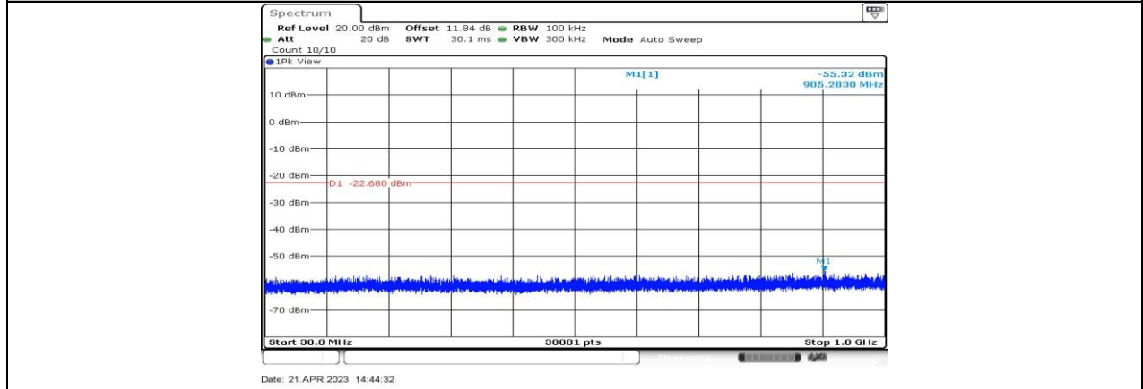
11BE20-CDD_Ant3_2462_30~1000
