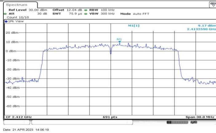
11BE20-CDD_Ant1_2412_0~Reference
