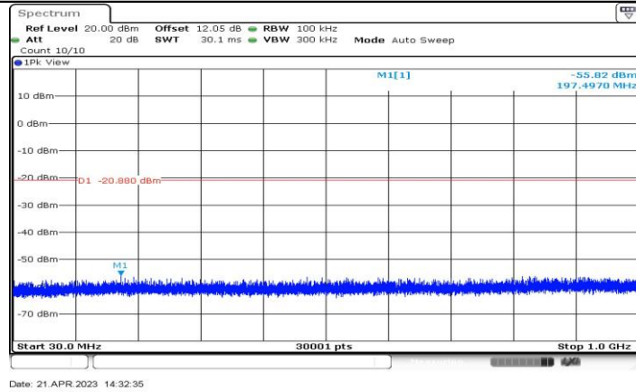
11BE20-CDD_Ant1_2457_30~1000
