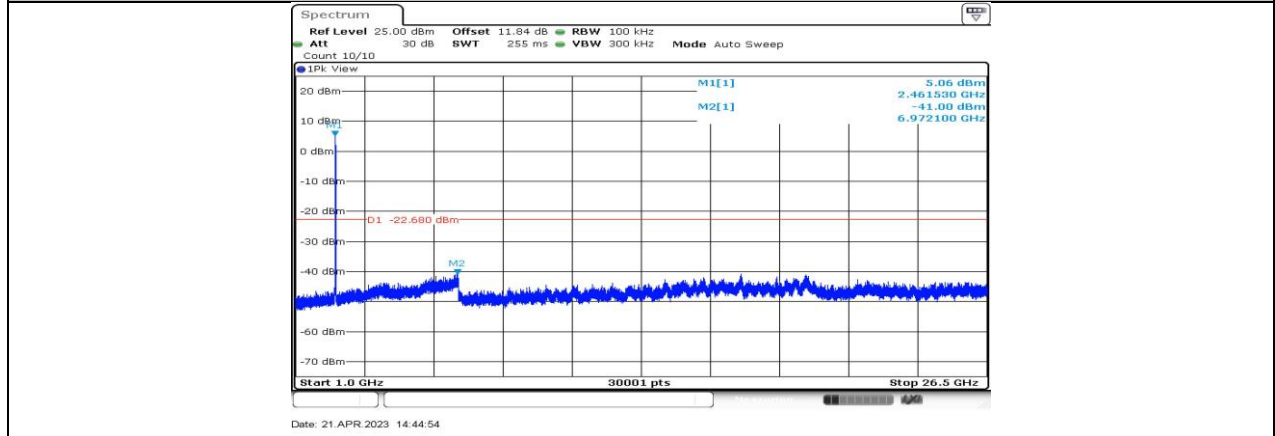
11BE20-CDD_Ant3_2462_1000~26500
