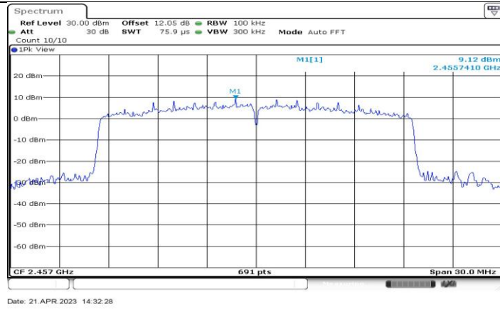
11BE20-CDD_Ant1_2457_0~Reference
