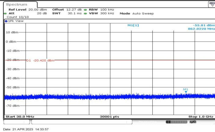
11BE20-CDD_Ant2_2457_30~1000
