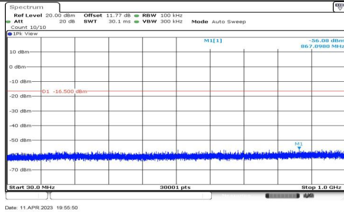
11BE20-CDD_Ant4_2417_30~1000
