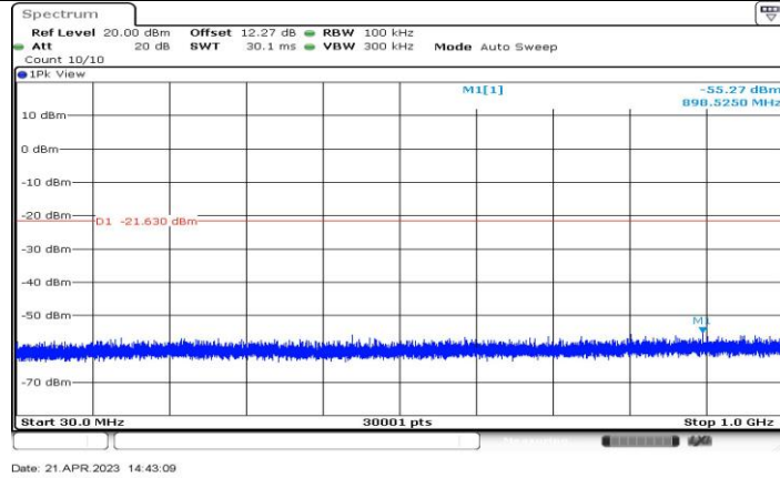
11BE20-CDD_Ant2_2462_30~1000
