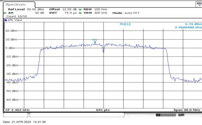
11BE20-CDD_Ant1_2462_0~Reference
