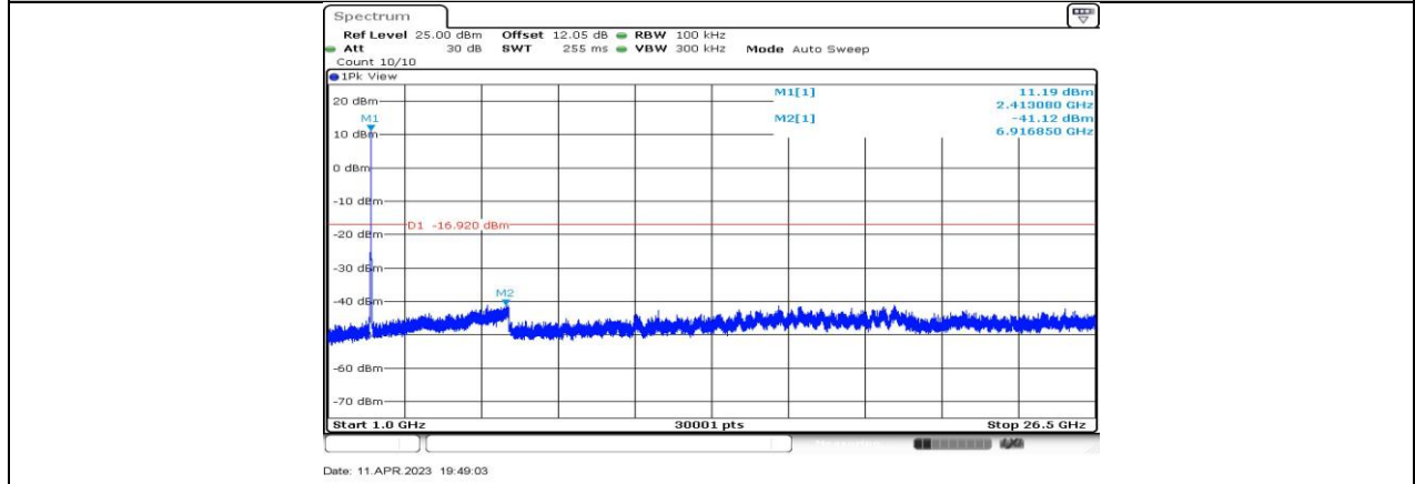
11BE20-CDD_Ant1_2417_1000~26500
