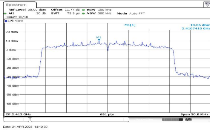
11BE20-CDD_Ant4_2412_0~Reference
