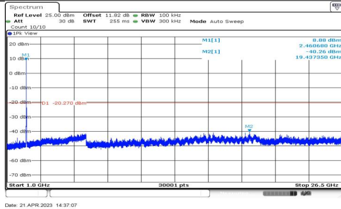
11BE20-CDD_Ant4_2457_1000~26500
