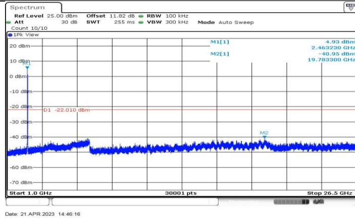
11BE20-CDD_Ant4_2462_1000~26500
