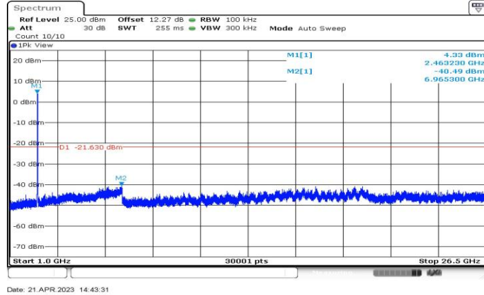
11BE20-CDD_Ant2_2462_1000~26500
