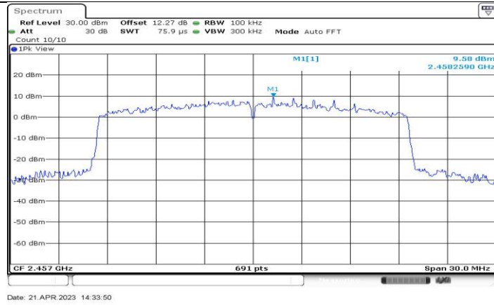
11BE20-CDD_Ant2_2457_0~Reference
