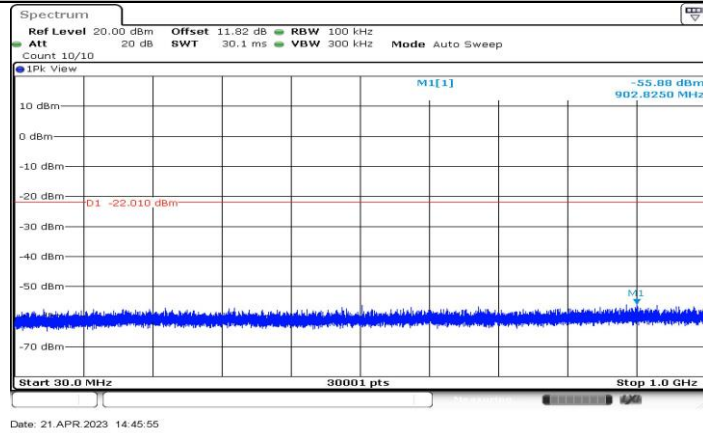
11BE20-CDD_Ant4_2462_30~1000
