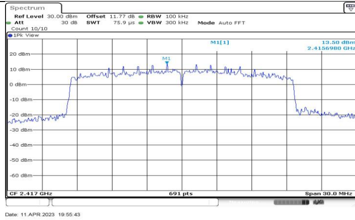
11BE20-CDD_Ant4_2417_0~Reference
