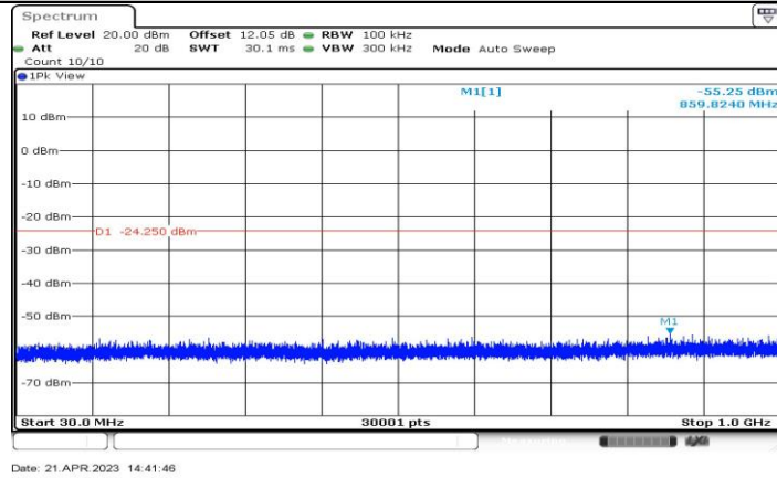
11BE20-CDD_Ant1_2462_30~1000
