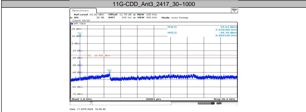
11G-CDD_Ant3_2417_1000~26500
