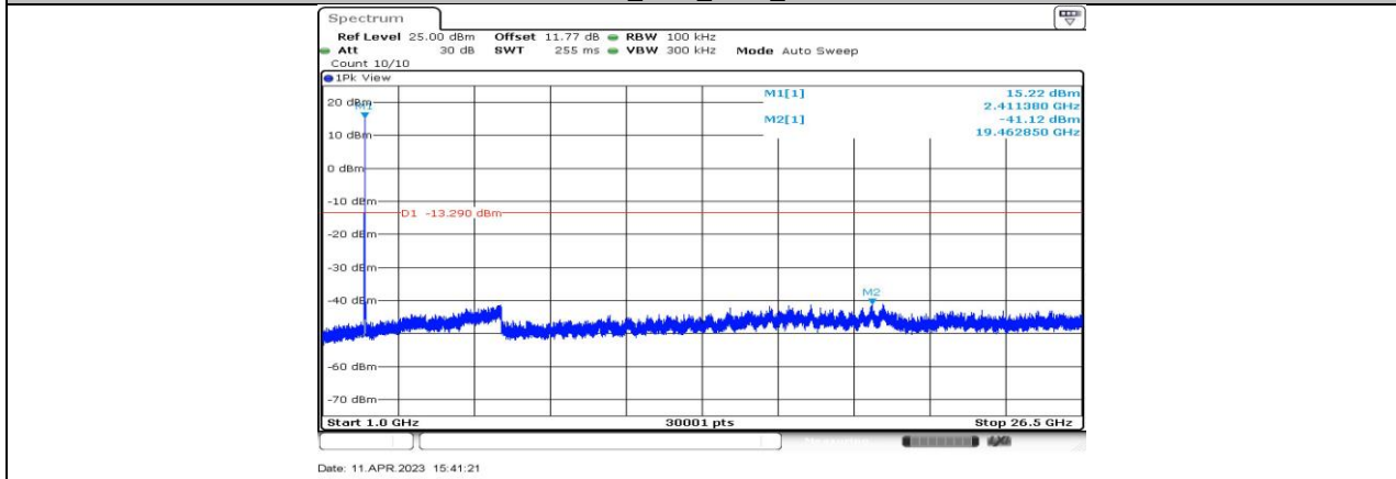
11B-CDD_Ant4_2412_1000~26500
