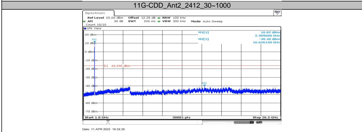
11G-CDD_Ant2_2412_1000~26500
