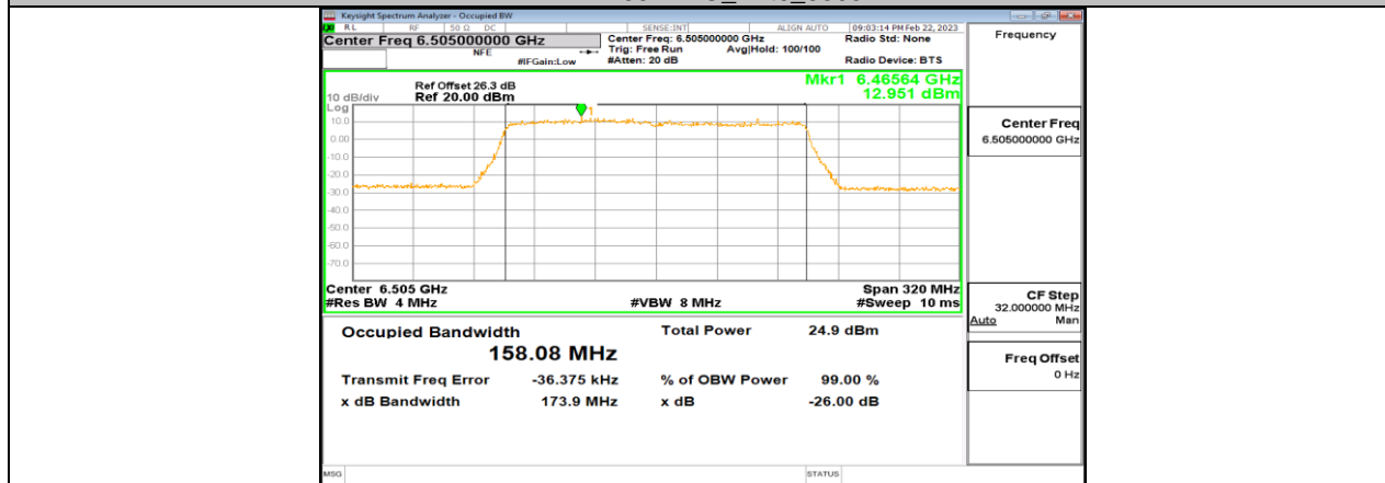
11AX160MIMO_Ant7_6505
