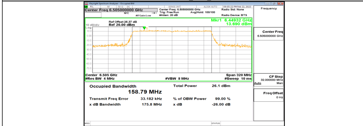
11AX160MIMO_Ant8_6505
