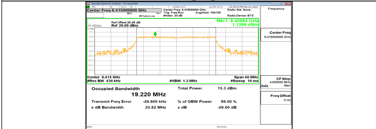
11BE20MIMO_Ant8_6415
