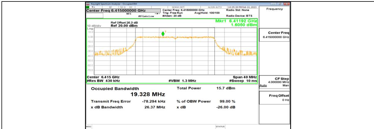
11BE20MIMO_Ant6_6415
