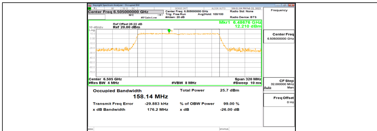
11AX160MIMO_Ant6_6505
