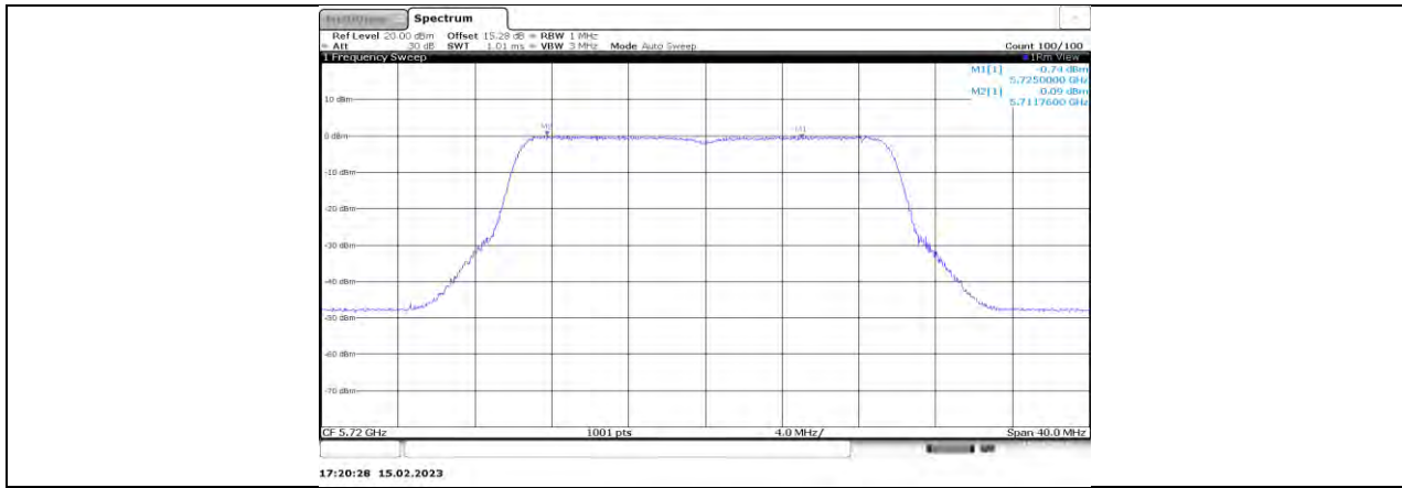
11AX20MIMO_Ant3_5720_UNII-2C
