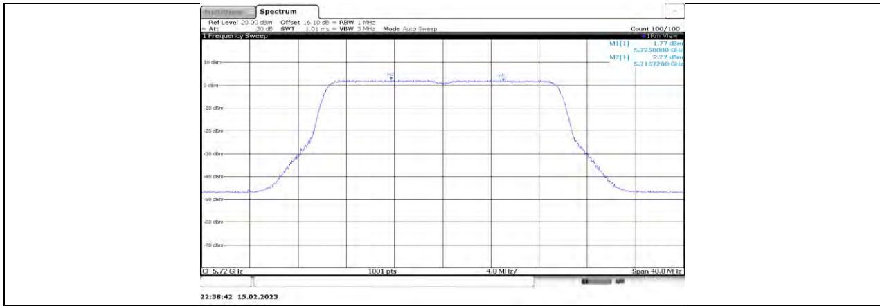
11BE20MIMO_Ant1_5720_UNII-2C
