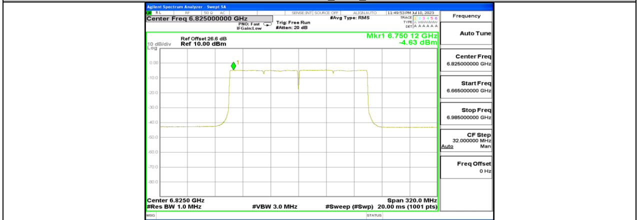
11BE160MIMO_Ant2_6825
