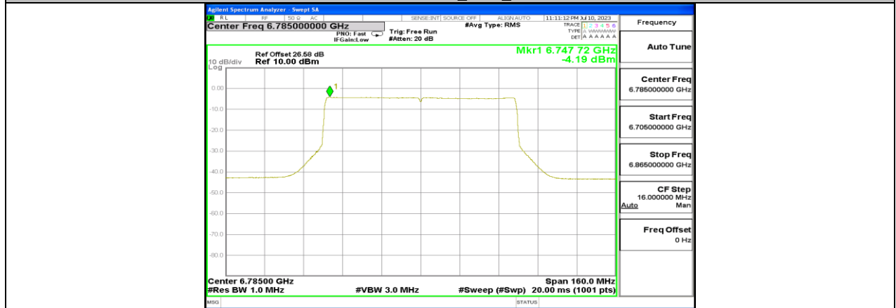
11BE80MIMO_Ant1_6785
