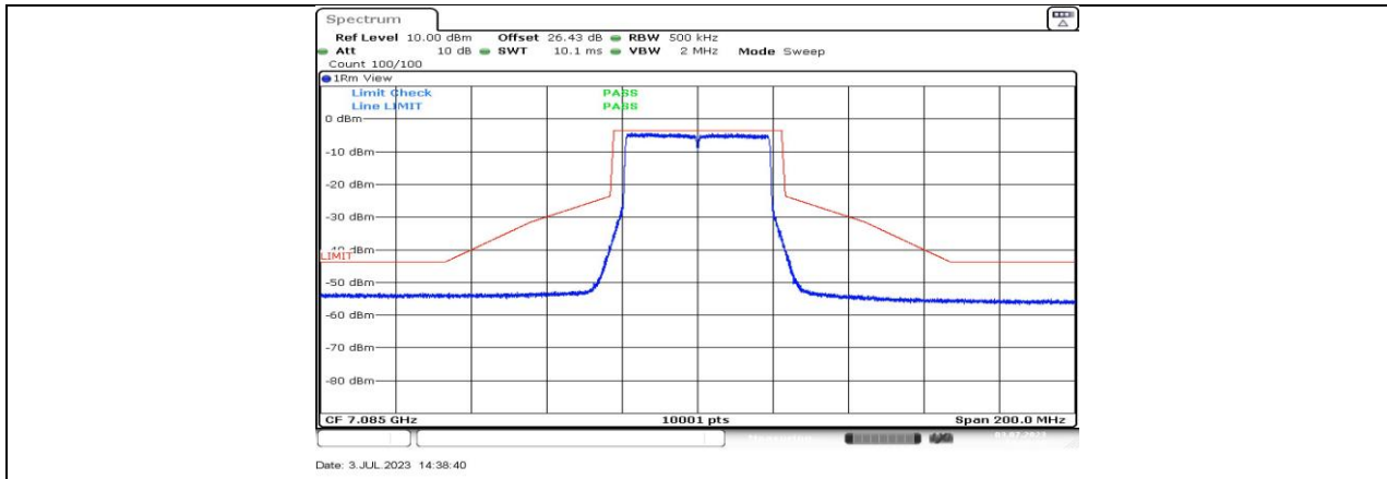
11BE40MIMO_Ant1_7085
