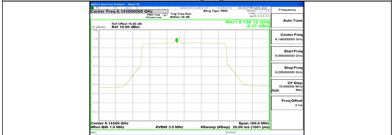
11BE80MIMO_Ant3_6145
