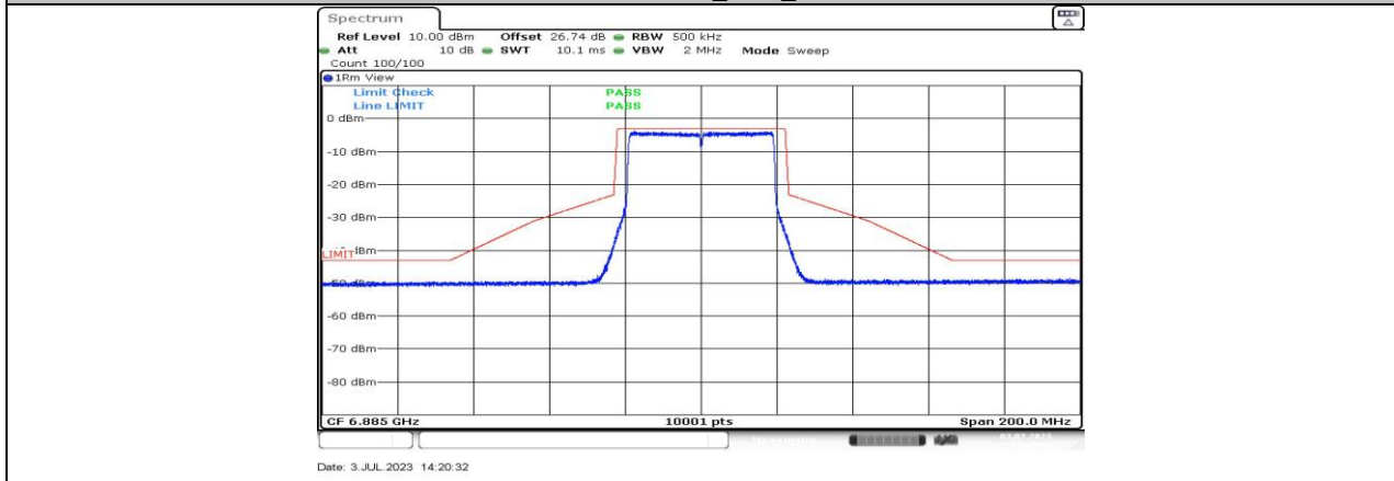
11BE40MIMO_Ant1_6885
