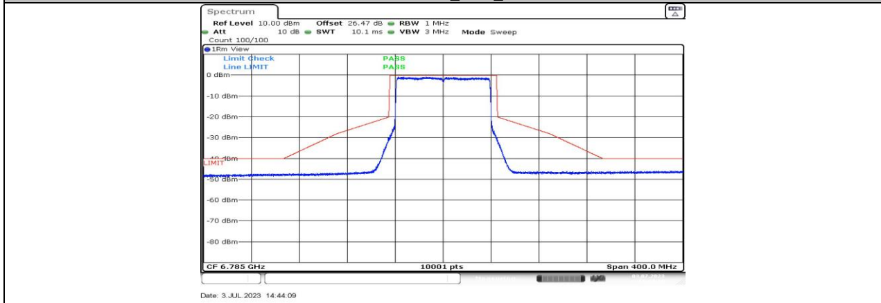
11BE80MIMO_Ant1_6785
