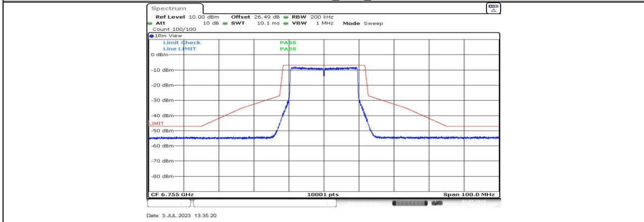
11BE20MIMO_Ant1_6755
