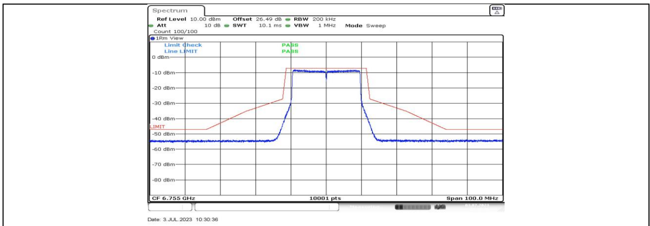
11AX20MIMO_Ant1_6755
