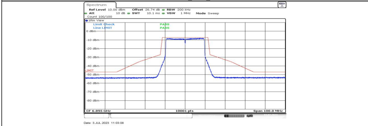
11AX20MIMO_Ant1_6895
