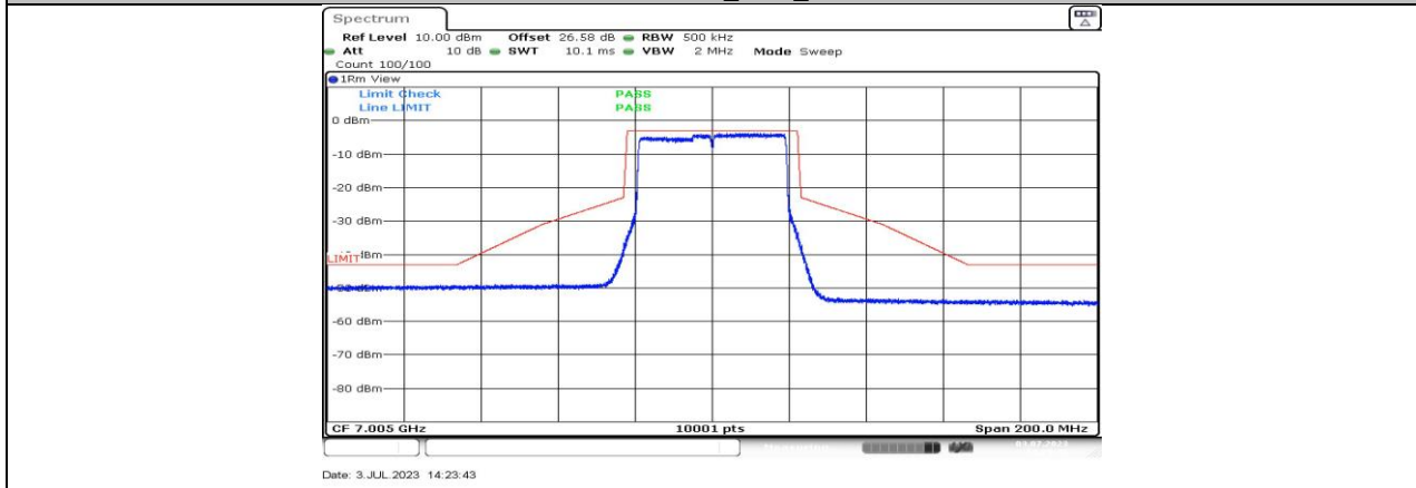
11BE40MIMO_Ant1_7005
