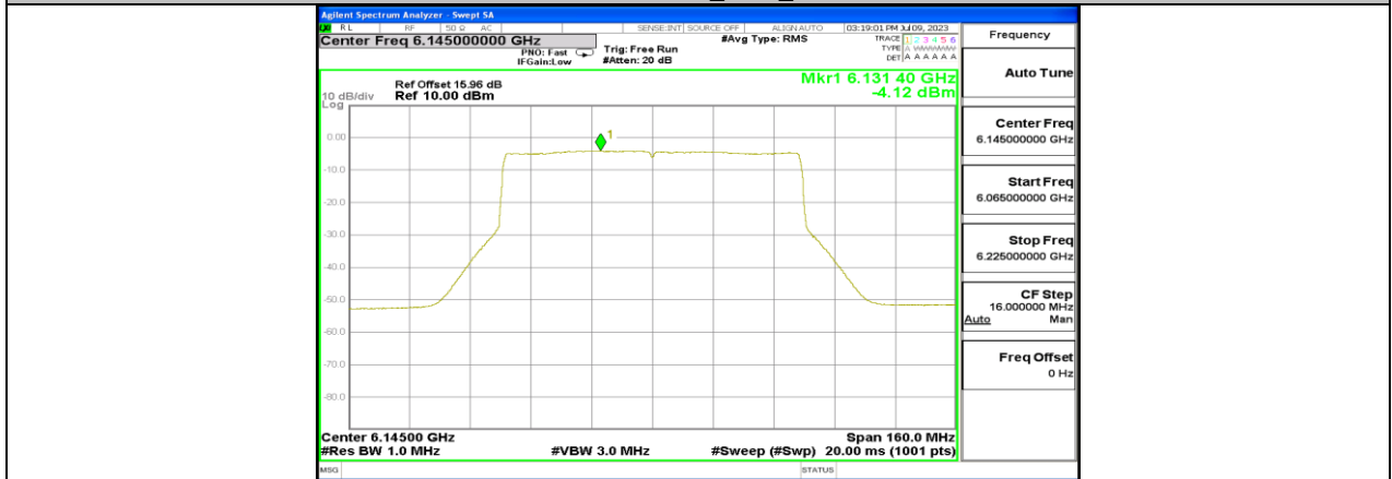
11AX80MIMO_Ant4_6145
