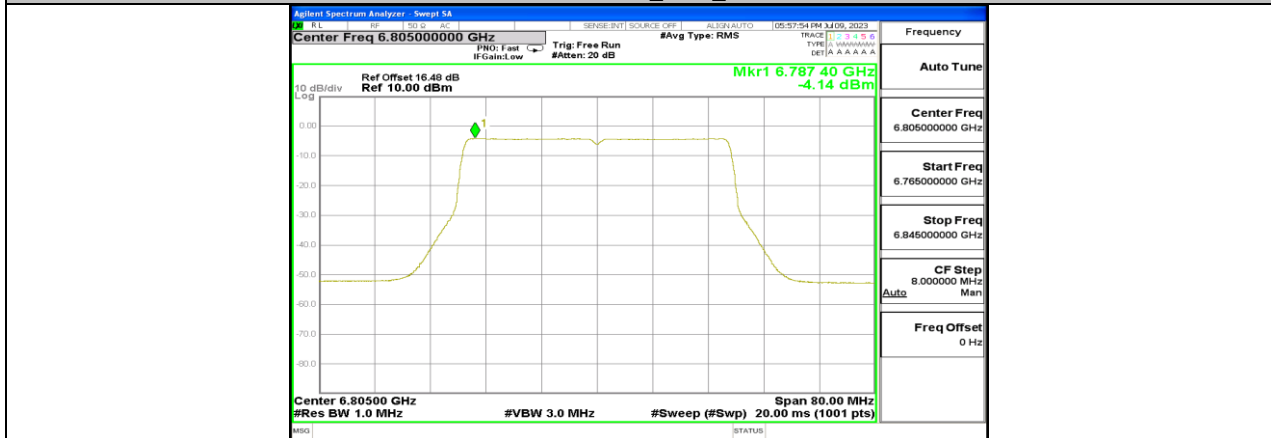
11AX40MIMO_Ant1_6805
