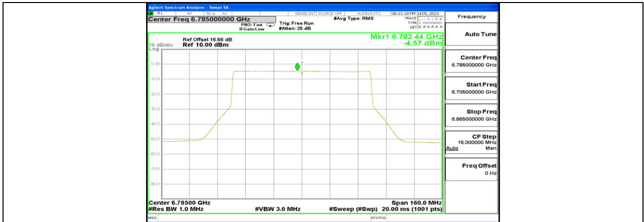
11AX80MIMO_Ant1_6785
