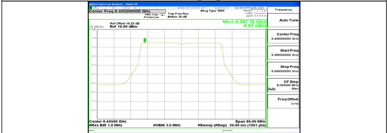
11AX40MIMO_Ant3_6405
