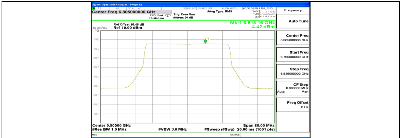
11AX40MIMO_Ant2_6805
