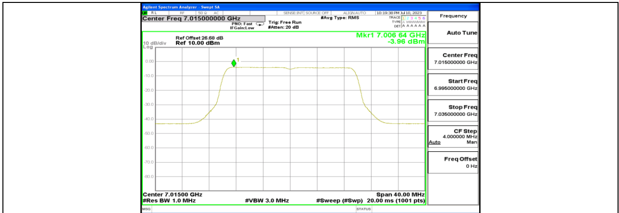
11BE20MIMO_Ant1_7015
