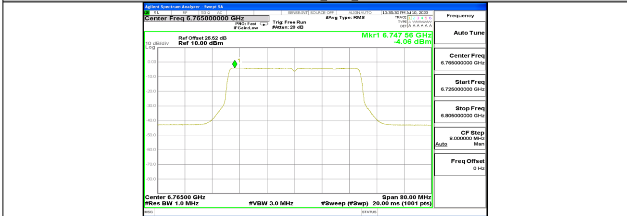
11BE40MIMO_Ant1_6765
