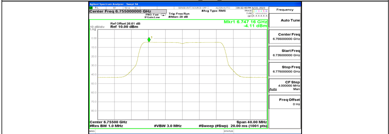
11BE20MIMO_Ant2_6755
