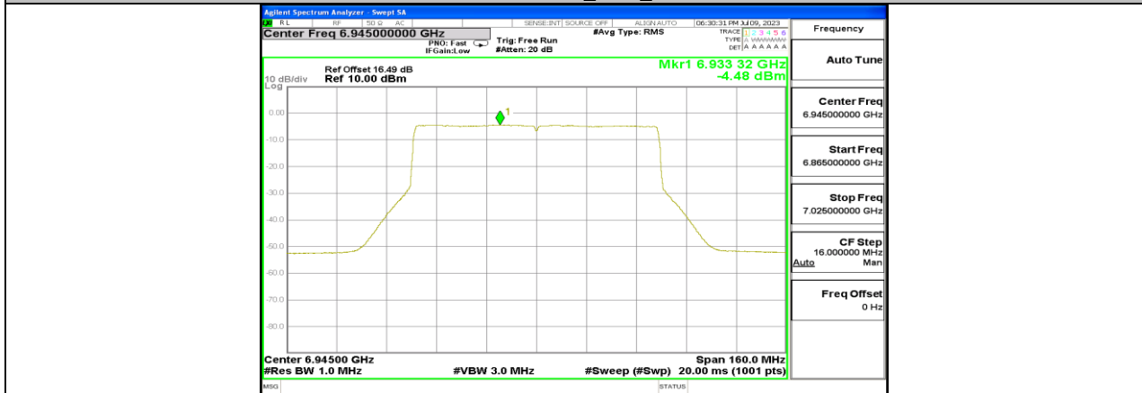
11AX80MIMO_Ant2_6945
