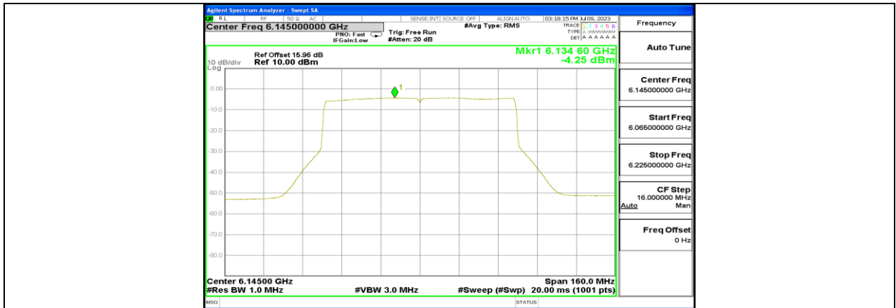
11AX80MIMO_Ant3_6145
