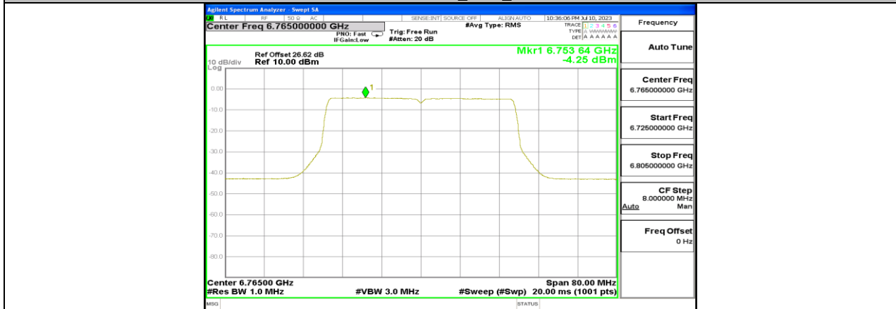
11BE40MIMO_Ant2_6765
