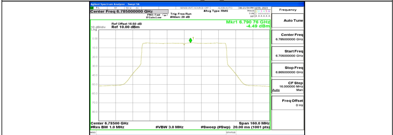
11AX80MIMO_Ant2_6785
