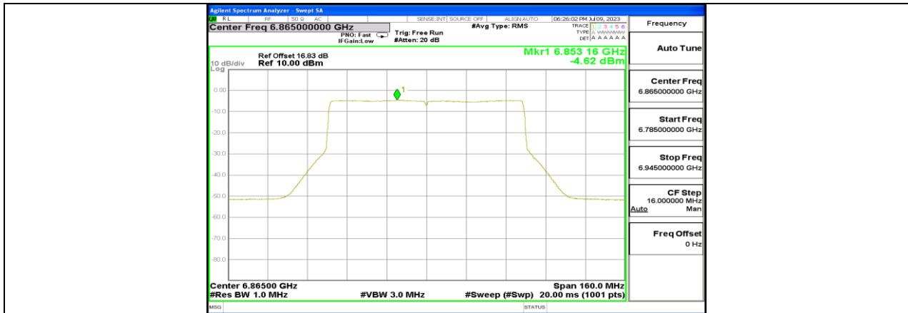
11AX80MIMO_Ant2_6865
