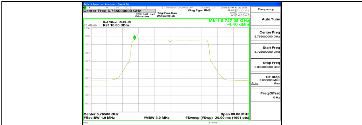
11AX40MIMO_Ant1_6765
