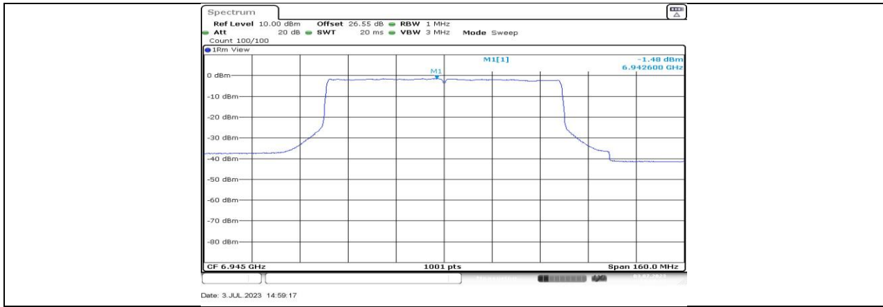
11BE80MIMO_Ant2_6945
