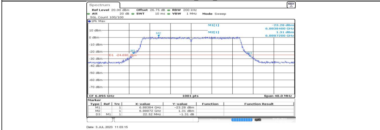
11AX20MIMO_Ant2_6895
