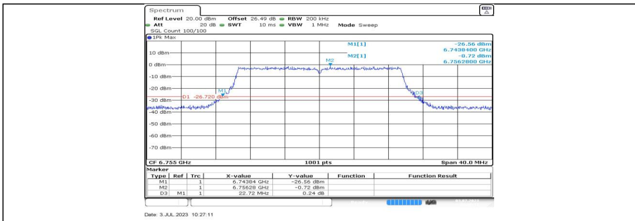
11AX20MIMO_Ant1_6755
