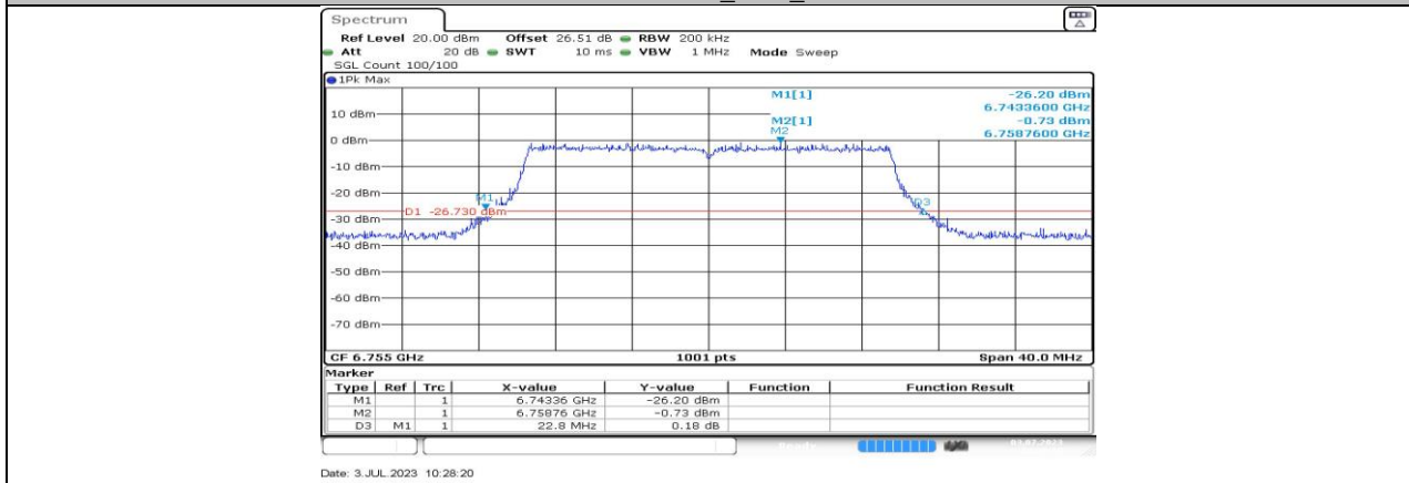
11AX20MIMO_Ant2_6755
