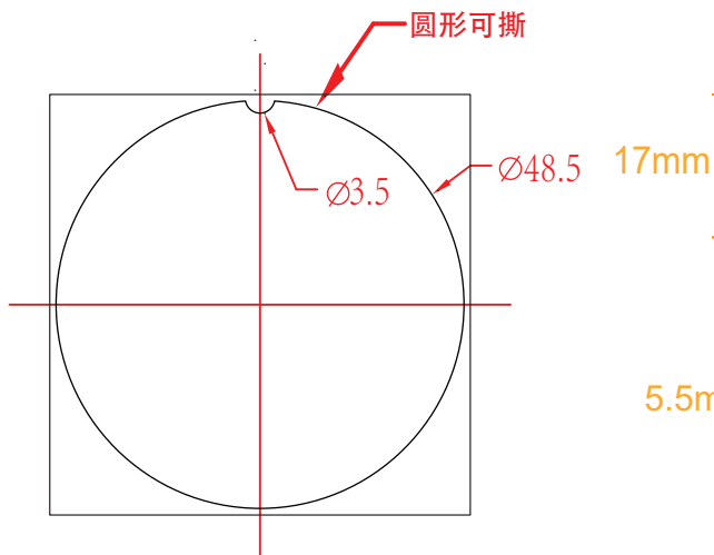
标贴尺寸图
