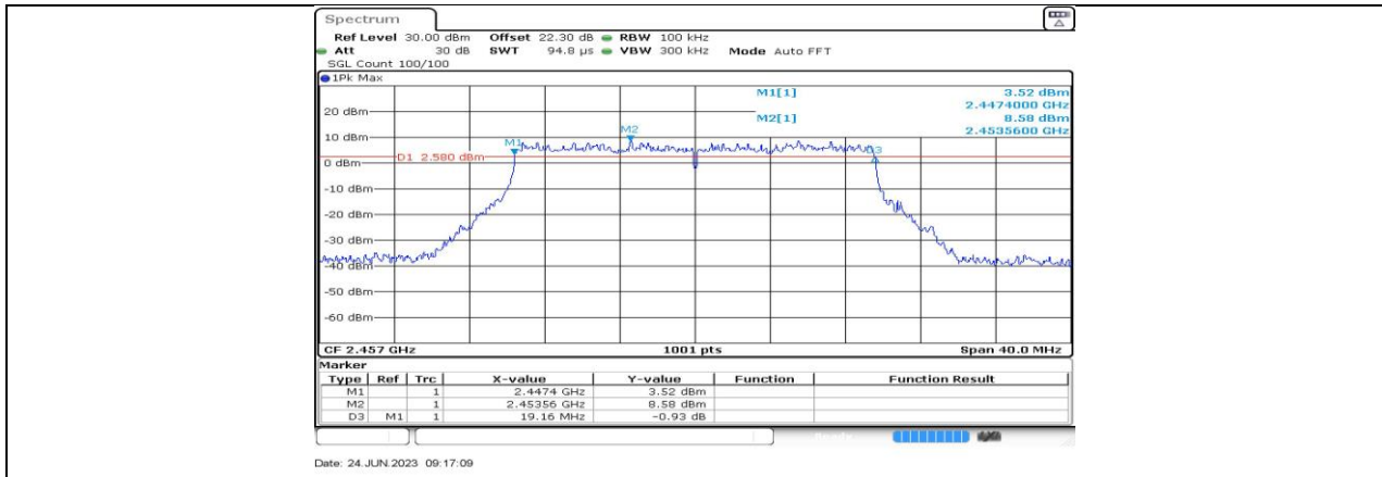
11AX20-CDD_Ant6_2457
