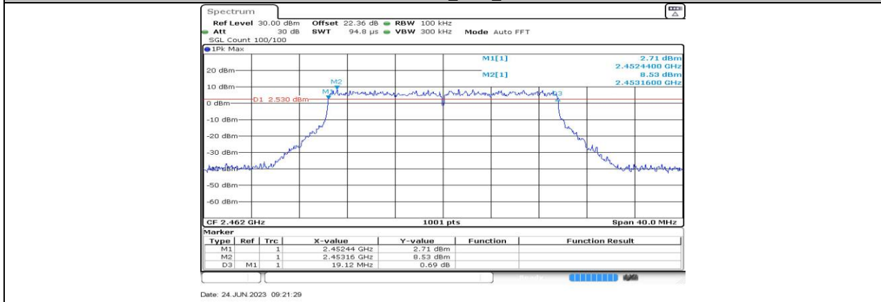
11AX20-CDD_Ant5_2462
