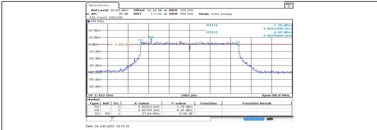
11AX40-CDD_Ant5_2422
