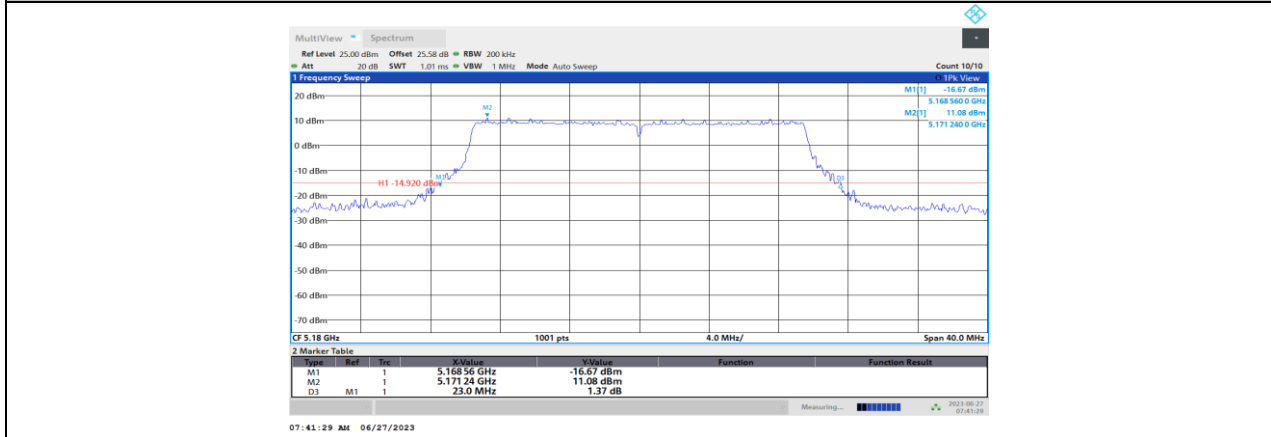
11BE20-CDD_Ant5_5180
