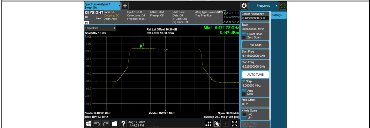
11BE40MIMO_Ant6_6485
