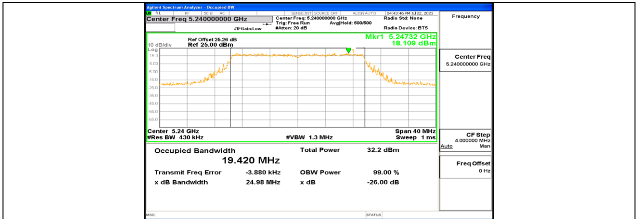
11BE20MIMO_Ant2_5240
