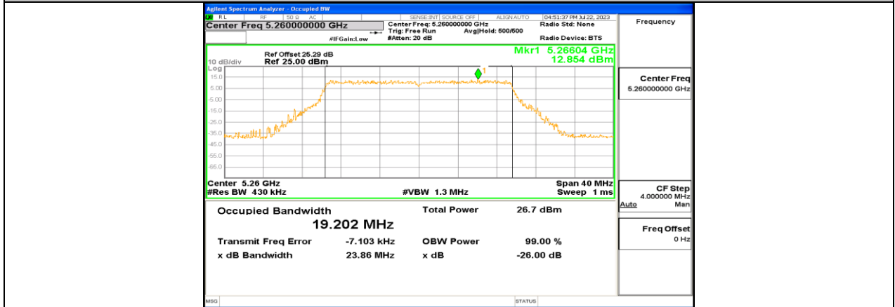
11BE20MIMO_Ant1_5260
