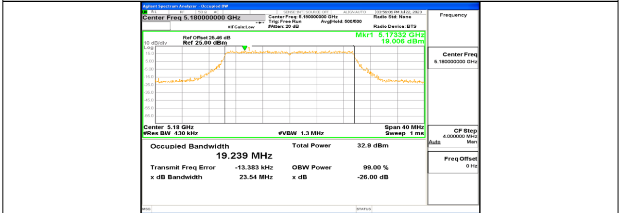
11BE20MIMO_Ant1_5180
