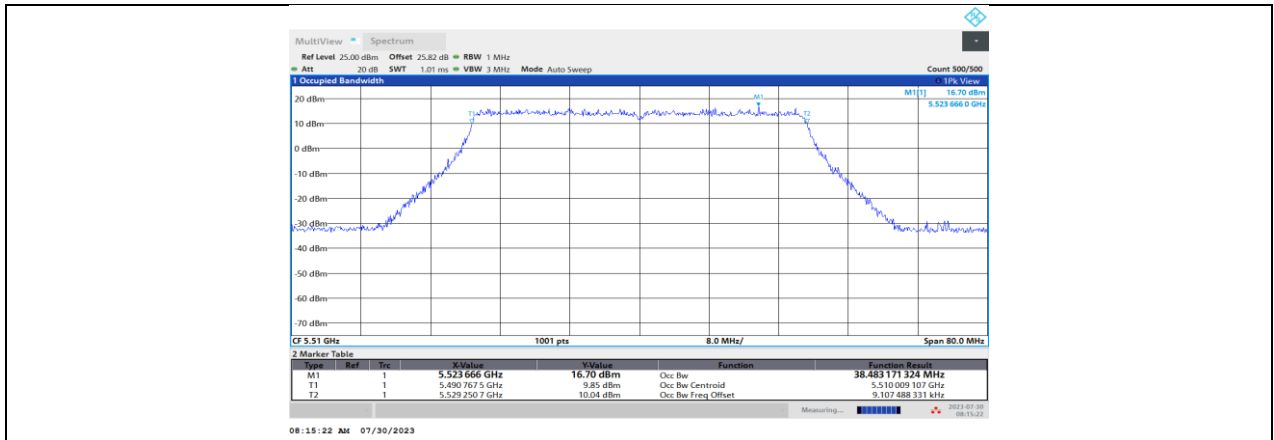
11BE40MIMO_Ant2_5510
