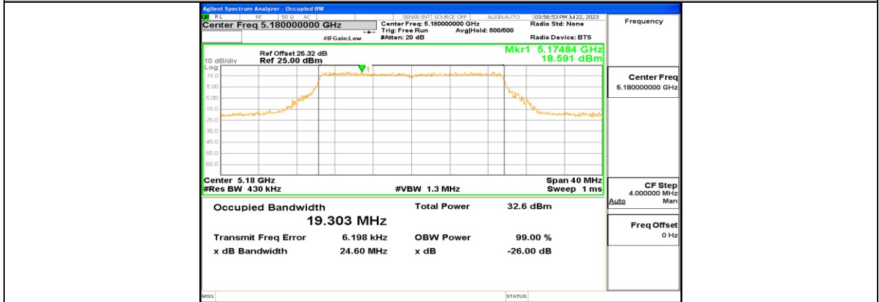
11BE20MIMO_Ant2_5180
