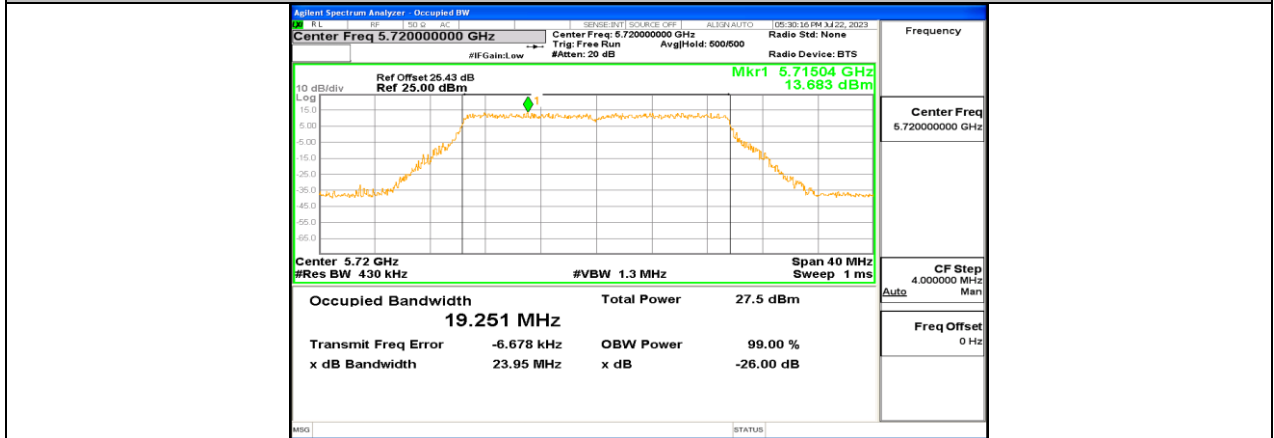
11BE20MIMO_Ant2_5720
