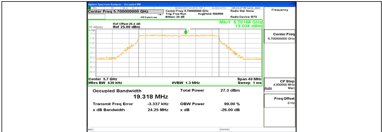
11BE20MIMO_Ant2_5700
