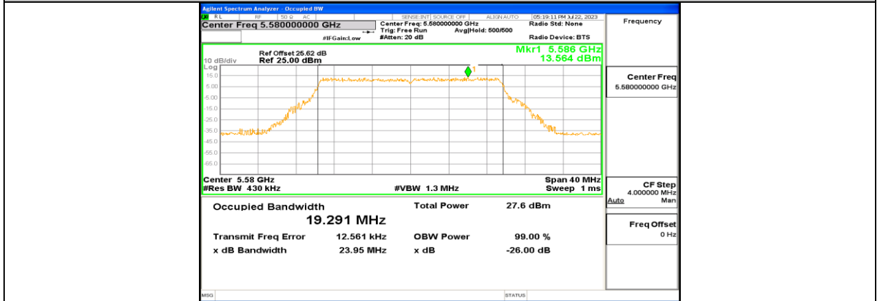
11BE20MIMO_Ant2_5580
