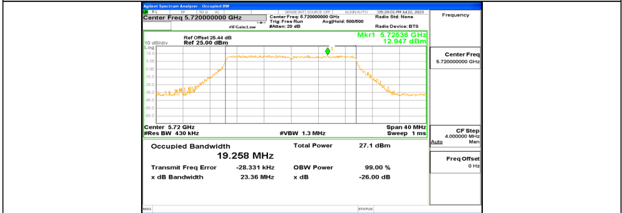
11BE20MIMO_Ant1_5720
