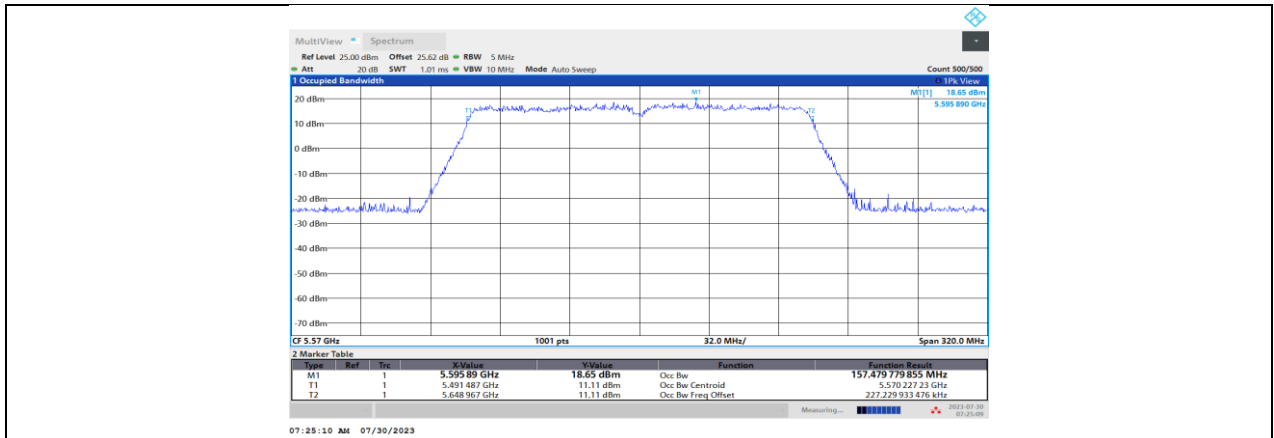
11AC160MIMO_Ant2_5570
