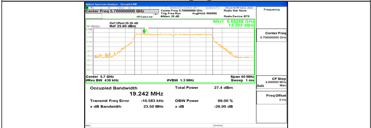
11BE20MIMO_Ant1_5700
