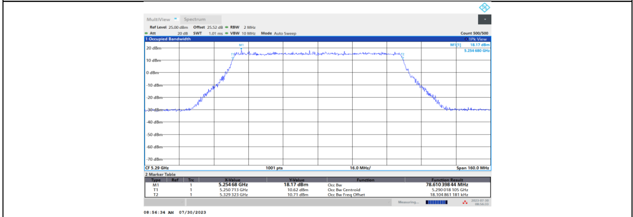
11BE80MIMO_Ant1_5290
