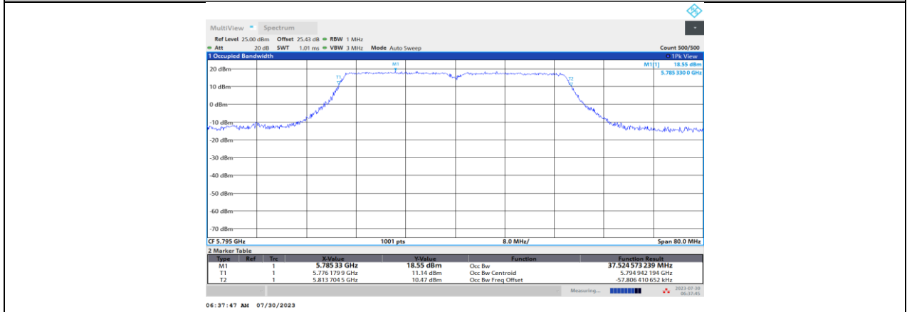
11AC40MIMO_Ant2_5795
