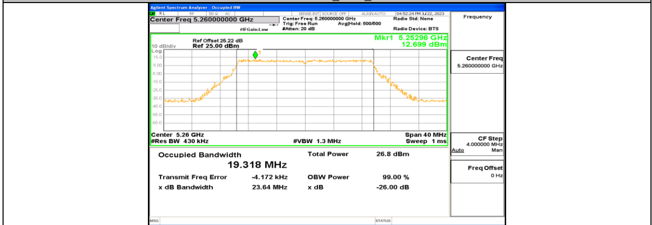
11BE20MIMO_Ant2_5260
